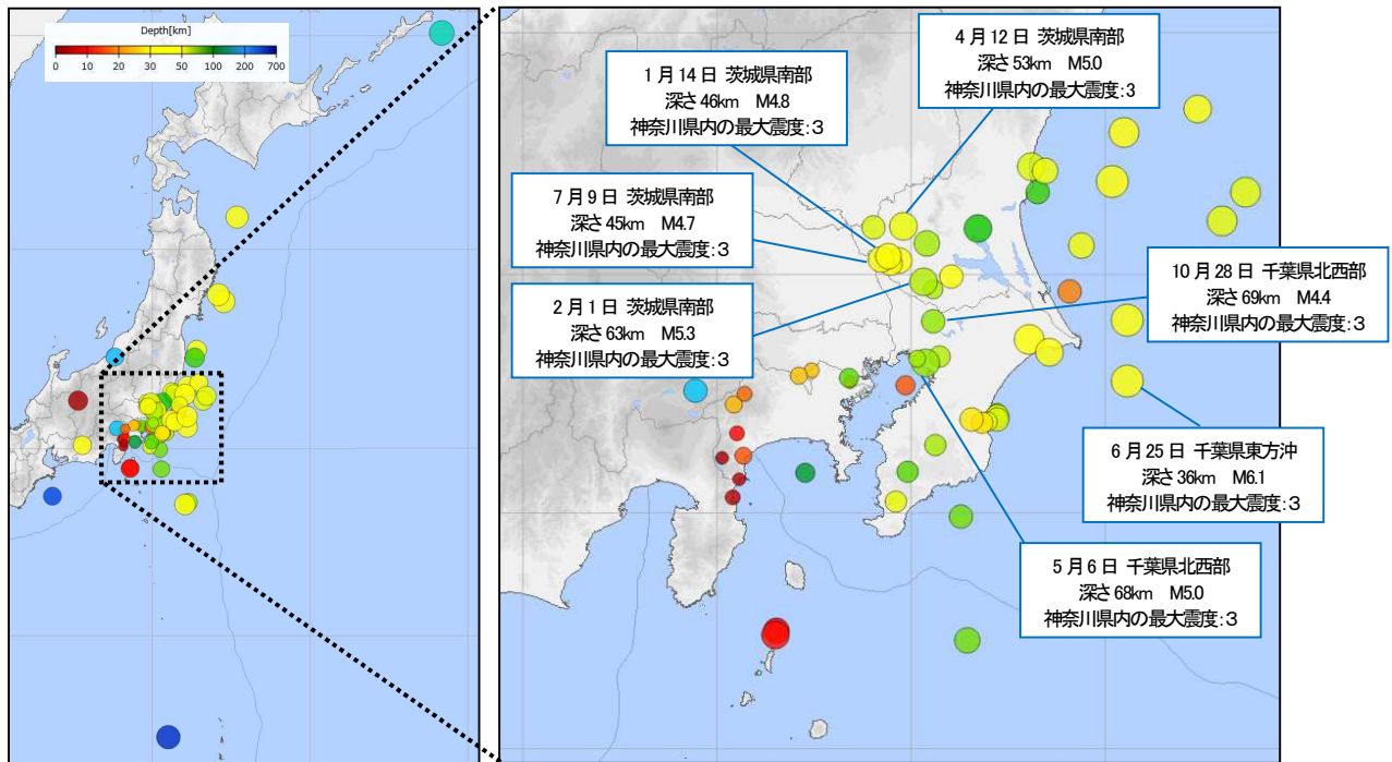
図1 神奈川県内で震度1以上を観測した地震の震央分布図(左:全体、右:神奈川県周辺拡大) ※神奈川県内で最大震度3以上を観測した地震に吹き出しをつけている。
