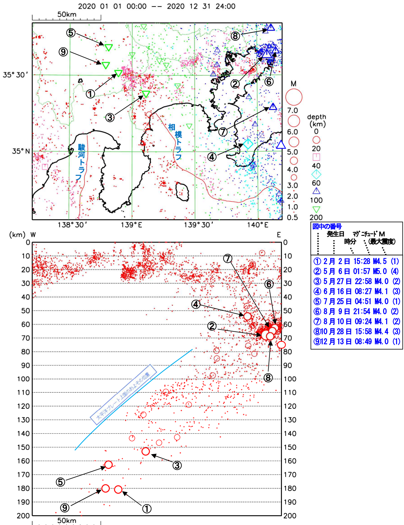
図2 神奈川県及び周辺域の震央分布図（上）と東西断面図（下）
