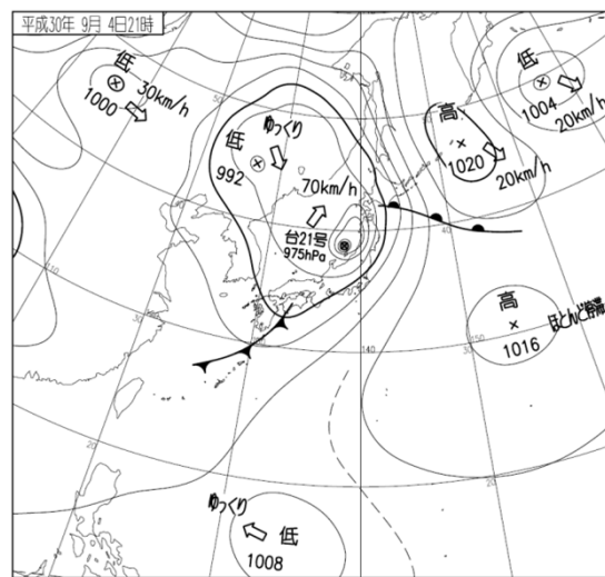
地上天気図
