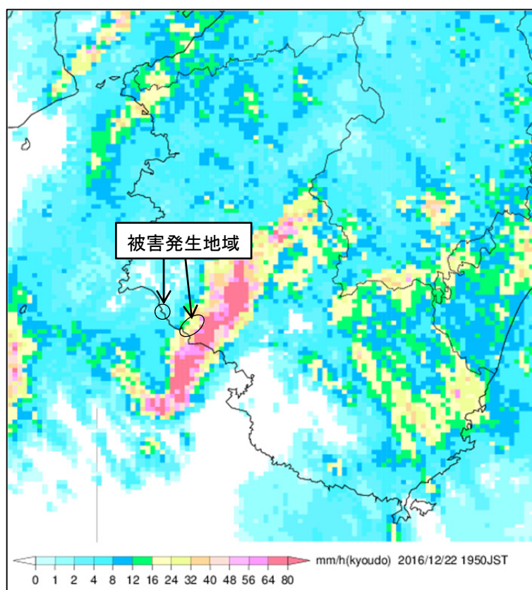
図10 気象レーダー画像（降水強度）（12月22日19時50分）
