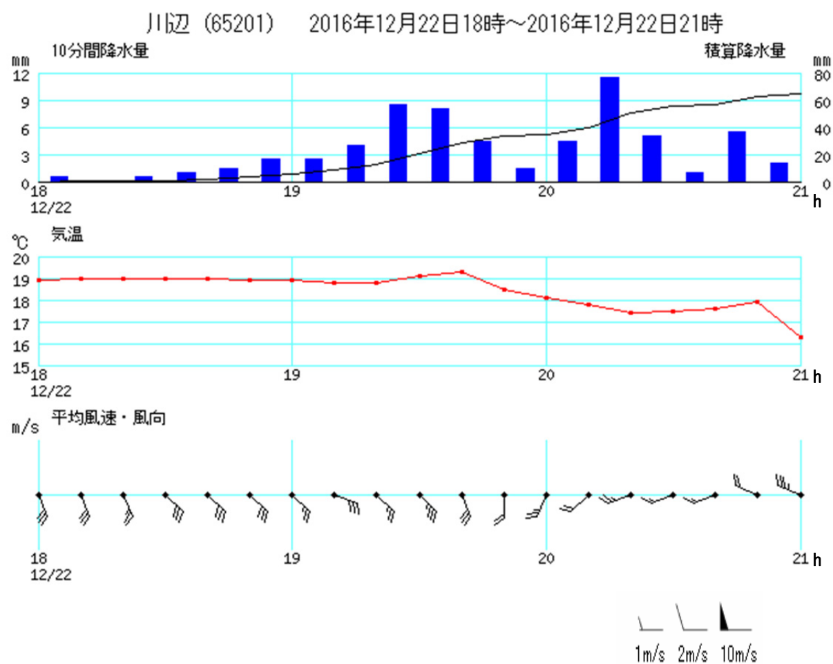
図 11 アメダス時系列グラフ (12 月 22 日 18 時 ～ 21 時)
