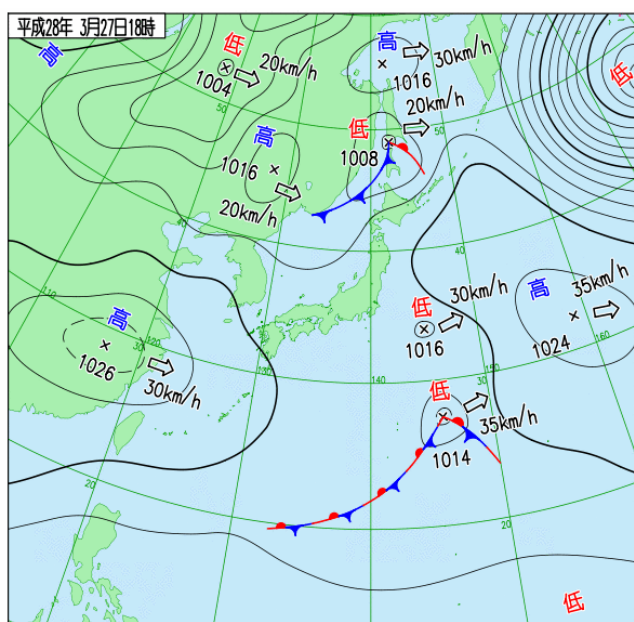
3月27日18時の地上天気図（左）と気象衛星赤外画像（右）
