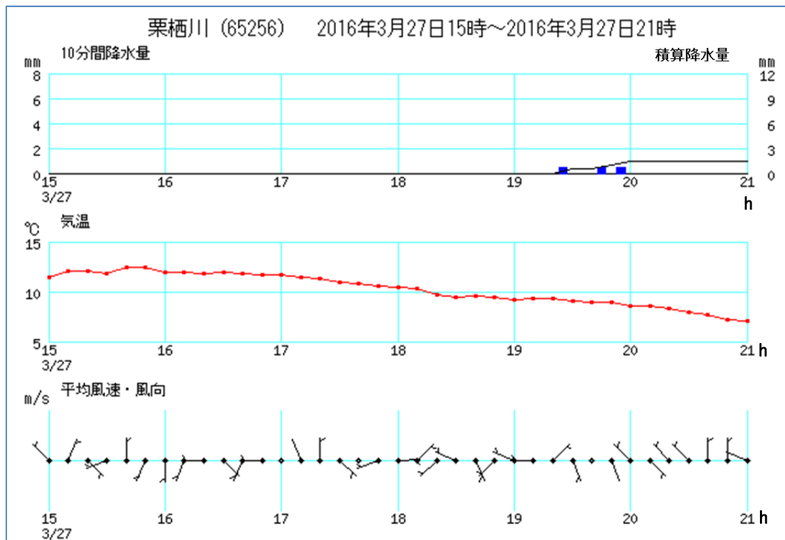
(5) 被害発生地域近傍のアメダス観測所 10 分値データ時系列図 (27 日 15 時～21 時)
