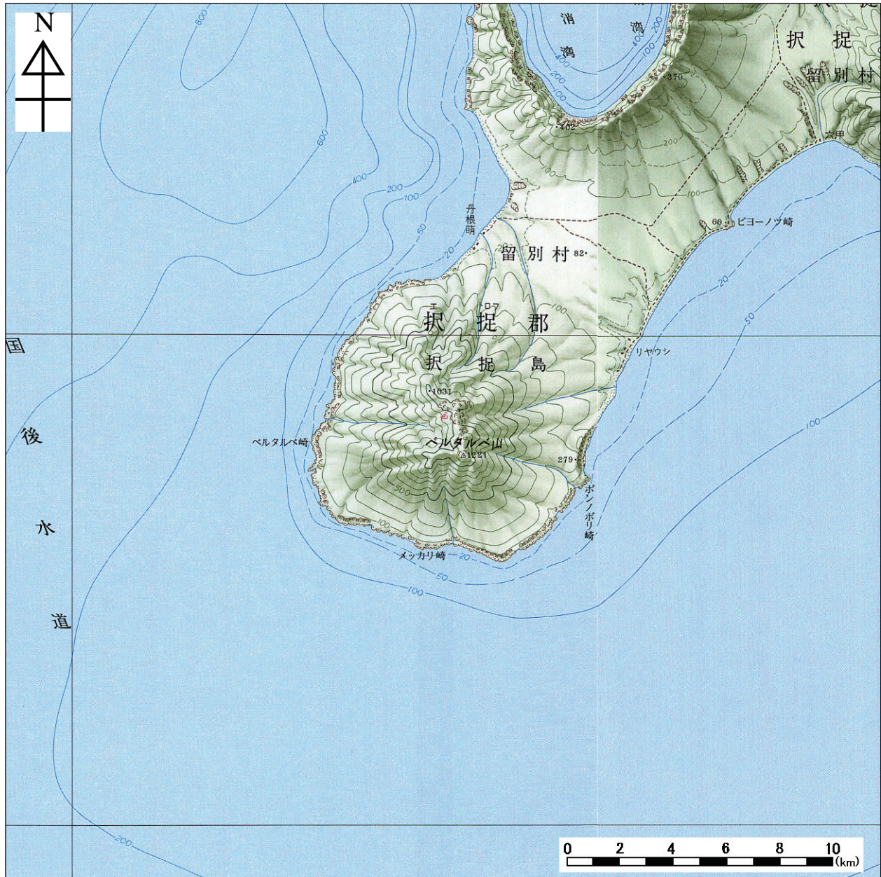
図 106-1 ベルタルベ山の地勢 国土地理院発行の 20 万分の 1 地勢図(安渡移矢岬、得茂別湖)
