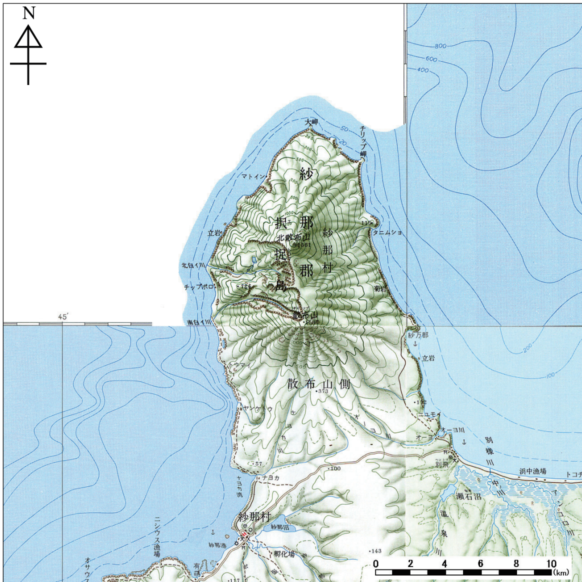
図 101-1 散布山の地勢 国土地理院発行の 20 万分の 1 地勢図(紗那、別飛、薬取)
