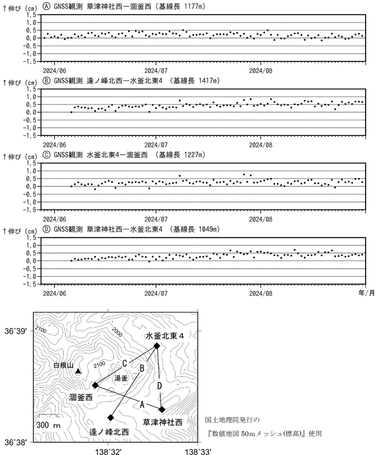
図6－1 草津白根山 湯釜近傍での臨時のGNSS連続観測結果（2024年5月29日～2024年8月31日） 下図の◆（水釜北東4、涸釜西、草津神社西及び逢ノ峰北西）は、臨時に設置したGNSS連続観測点を示します。 上図の①～④は下図のA～Dと対応しています。
