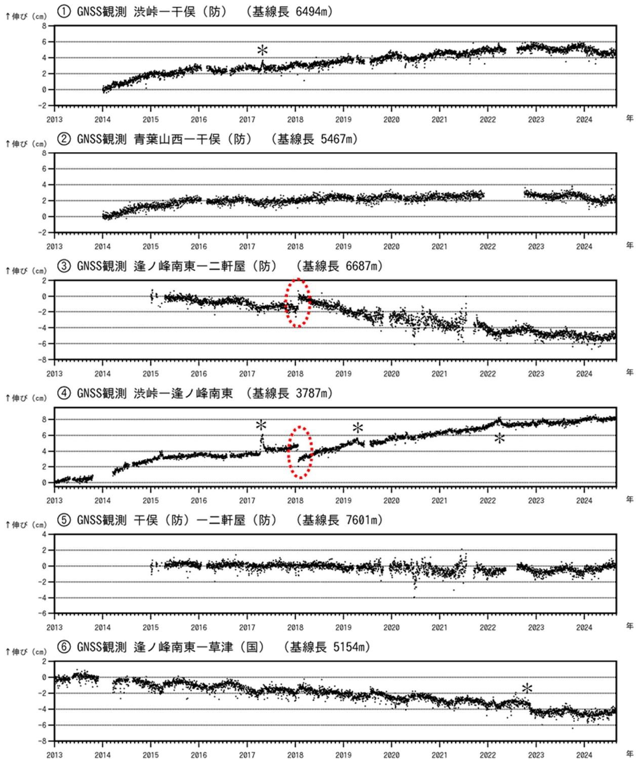
図6-2 草津白根山 GNSS 連続観測の結果（2013年1月1日～2024年8月31日）
