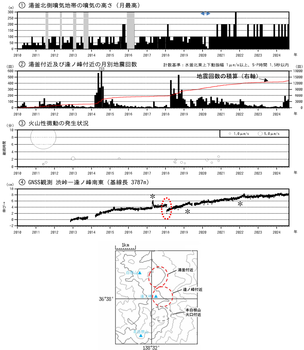
図3 草津白根山（白根山（湯釜付近）） 火山活動経過図（2010年1月1日～2024年8月31日）
