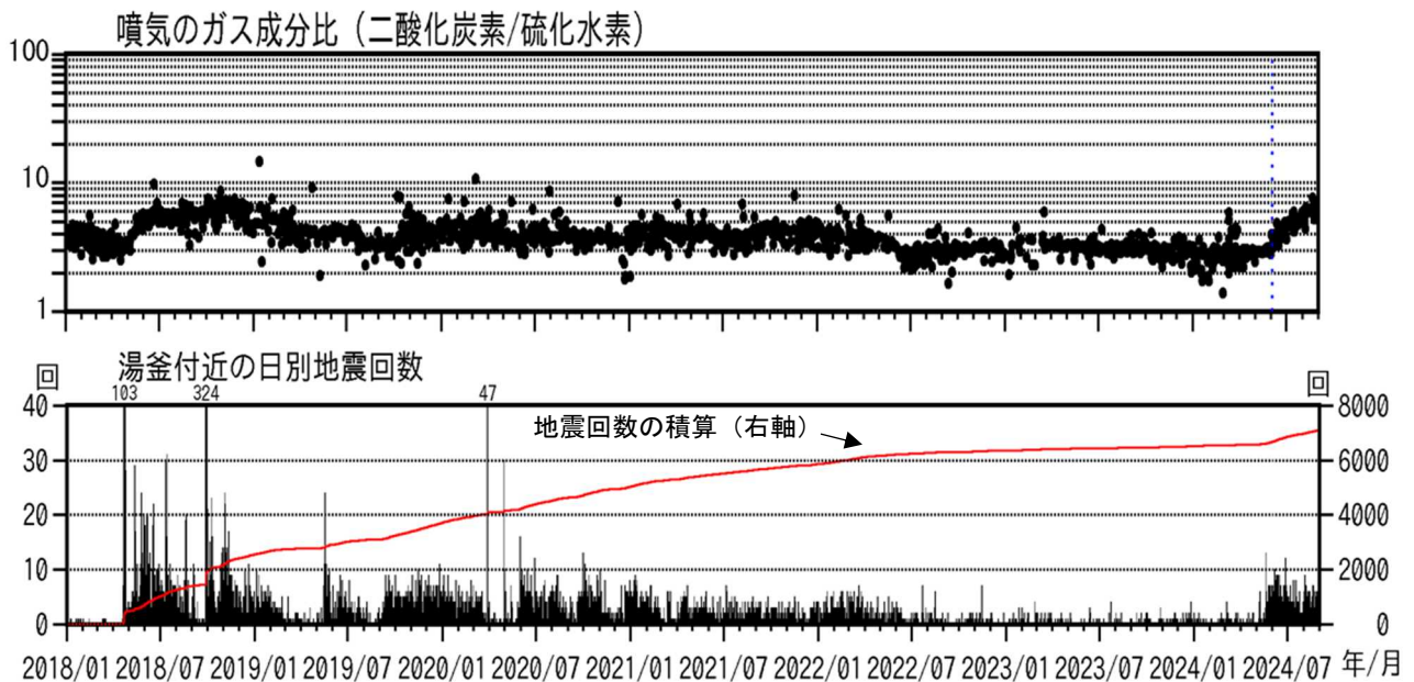
図8 草津白根山（白根山（湯釜付近）） 火山ガス観測結果（2018年1月～2024年8月）
