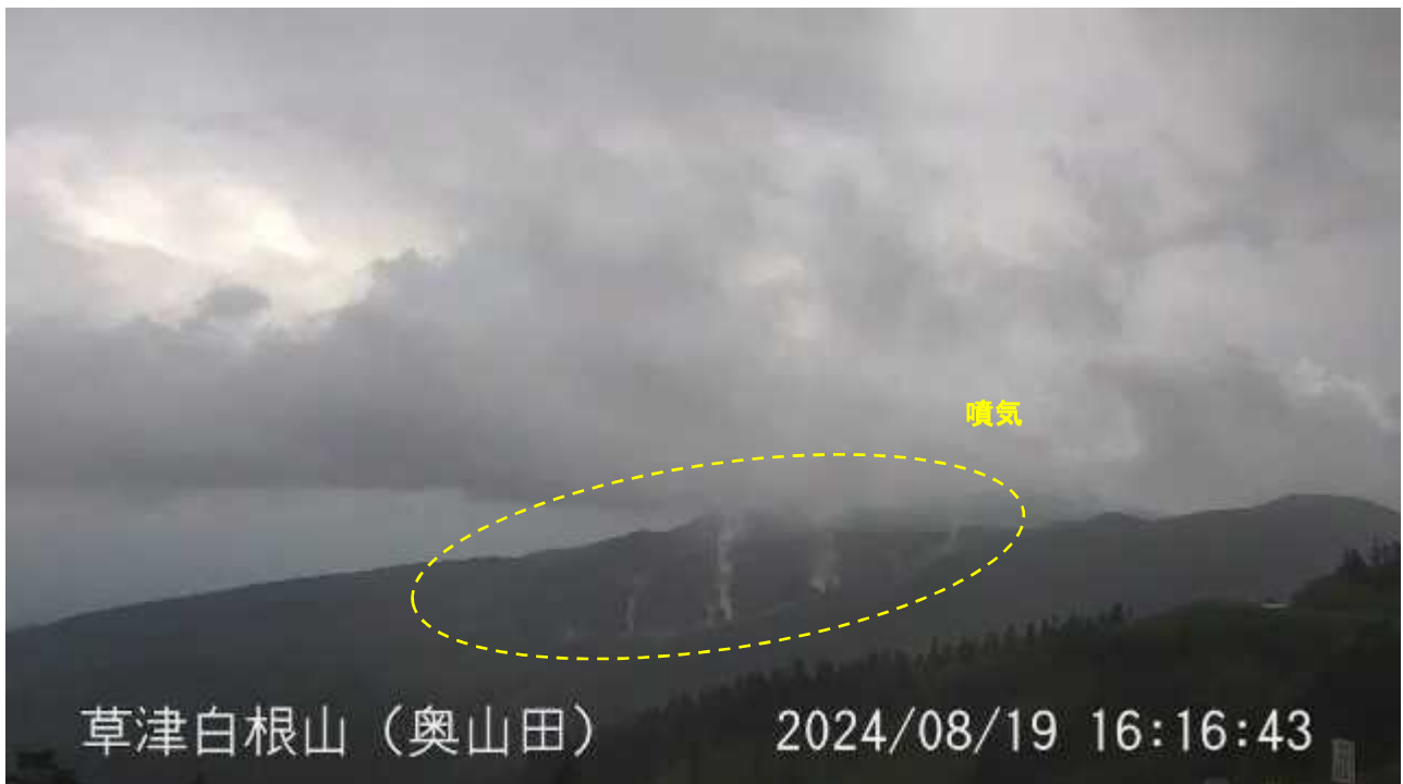
図 2 草津白根山（白根山（湯釜付近））奥山田監視カメラによる湯釜付近の状況（8月19日） ・湯釜火口北側噴気地帯の噴気は 200m 以下で推移し、特段の変化は認められませんでした。
