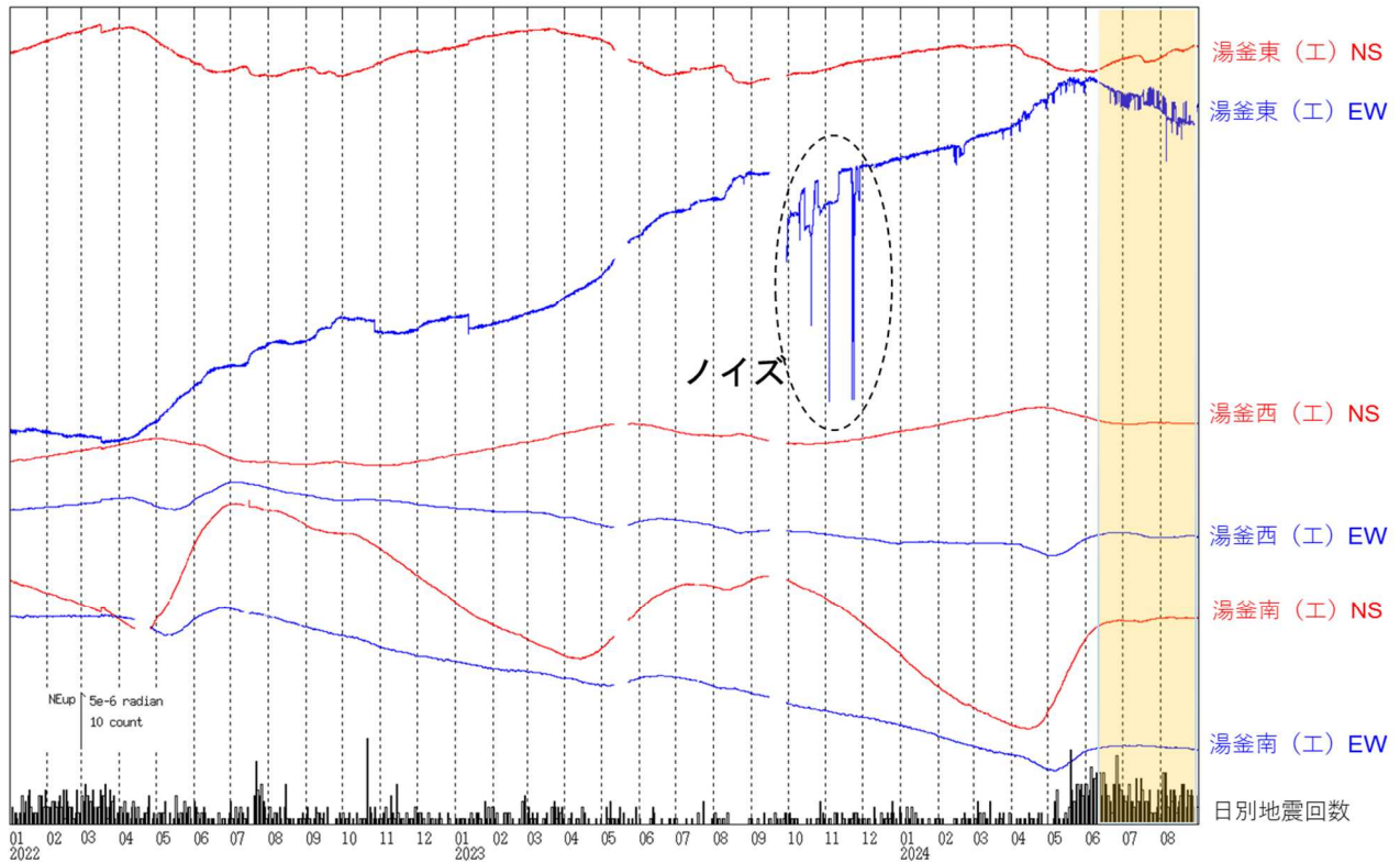
図5 草津白根山（白根山（湯釜付近）） 傾斜変動（2022年1月1日～2024年8月31日）
