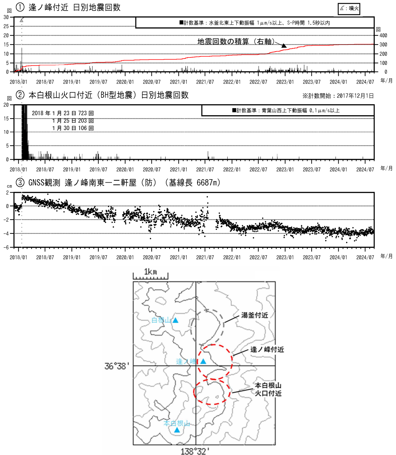
図13 草津白根山（本白根山） 火山活動経過図（2017年12月1日～2024年8月31日）
