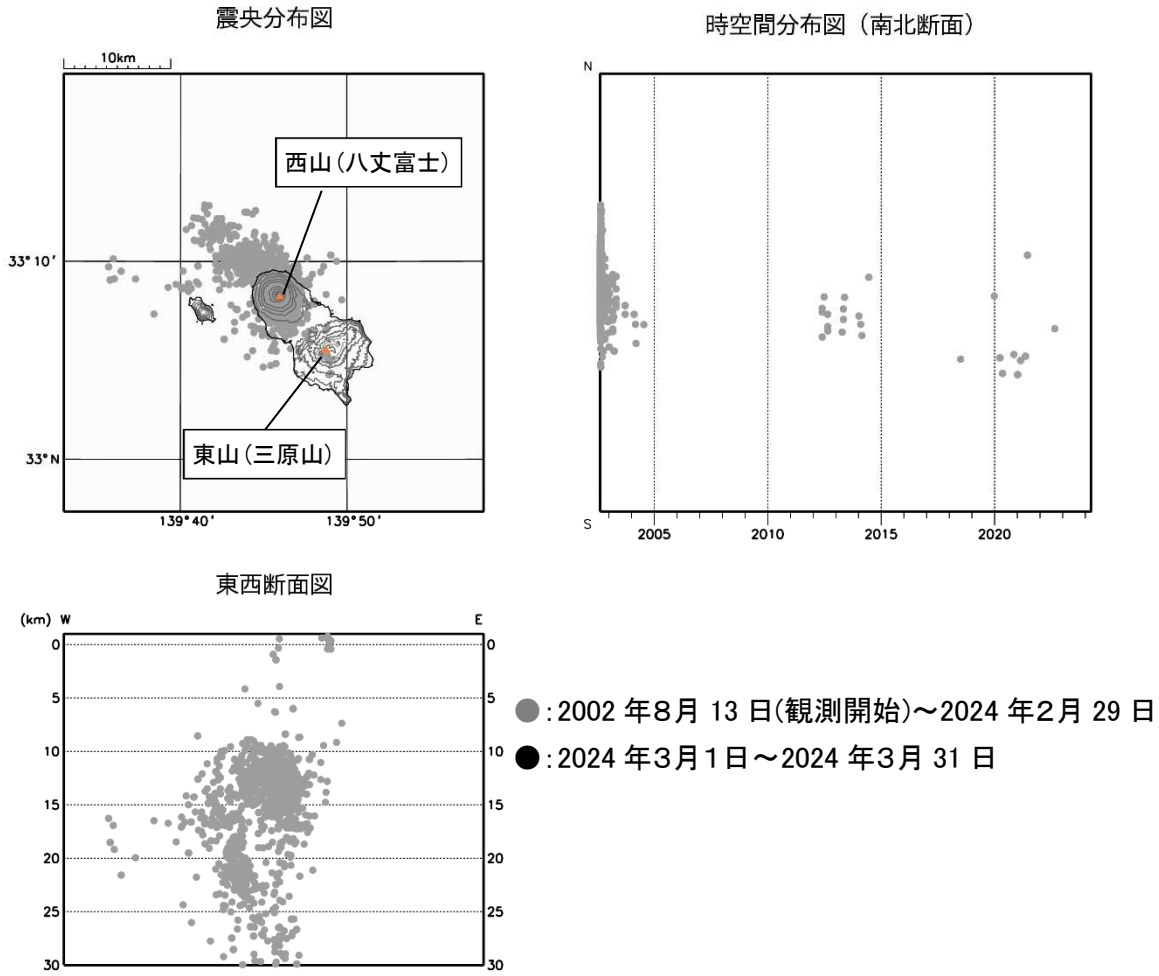
図3 八丈島 震源分布図（2002年8月13日～2024年3月31日）
