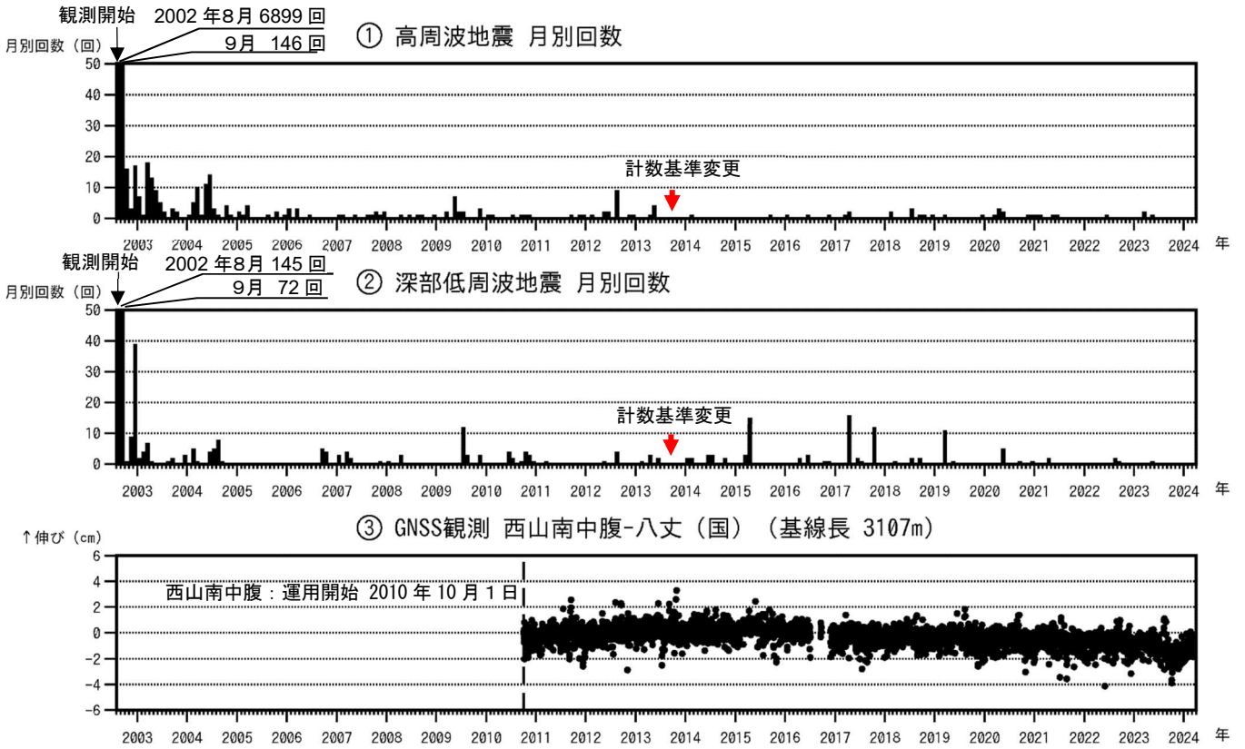
図2 八丈島 火山活動経過図（2002年8月13日～2024年3月31日）
