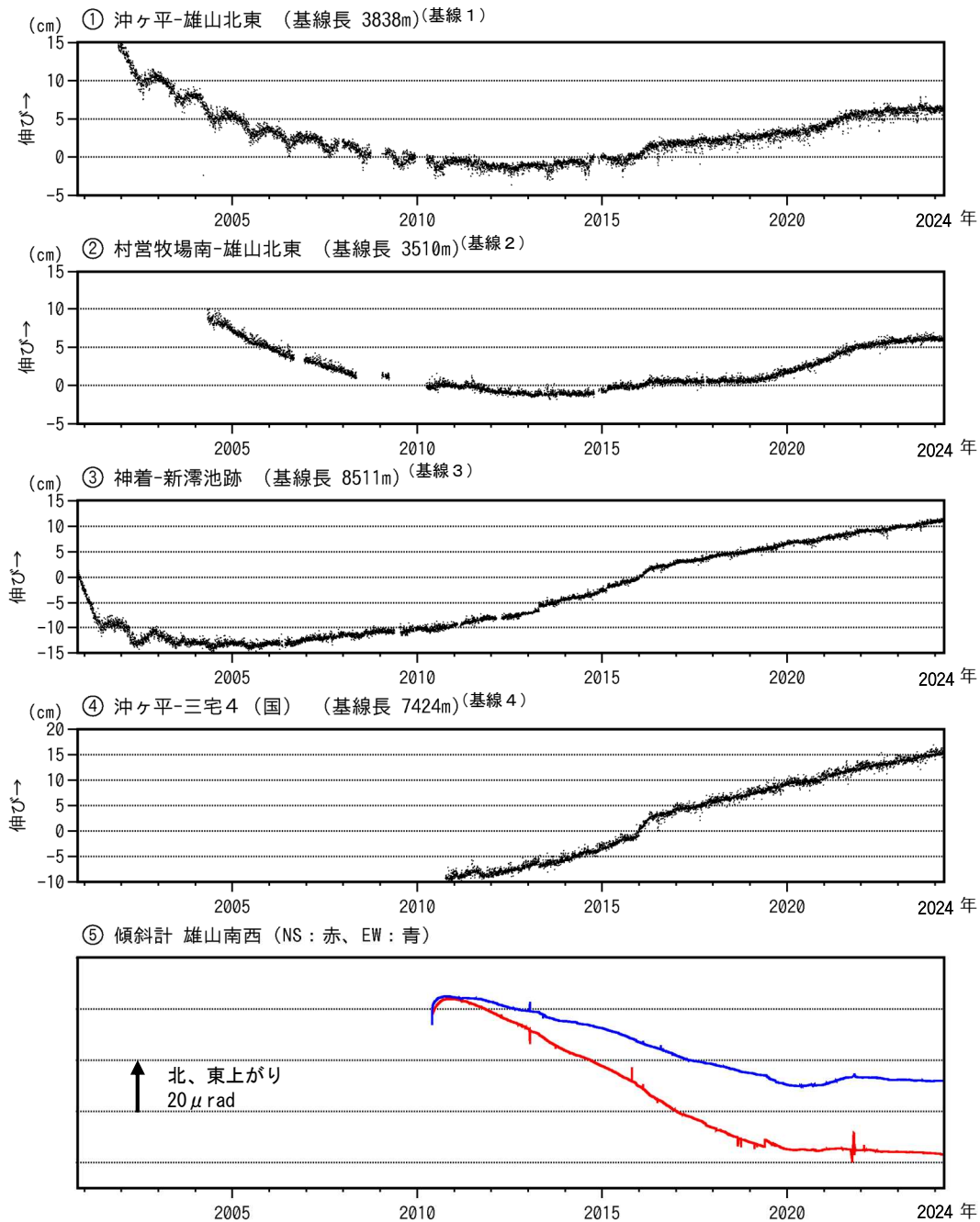
図8 三宅島 GNSS 連続観測及び傾斜計観測結果（2000年10月26日～2024年3月31日）
