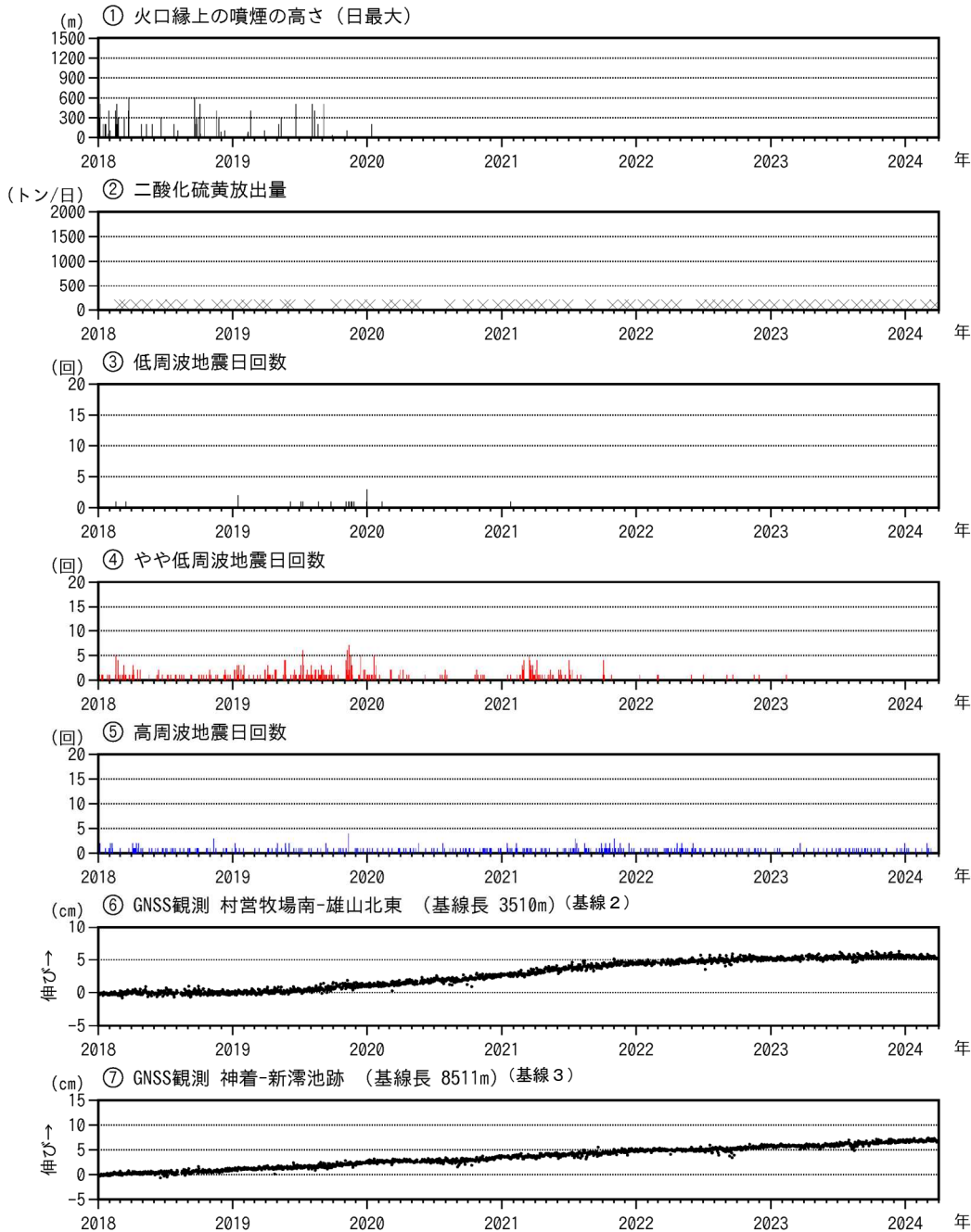
図6 三宅島 火山活動経過図（2018年1月1日～2024年3月31日）
