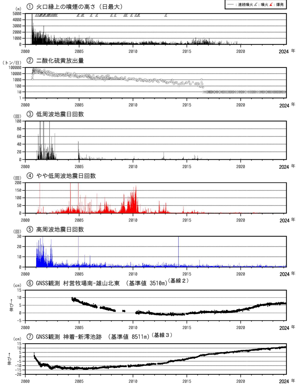
図7 三宅島 長期の火山活動経過図（2000年1月1日～2024年3月31日）
