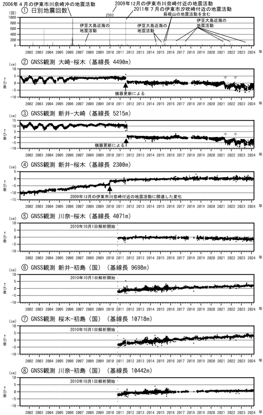
図3 伊豆東部火山群 火山活動経過図（2001年2月1日～2024年3月31日）
