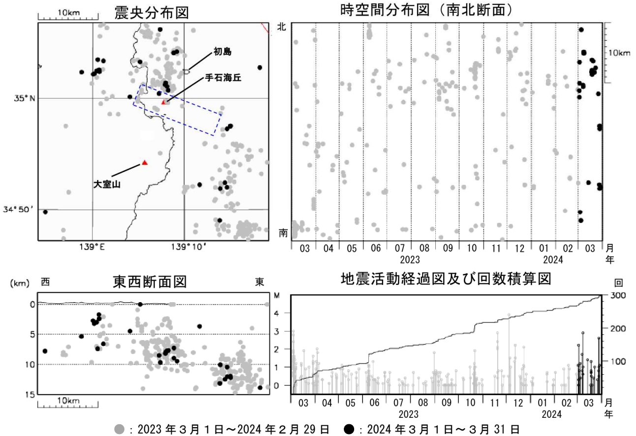
図2 伊豆東部火山群 広域地震観測網による震源分布図（2023年3月1日～2024年3月31日） □の領域は群発地震活動の発生する可能性がある範囲（火口が出現する可能性のある範囲）を示しています。 https://www.data.jma.go.jp/vois/data/tokyo/STOCK/level/PDF/level_316.pdf 広域地震観測網により震源決定したもので、深さは全て海面以下として決定しています。 M（マグニチュード）は地震の規模を表し、M0.0以上を表示しています。 図中の震源要素は一部暫定値が含まれており、後日変更することがあります。 この図では、関係機関の地震波形を一元的に処理し、地震観測点の標高を考慮する等した手法で得られた震源を用いています。
