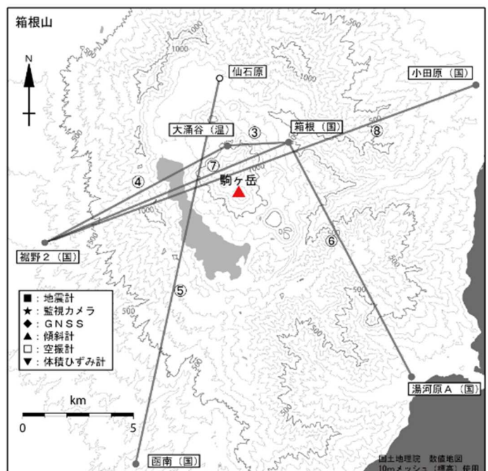
図3-2 箱根山 GNSS 連続観測による基線長変化及び観測点配置図 (2012年1月1日~2024年3月31日) (国): 国土地理院 (温): 神奈川県温泉地学研究所 空白部分は欠測を示します。
