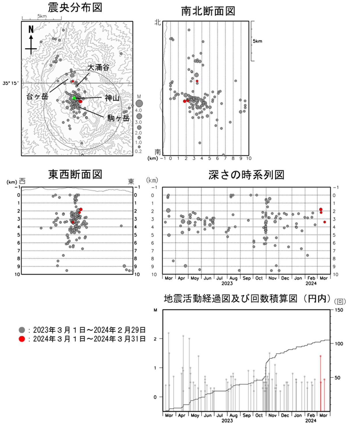
図4 箱根山 広域地震観測網による山体周辺の震源分布図（2023年3月1日～2024年3月31日）
