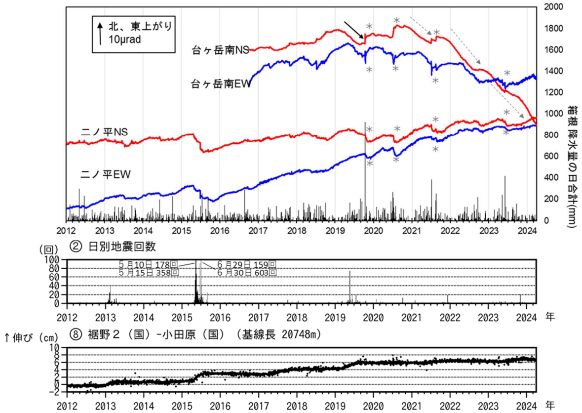
図5 箱根山 傾斜観測及び地震回数・GNSS観測（2012年1月1日～2024年3月31日）
