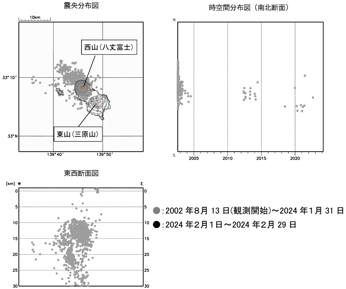
図3 八丈島 震源分布図（2002年8月13日～2024年2月29日）
