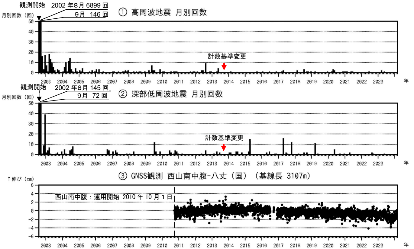
図2 八丈島 火山活動経過図（2002年8月13日～2024年2月29日）
