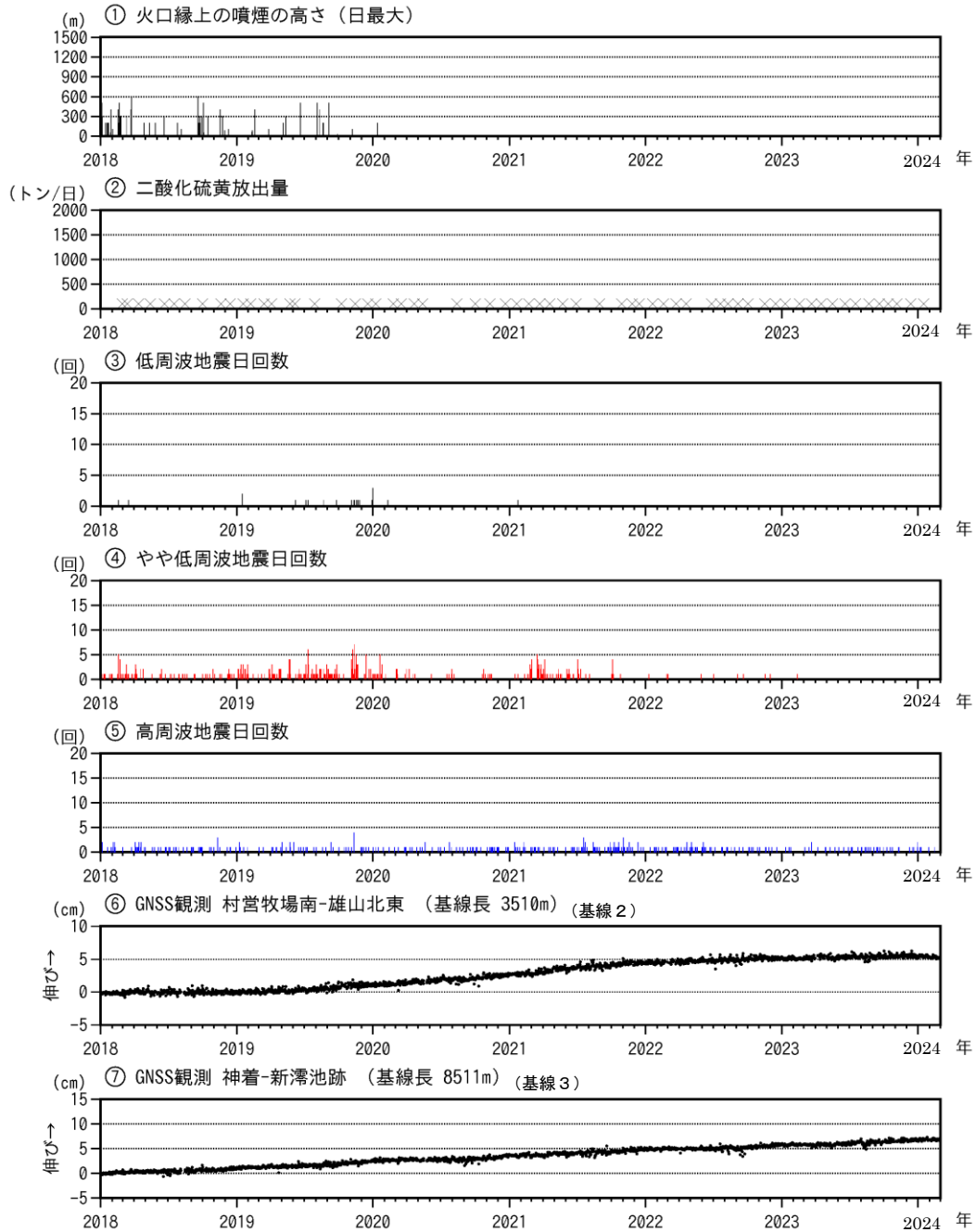
図7 三宅島 火山活動経過図（2018年1月1日～2024年2月29日）
