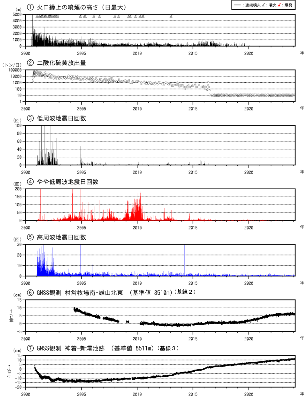
図8 三宅島 長期の火山活動経過図（2000年1月1日～2024年2月29日）
