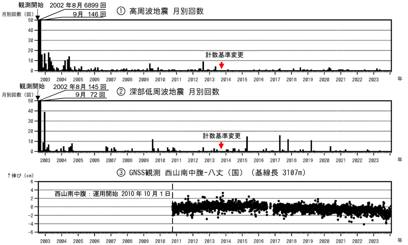
図2 八丈島 火山活動経過図（2002年8月13日～2024年1月31日）
