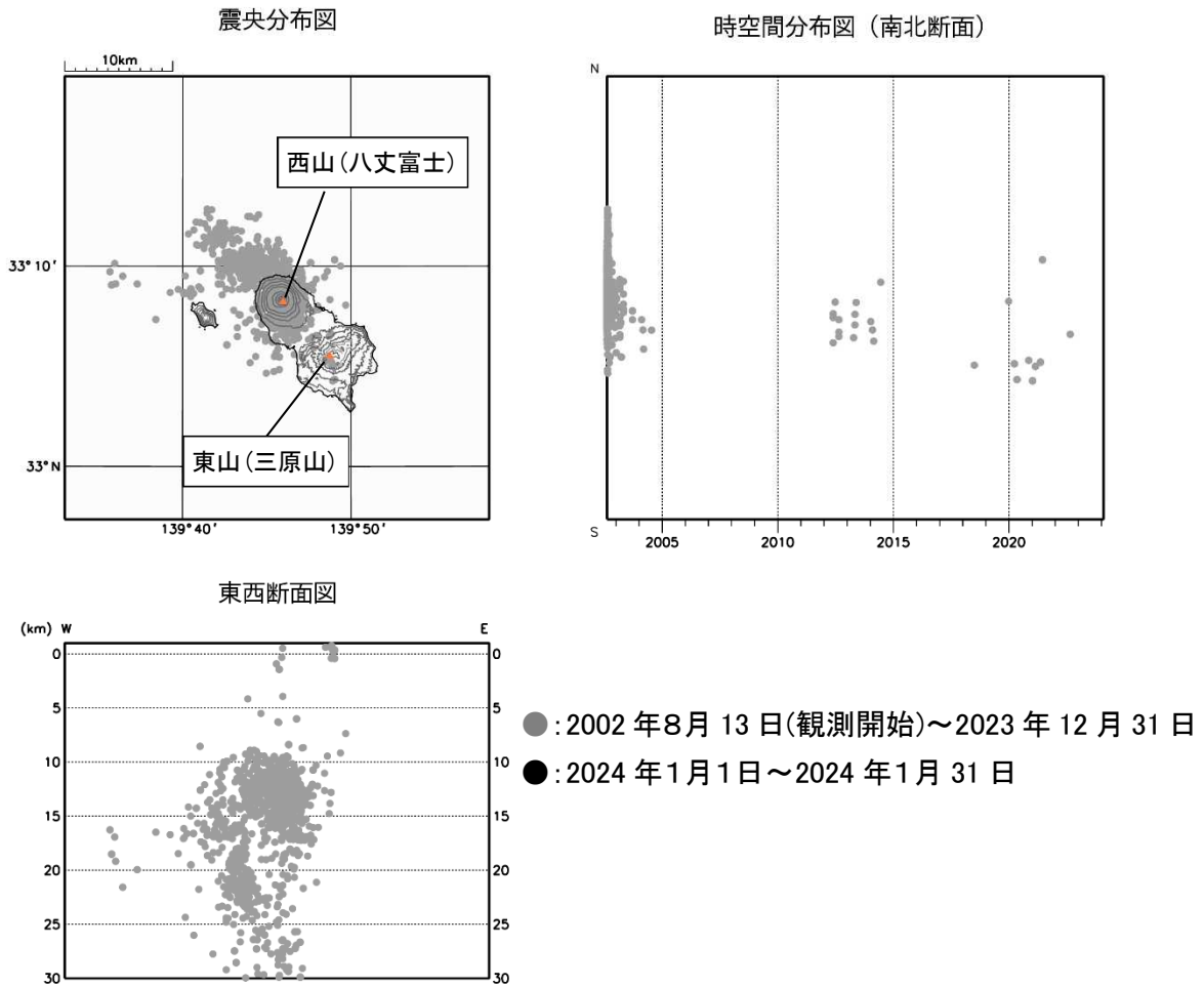
図3 八丈島 震源分布図（2002年8月13日～2024年1月31日）
