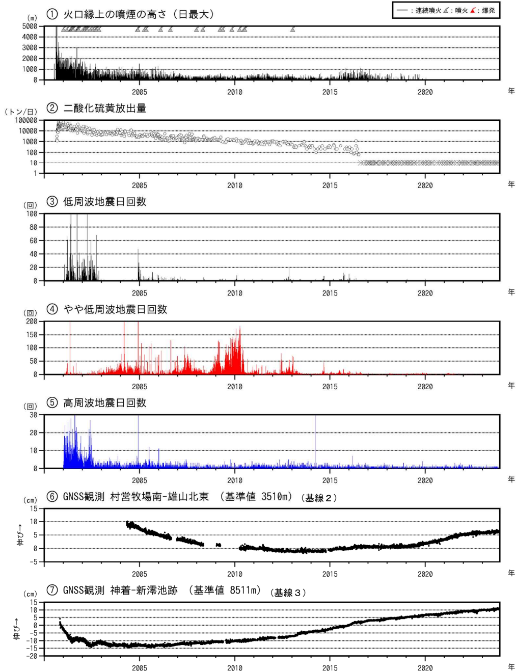
図7 三宅島 長期の火山活動経過図（2000年1月1日～2023年11月30日）
