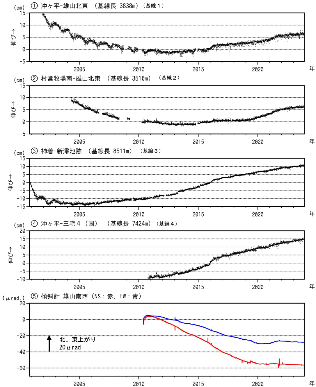
図 8 三宅島 GNSS 連続観測及び傾斜計観測結果（2000 年 10 月 26 日～2023 年 11 月 30 日）
