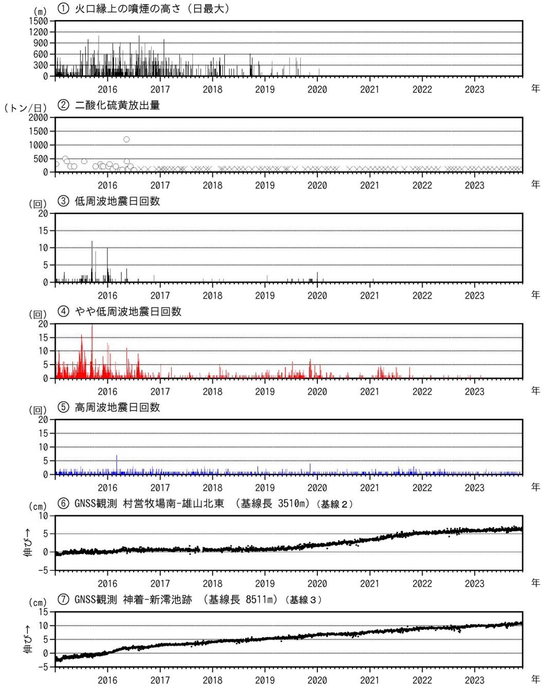
図6 三宅島 火山活動経過図（2015年1月1日～2023年11月30日）
