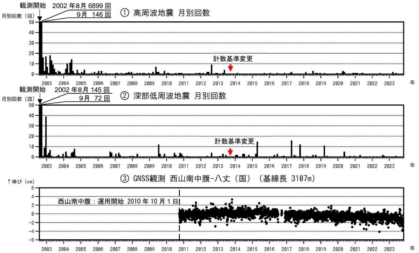
図2 八丈島 火山活動経過図（2002年8月13日～2023年10月31日）
