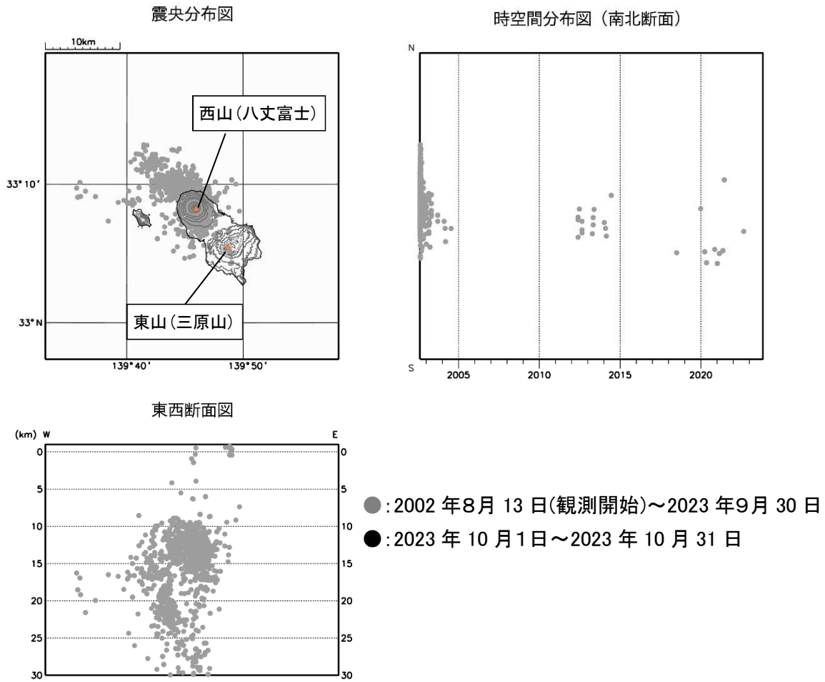
図3 八丈島 震源分布図（2002年8月13日～2023年10月31日）
