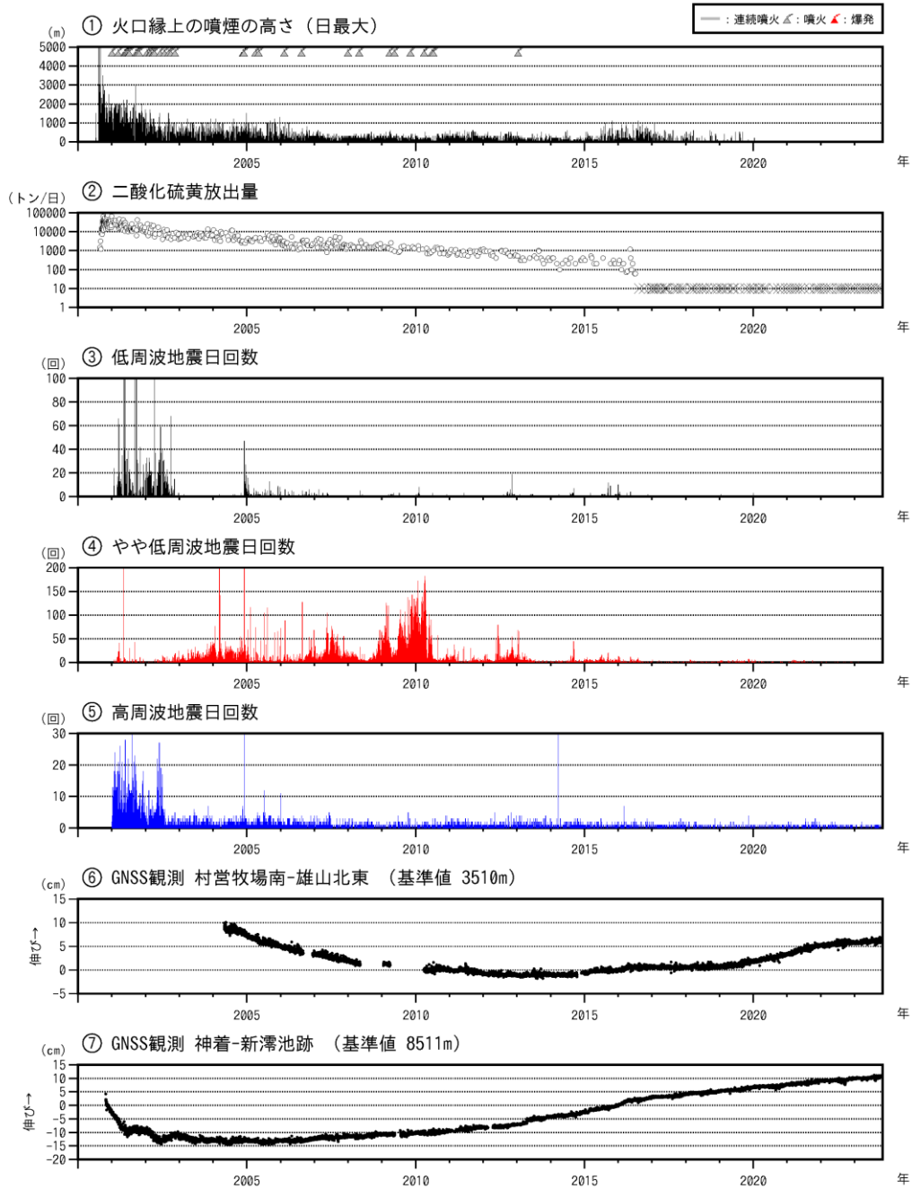
図7 三宅島 長期の火山活動経過図（2000年1月1日～2023年10月31日）
