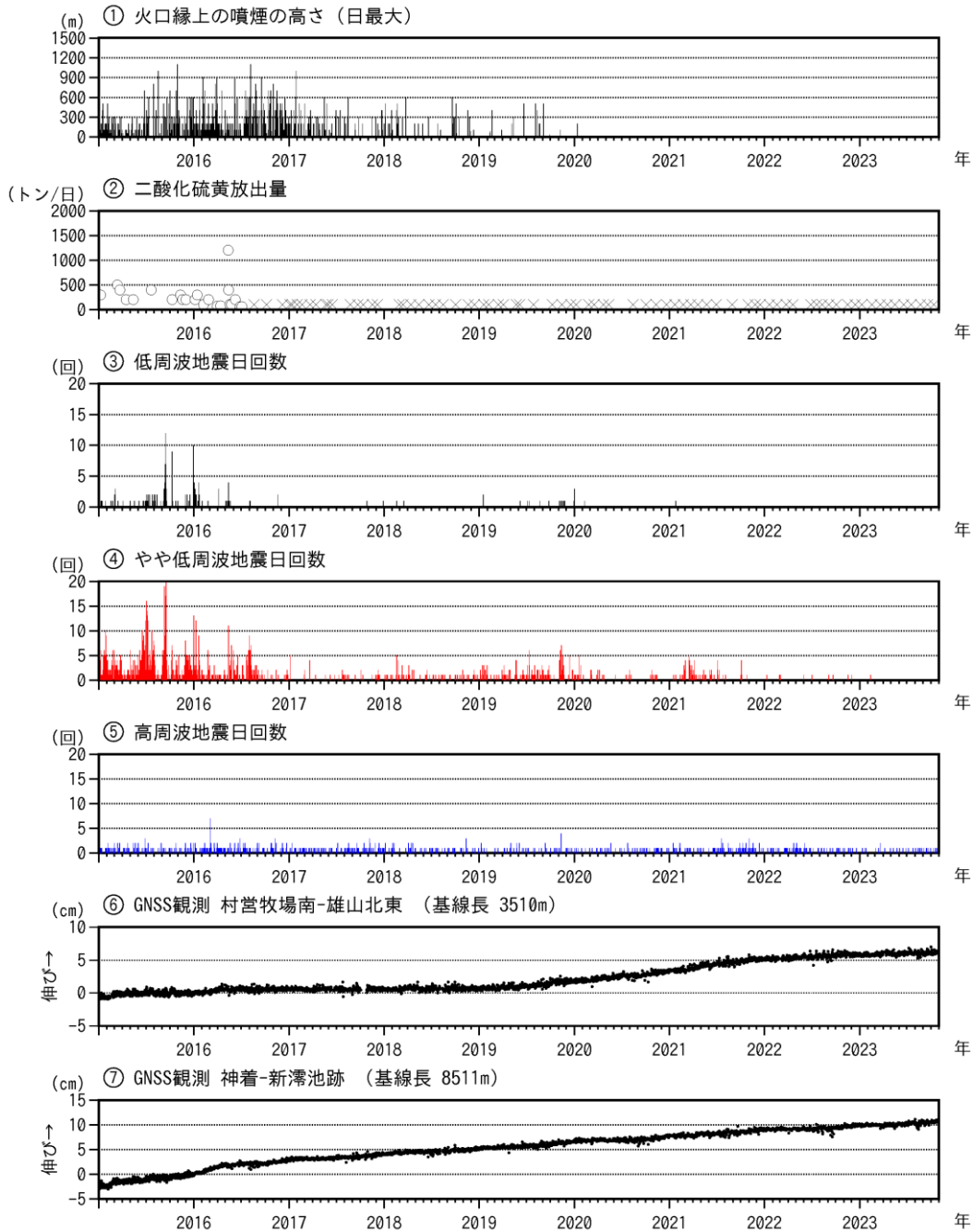
図6 三宅島 火山活動経過図（2015年1月1日～2023年10月31日）
