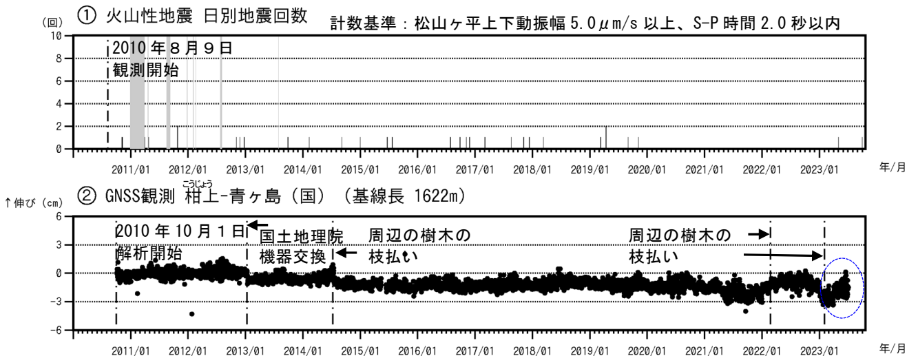
図3 青ヶ島 火山活動経過図（2010年8月9日～2023年9月30日） ① グラフの灰色部分は機器障害による欠測を示す。 ② (国)：国土地理院、図4のGNSS基線②に対応。グラフの空白部分は欠測を示す。 ・青破線で囲んだ変化は原因不明の変化ですが、火山活動によるものではないと考えています。
