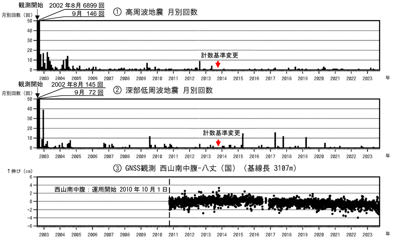
図2 八丈島 火山活動経過図（2002年8月13日～2023年9月30日）
