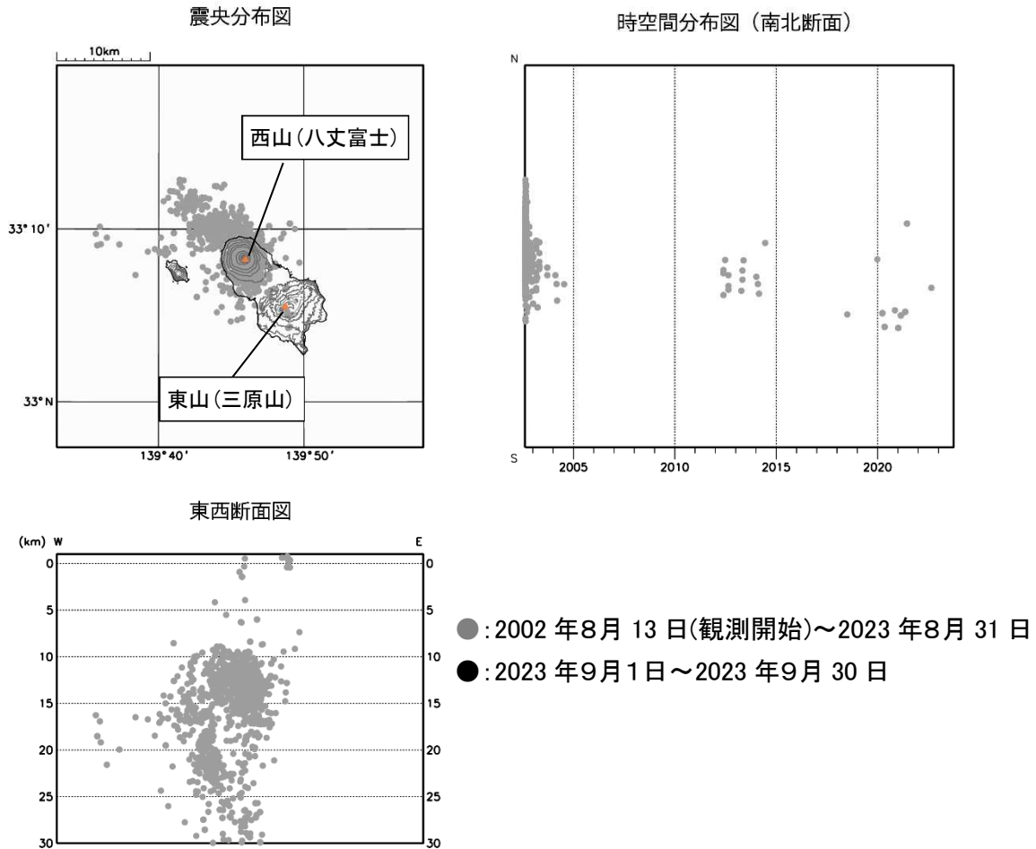
図3 八丈島 震源分布図（2002年8月13日～2023年9月30日）
