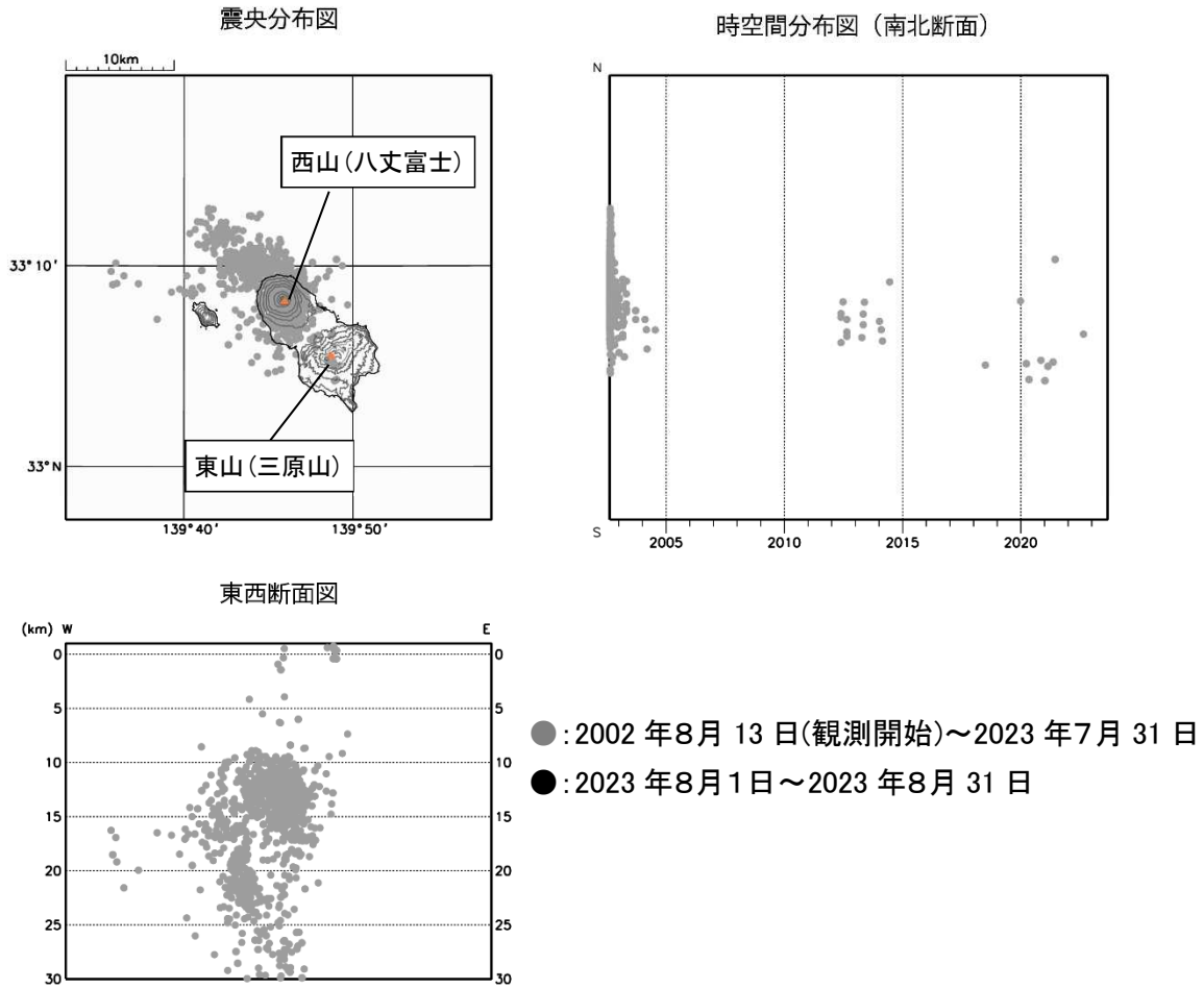
図3 八丈島 震源分布図（2002年8月13日～2023年8月31日）
