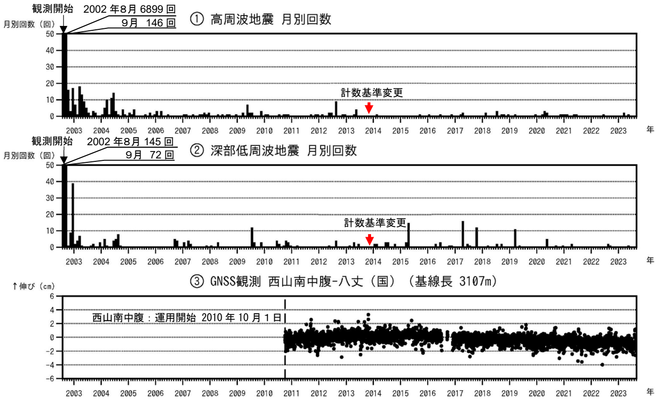
図2 八丈島 火山活動経過図（2002年8月13日～2023年8月31日）
