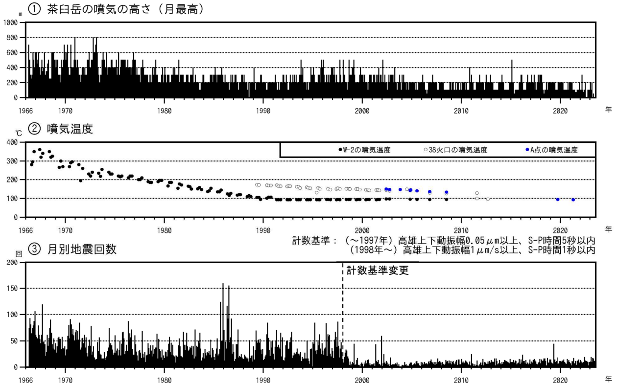
図3-1 那須岳 火山活動経過図（1966年5月～2023年7月）
