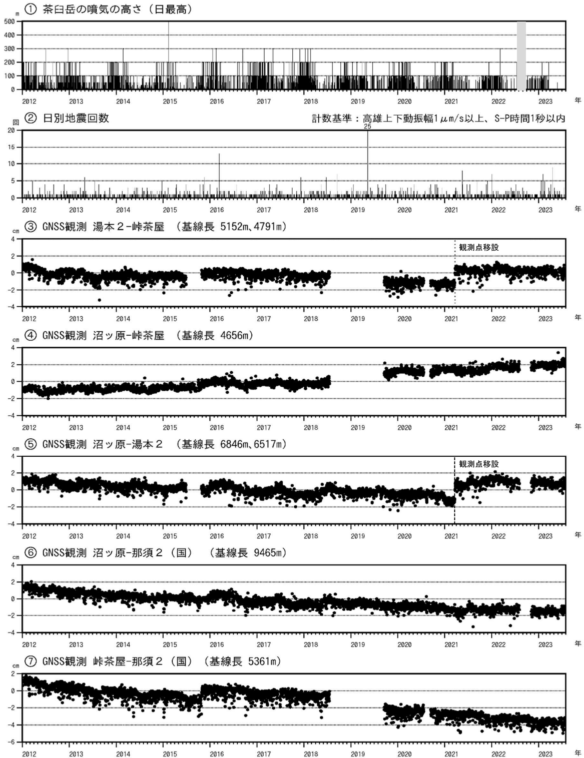
図4 那須岳 火山活動経過図（2012年1月1日～2023年7月31日）
