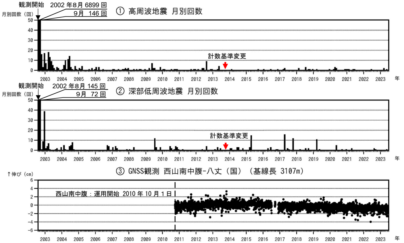
図2 八丈島 火山活動経過図（2002年8月13日～2023年6月30日）
