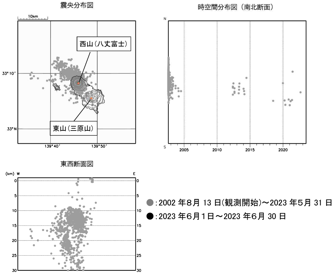
図3 八丈島 震源分布図（2002年8月13日～2023年6月30日）
