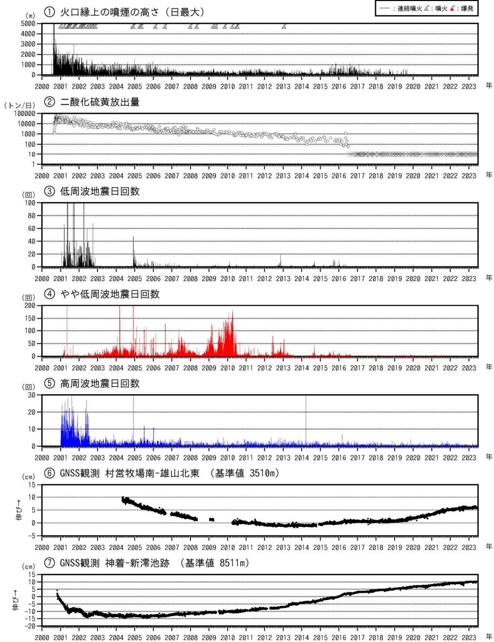
図7 三宅島 長期の火山活動経過図（2000年1月1日～2023年6月30日）
