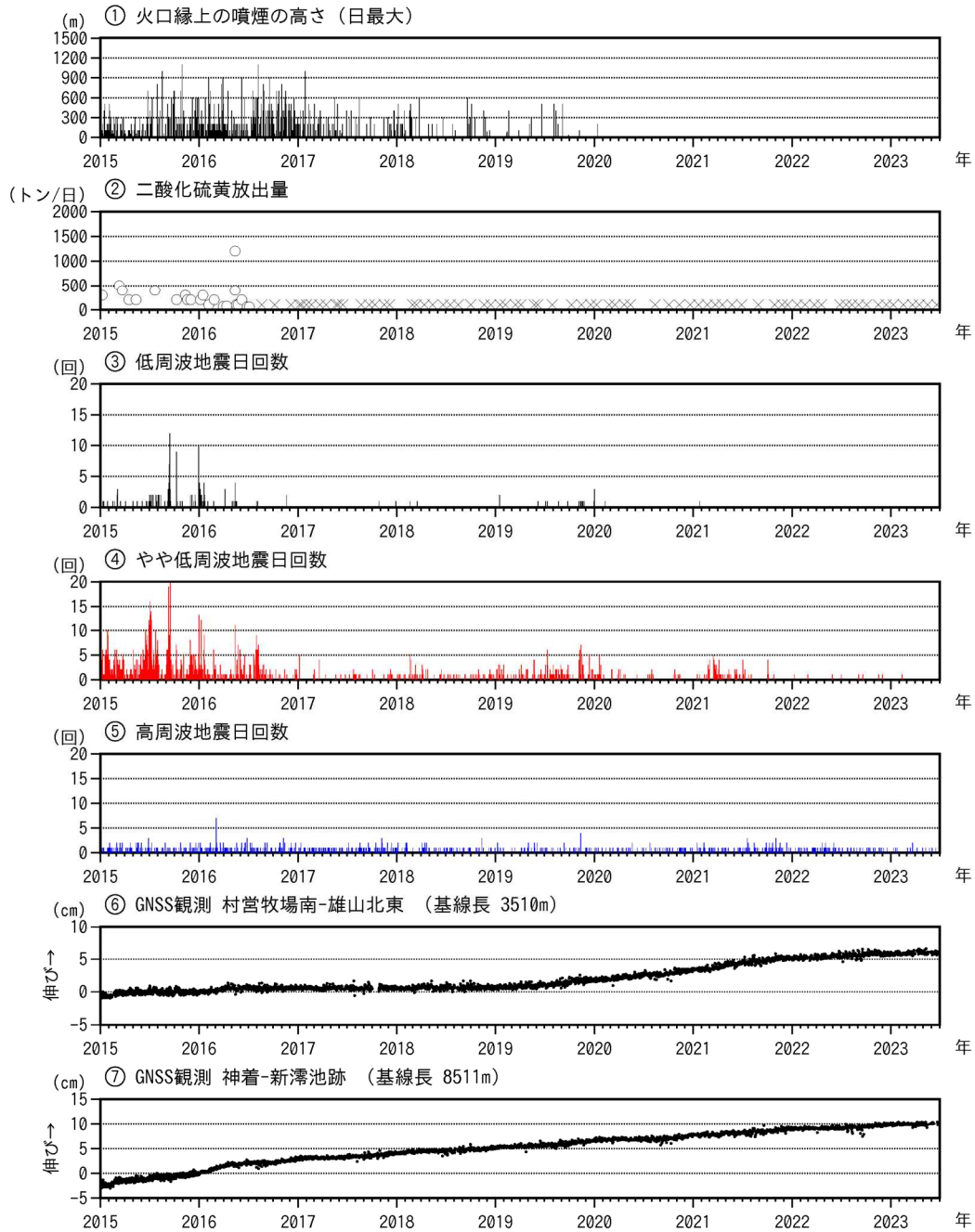
図6 三宅島 火山活動経過図（2015年1月1日～2023年6月30日）
