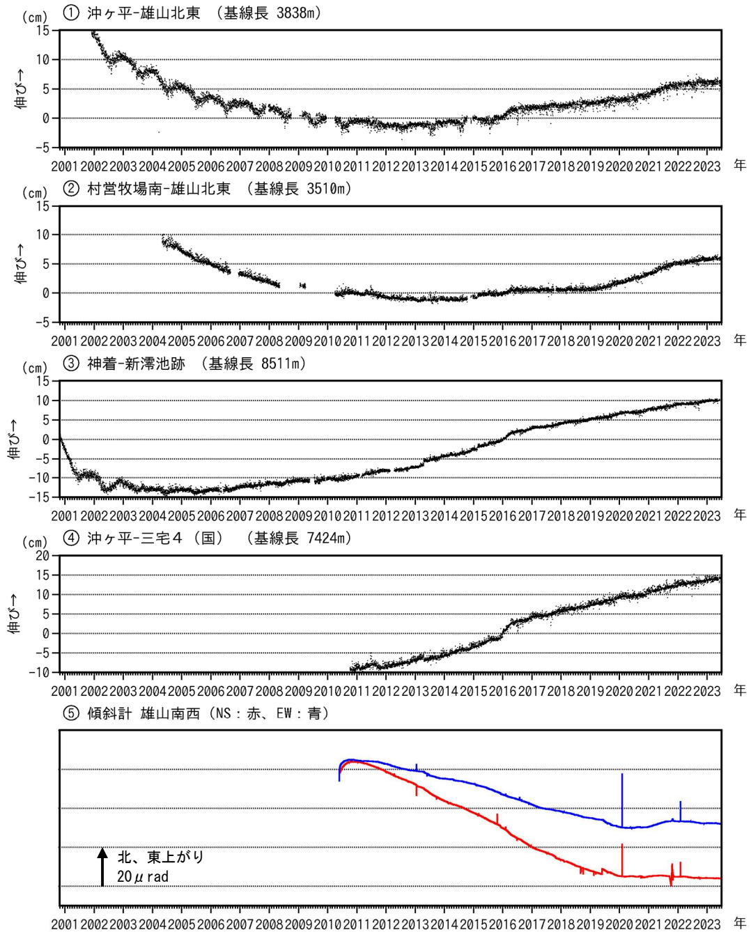
図8 三宅島 GNSS 連続観測及び傾斜計観測結果（2000年10月26日～2023年6月30日）
