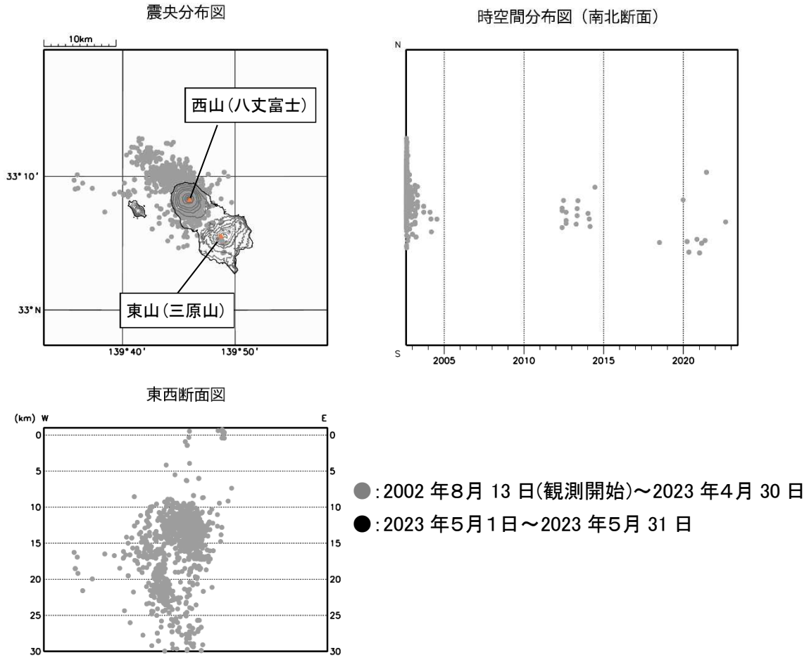
図3 八丈島 震源分布図（2002年8月13日～2023年5月31日）
