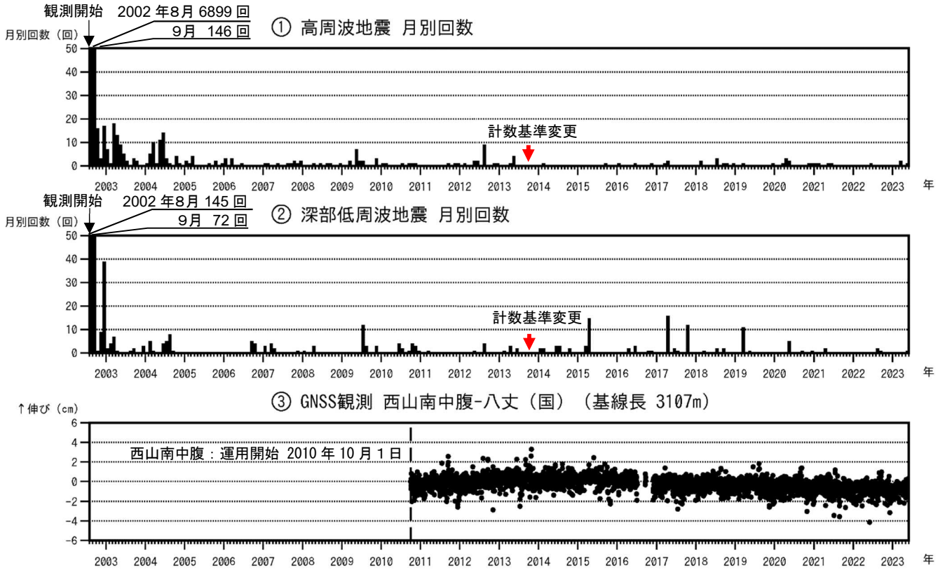
図2 八丈島 火山活動経過図（2002年8月13日～2023年5月31日）
