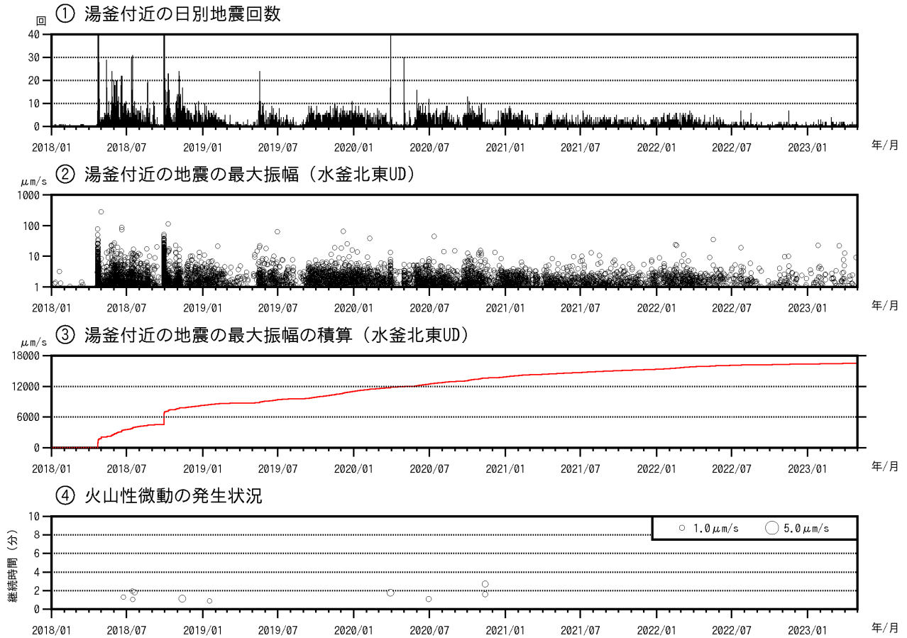
図1 草津白根山（白根山（湯釜付近）） 湯釜付近の地震活動及び火山性微動の発生状況 （2018年1月1日～2023年4月30日）
