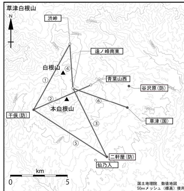
小さな白丸（○）は気象庁、小さな黒丸（●）は気象庁以外の機関の観測点位置を示しています。 (国)：国土地理院、(防)：防災科学技術研究所、(工)：東京工業大学、(関地)：関東地方整備局、(町)：草津町 国土地理院 数値地図 50mメッシュ (標高) 使用
