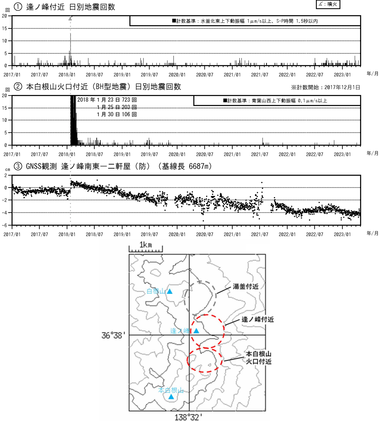
図13 草津白根山（本白根山） 火山活動経過図（2017年1月1日～2023年4月30日）
