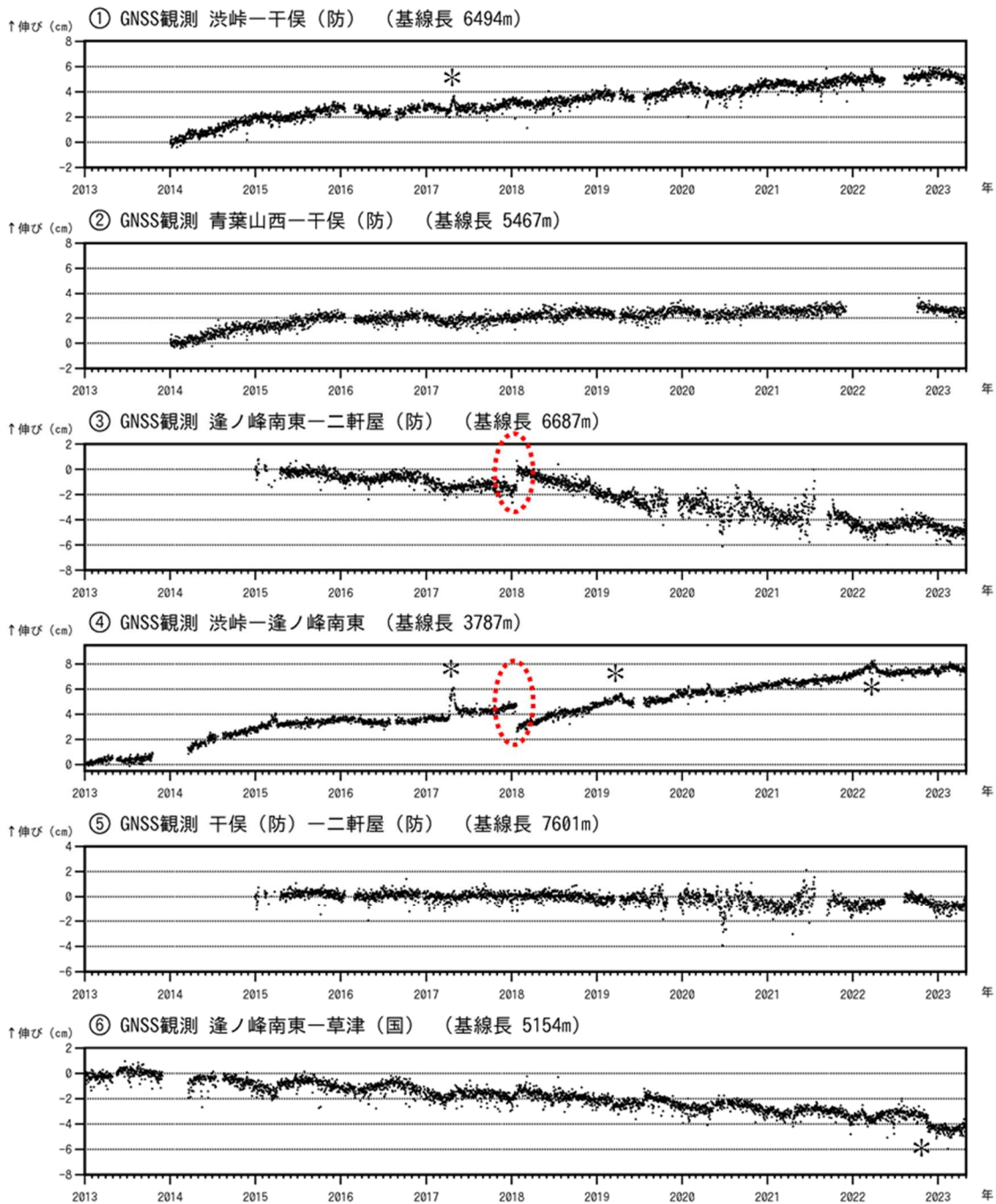
図6 草津白根山 GNSS連続観測の結果（2013年1月1日～2023年4月30日）
