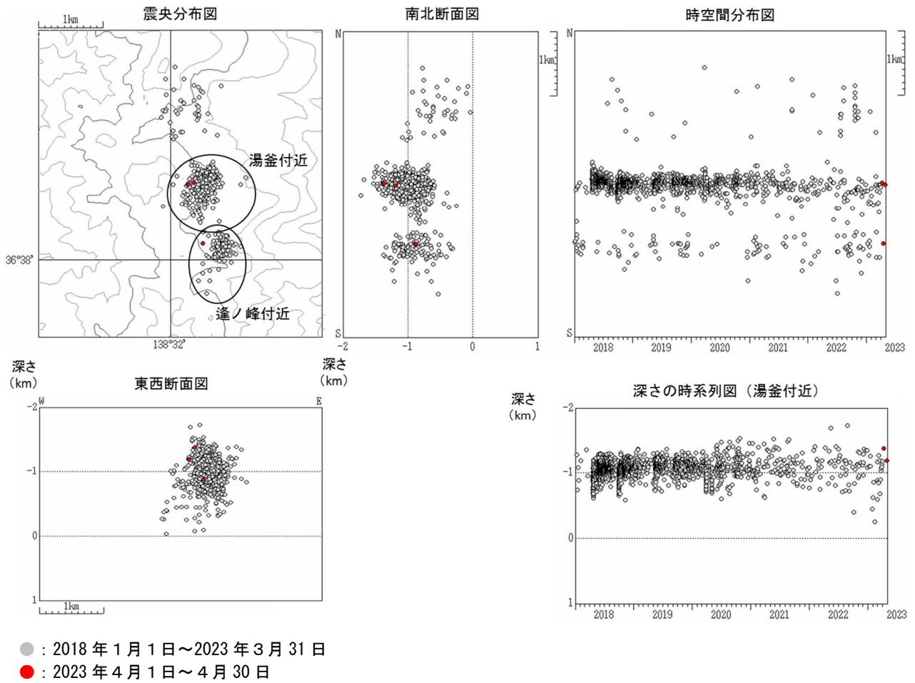
図4 草津白根山 震源分布図（2018年1月1日～2023年4月30日）
