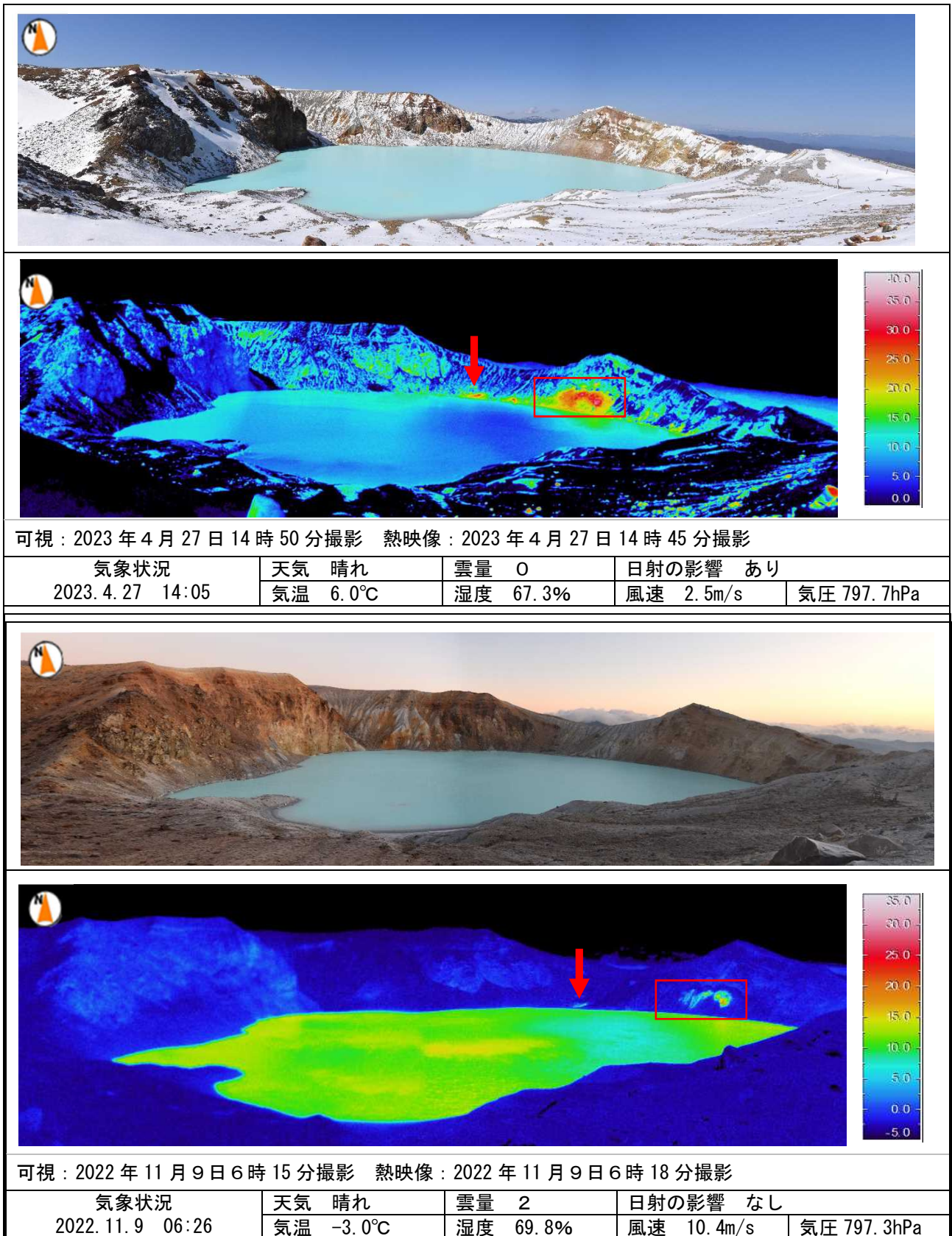
図2-2 草津白根山（白根山（湯釜付近）） 湯釜火口内の状況
