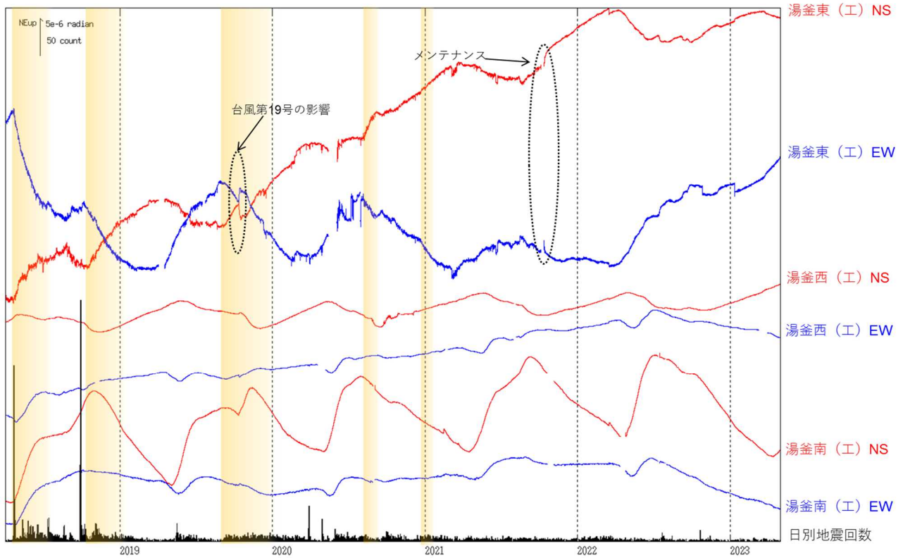
図5 草津白根山（白根山（湯釜付近）） 傾斜変動（2018年4月1日～2023年4月30日）
