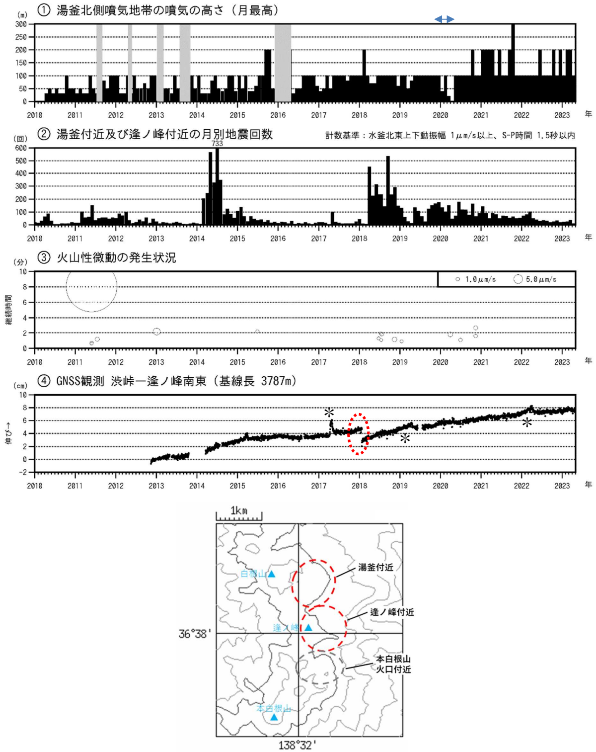
図3 草津白根山（白根山（湯釜付近））火山活動経過図（2010年1月1日～2023年4月30日）
