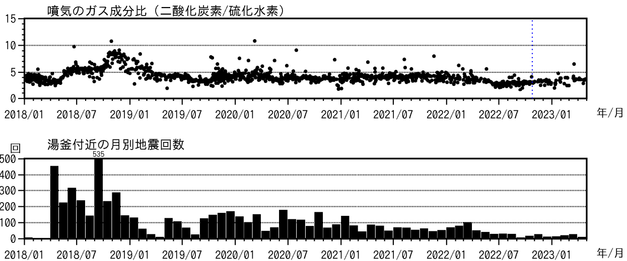
図8 草津白根山（白根山（湯釜付近）） 火山ガス観測結果（2018年1月～2023年4月）
