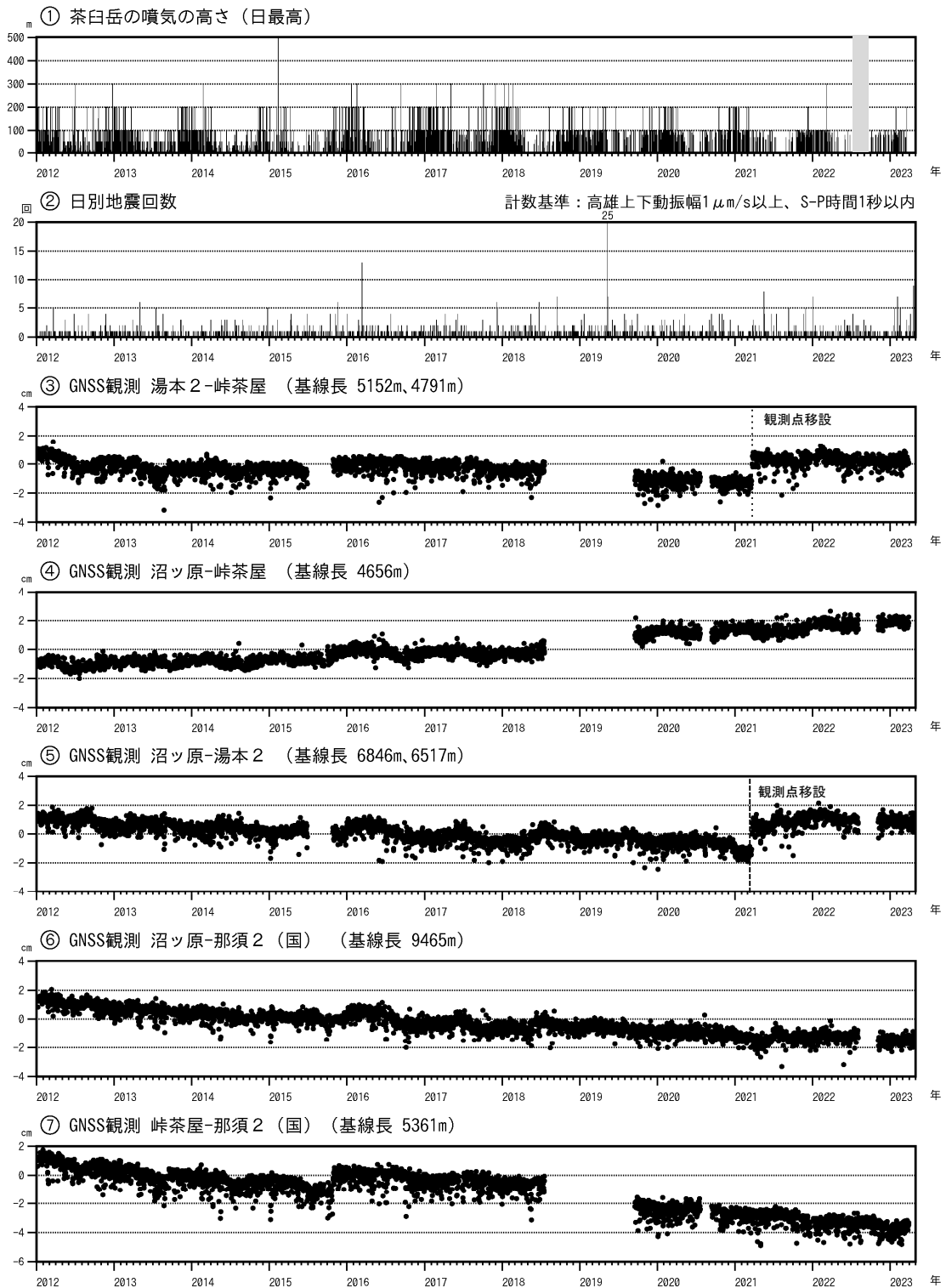
図4 那須岳 火山活動経過図（2012年1月1日～2023年4月30日）
