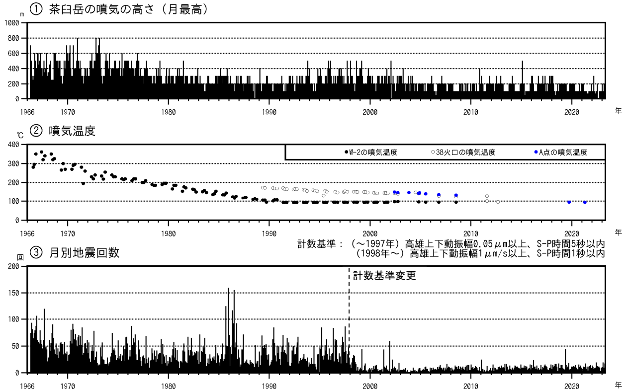
図3-1 那須岳 火山活動経過図（1966年5月～2023年4月）
