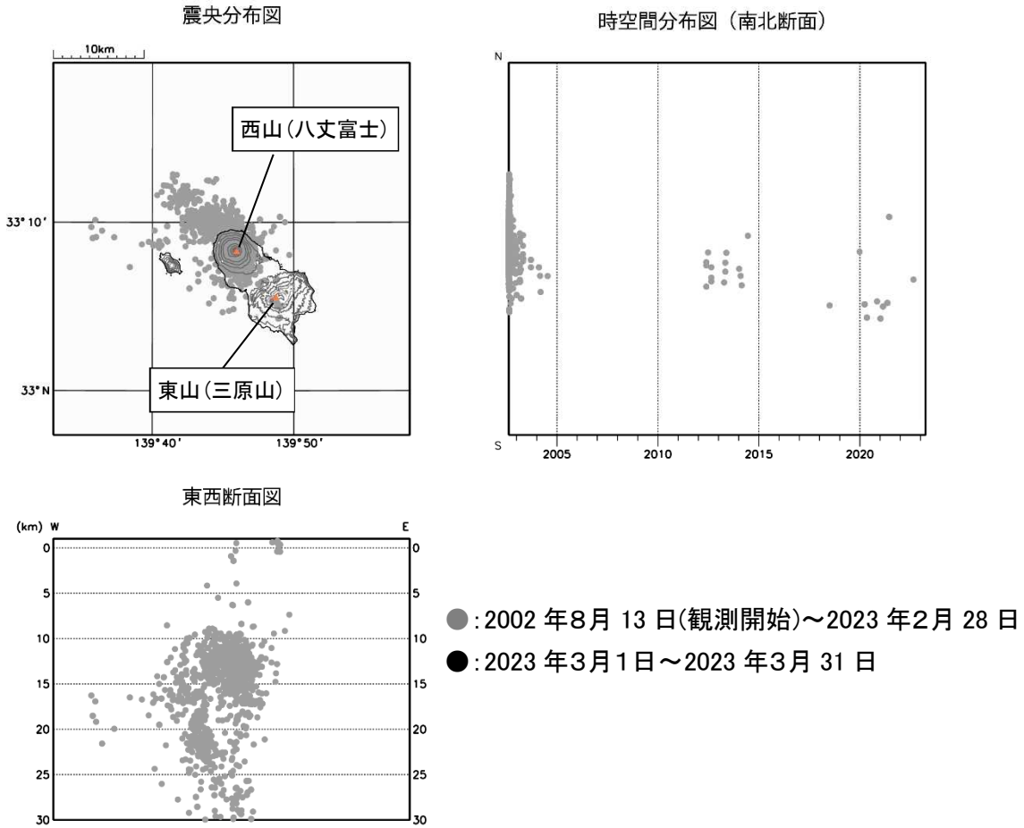
図3 八丈島 震源分布図（2002年8月13日～2023年3月31日）
