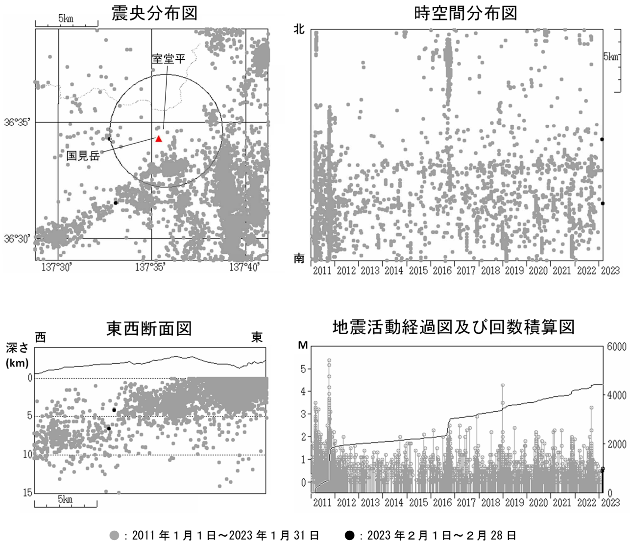
図2 弥陀ヶ原 広域地震観測網による山体・周辺の地震活動（2011 年 1 月 1 日～2023 年 2 月 28 日） 震央分布図中の円は弥陀ヶ原の計数対象地震（室堂平で S-P 時間 1 秒以内）のおよその範囲を示しています。 広域地震観測網により震源決定したもので、深さは全て海面以下として決定しています。 図中の震源要素は一部暫定値が含まれており、後日変更することがあります。 この図では、関係機関の地震波形を一元的に処理し、地震観測点の標高を考慮する等した手法で得られた震源を用いています（ただし、2020 年 8 月以前の地震については火山活動評価のための参考震源です）。
