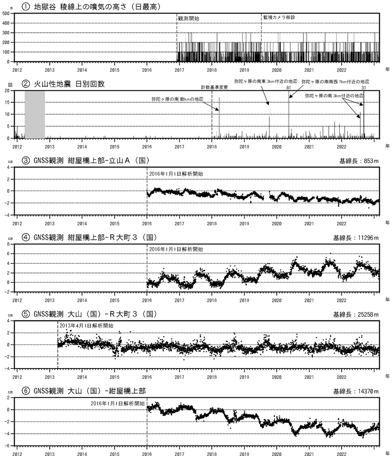
図3 弥陀ヶ原 火山活動経過図（2011年12月1日～2023年2月28日）
