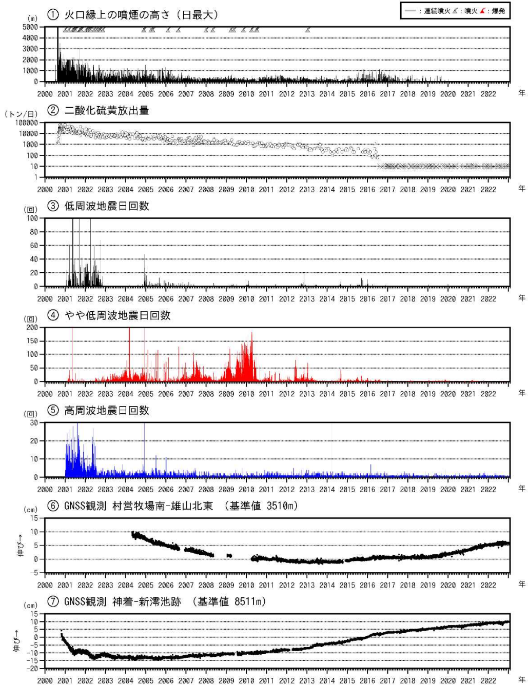
図5 三宅島 長期の火山活動経過図（2000年1月1日～2023年1月31日）
