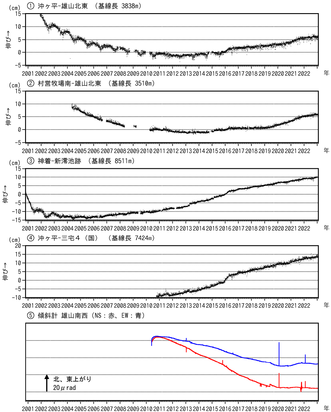
図6 三宅島 GNSS 連続観測及び傾斜計観測結果（2000年10月26日～2023年1月31日）
