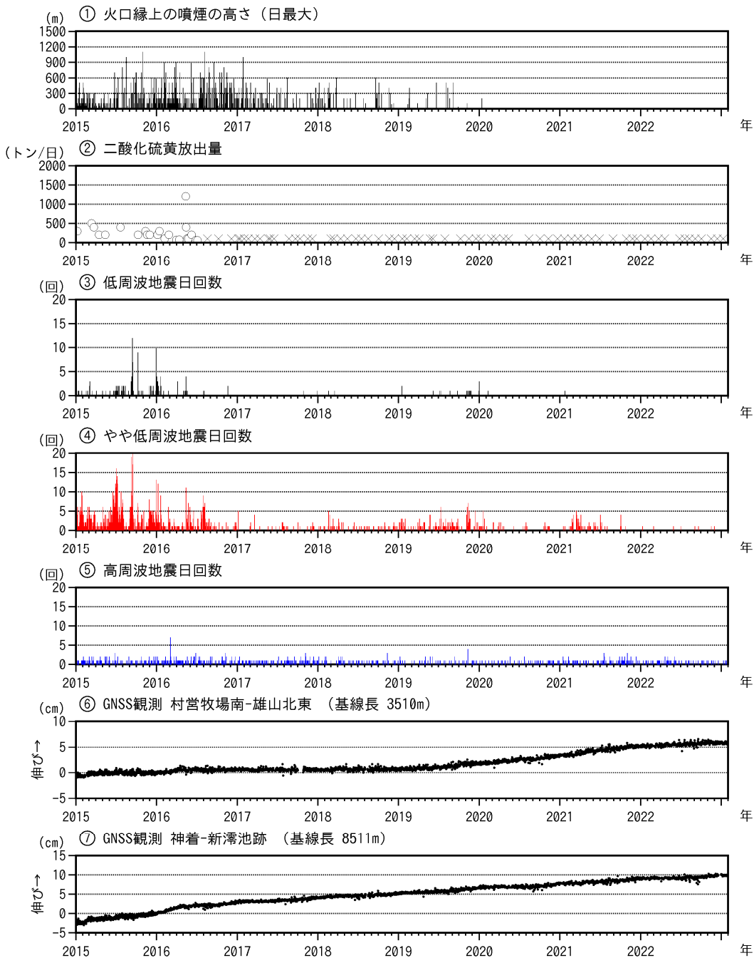
図4 三宅島 火山活動経過図（2015年1月1日～2023年1月31日）
