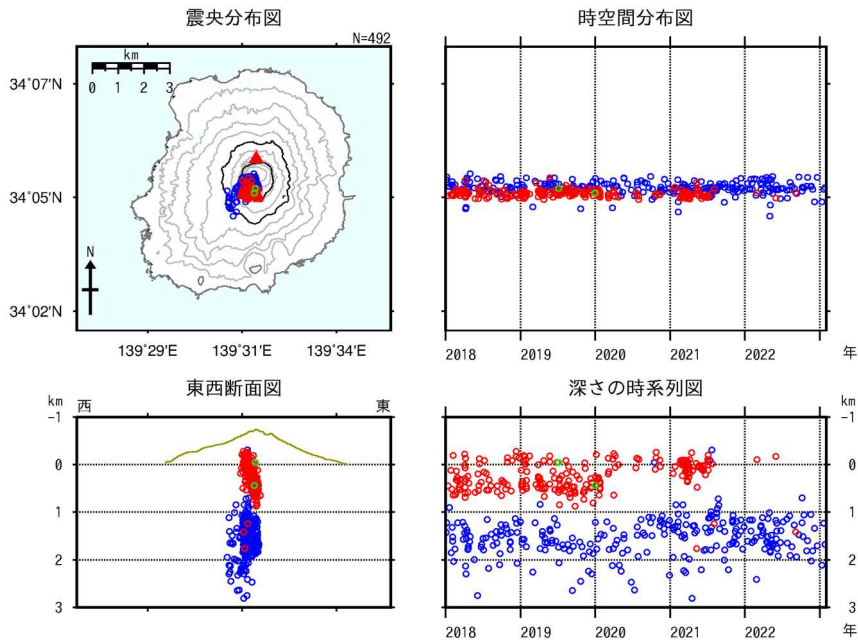
図7 三宅島 震源分布図
