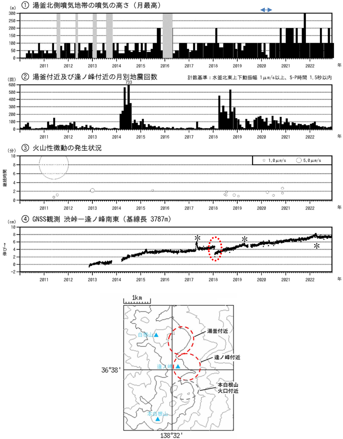
図3 草津白根山（白根山（湯釜付近）） 火山活動経過図（2010年1月1日～2022年11月30日）
