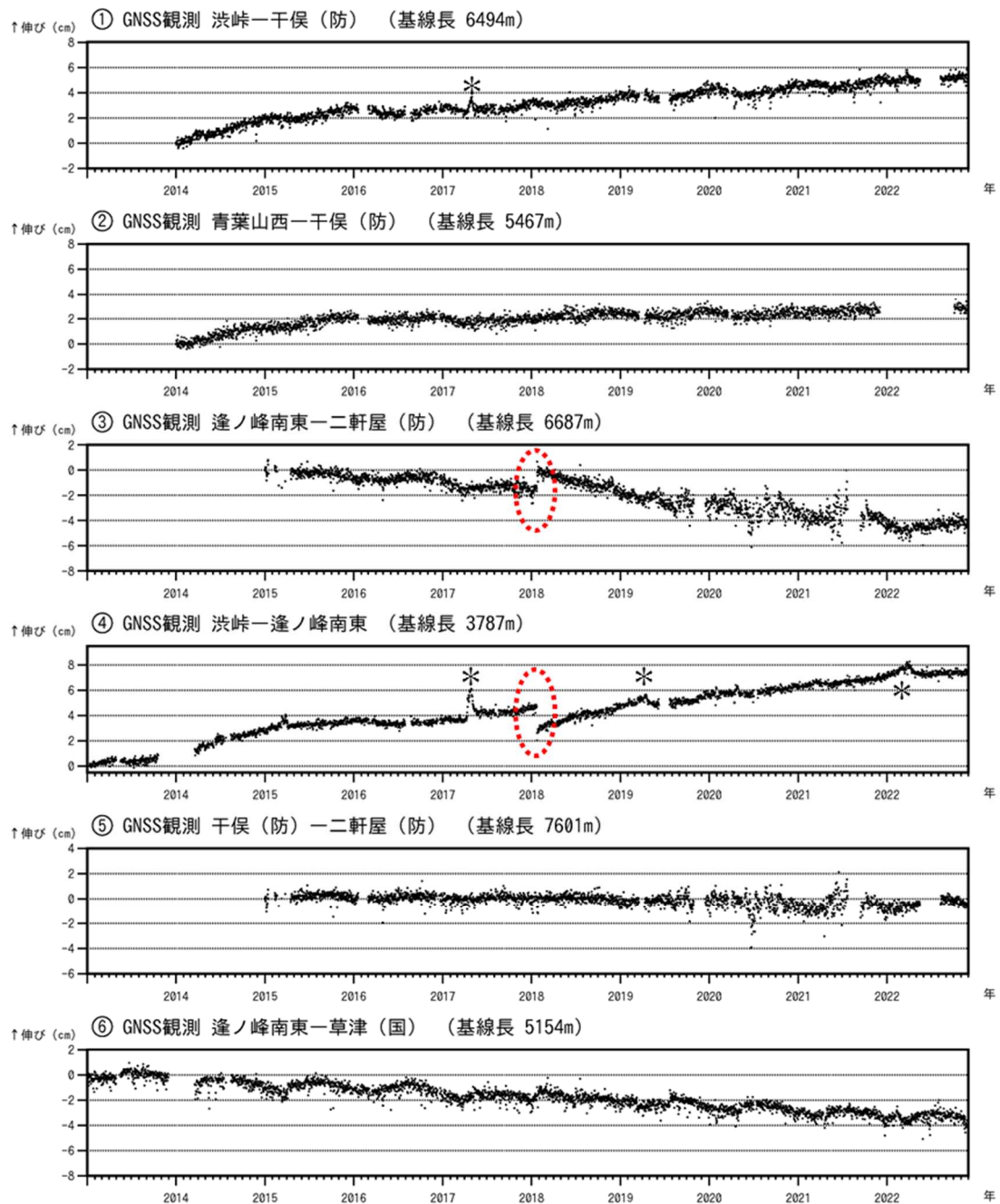
図6 草津白根山 GNSS連続観測の結果（2013年1月1日～2022年11月30日）
