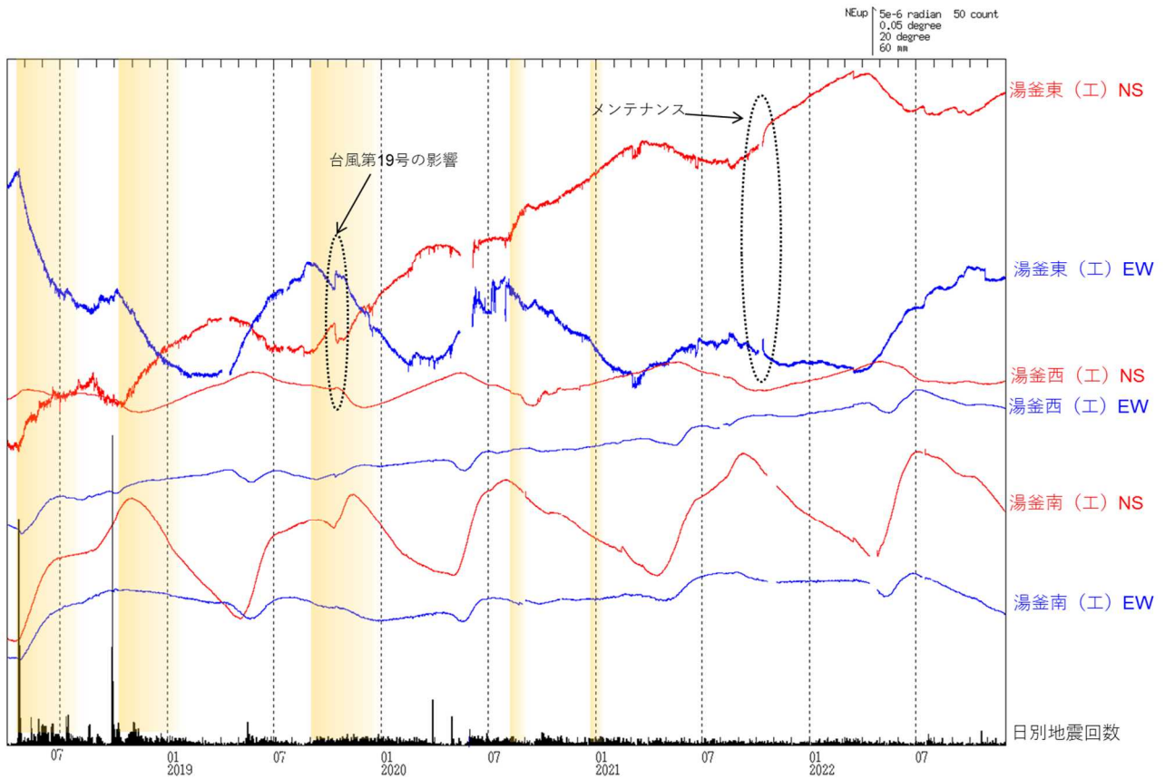
図5 草津白根山（白根山（湯釜付近）） 傾斜変動（2018年4月1日～2022年11月30日） (工)：東京工業大学
