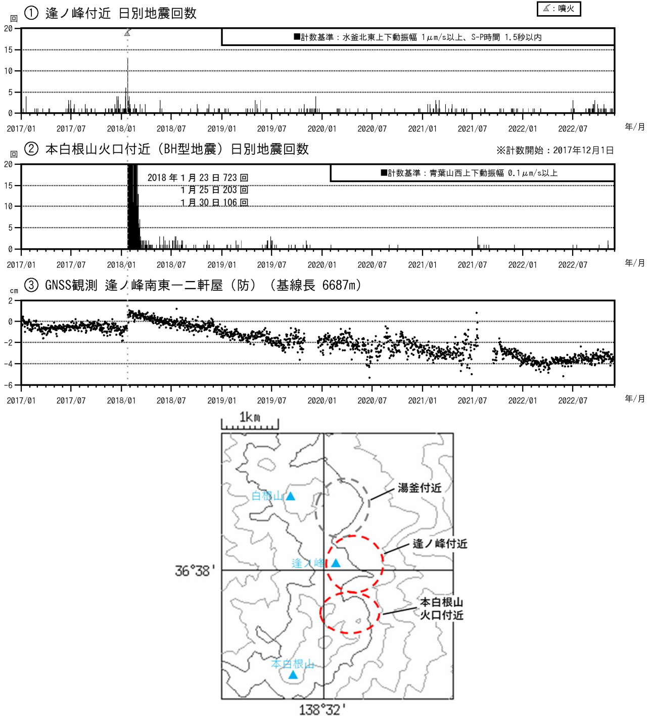
図12 草津白根山（本白根山） 火山活動経過図（2017年1月1日～2022年11月30日）
