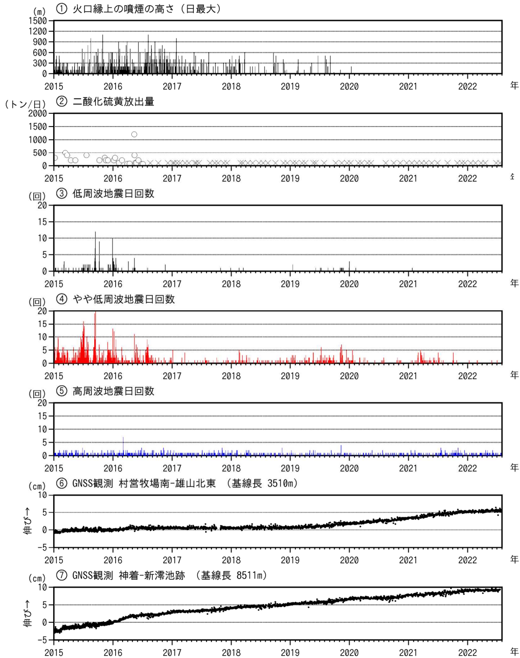
図6 三宅島 火山活動経過図（2015年1月1日～2022年7月31日）
