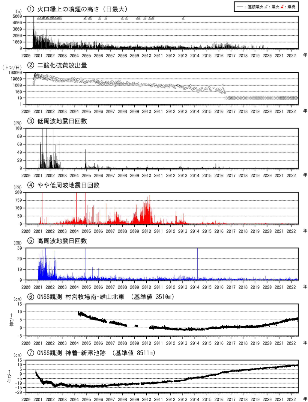
図7 三宅島 長期の火山活動経過図（2000年1月1日～2022年7月31日）
