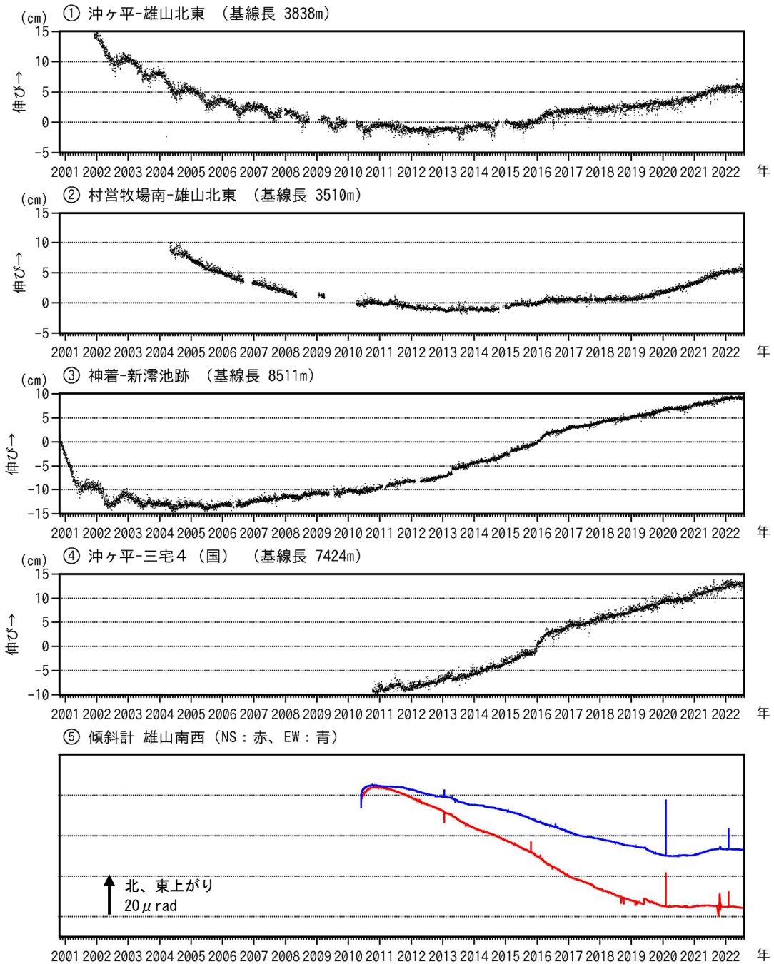
図8 三宅島 GNSS 連続観測及び傾斜計観測結果（2000年10月26日～2022年7月31日）
