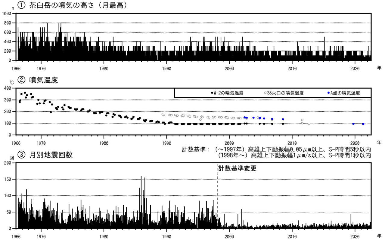
図3-1 那須岳 火山活動経過図（1966年5月～2022年7月）
