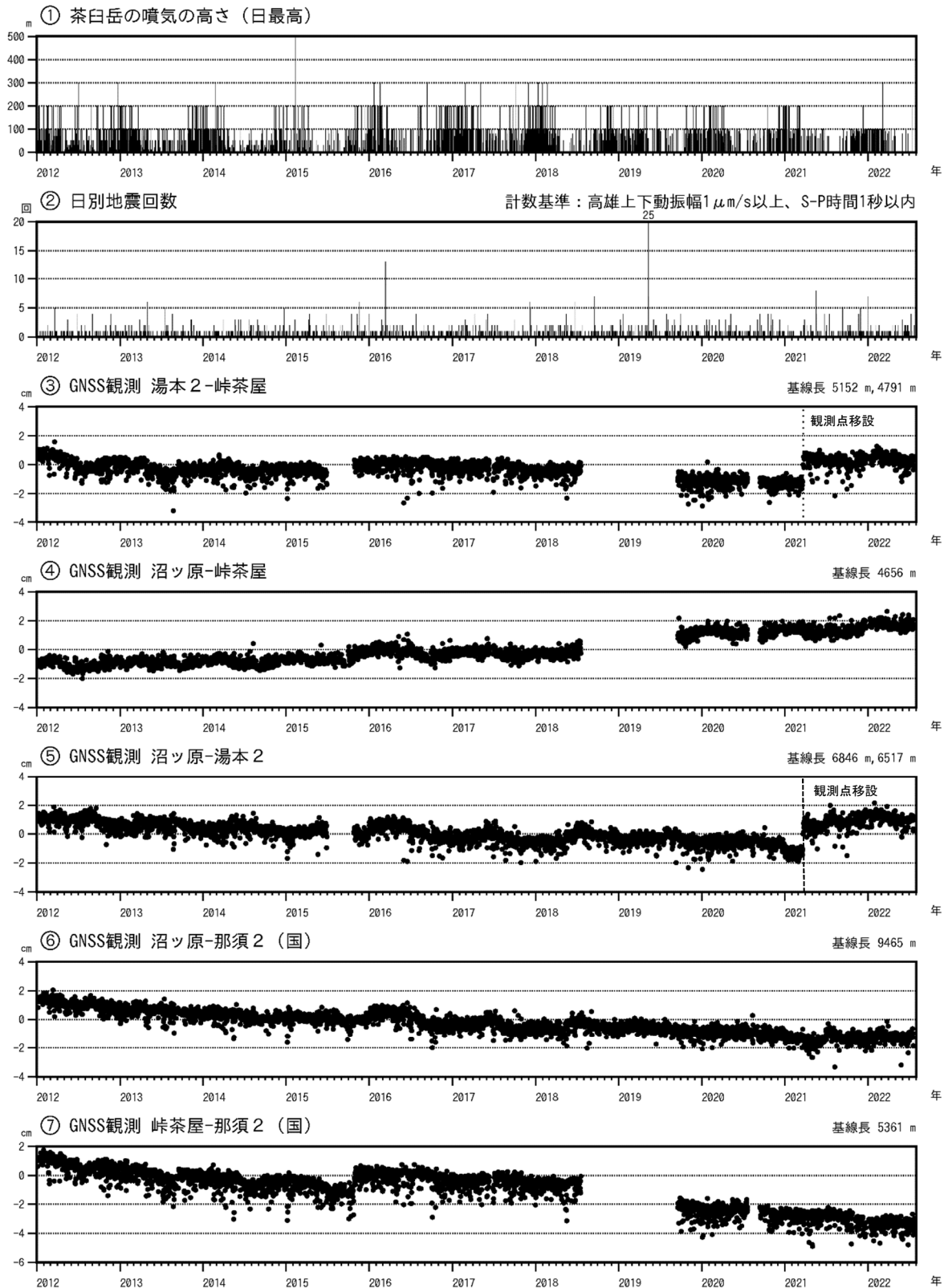
図4 那須岳 火山活動経過図（2012年1月1日～2022年7月31日）
