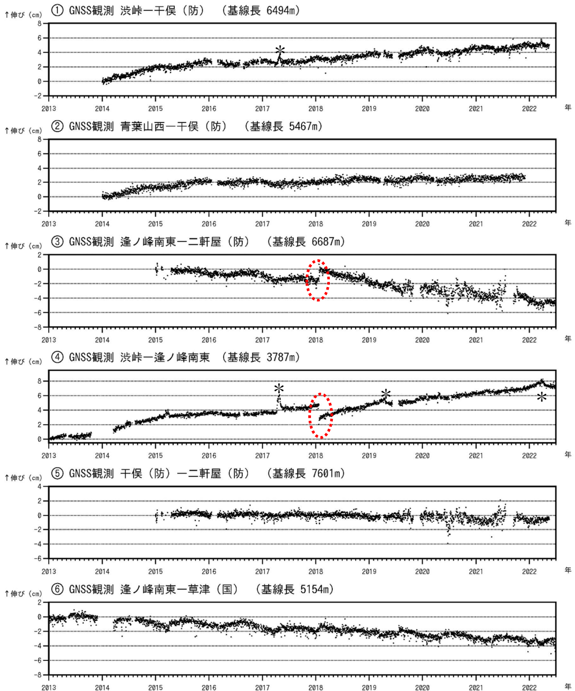
図6 草津白根山 GNSS連続観測の結果 (2013年1月1日~2022年6月30日)
