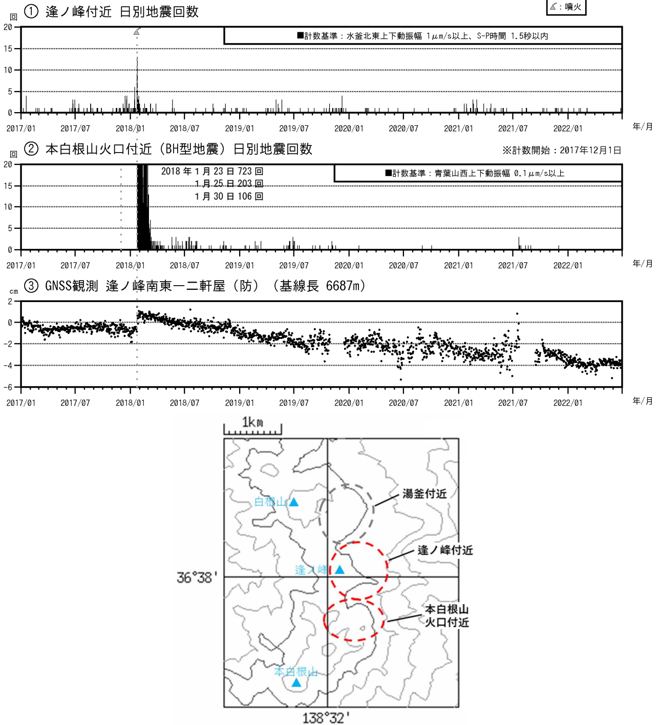
図9 草津白根山（本白根山） 火山活動経過図（2017年1月1日～2022年6月30日）
