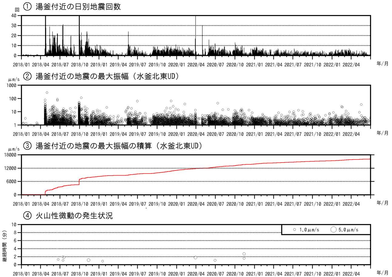
図1 草津白根山（白根山（湯釜付近）） 湯釜付近の地震活動及び火山性微動の発生状況 （2018年1月1日～2022年6月30日）
