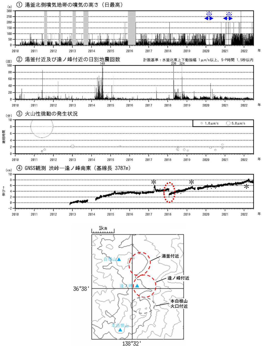
図3 草津白根山（白根山（湯釜付近））火山活動経過図（2010年1月1日～2022年6月30日）
