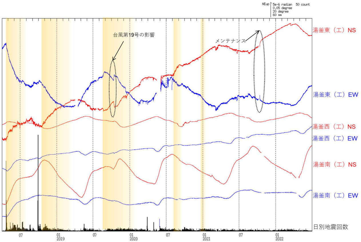
図5 草津白根山（白根山（湯釜付近）） 傾斜変動（2018年4月1日～2022年6月30日） (工)：東京工業大学
