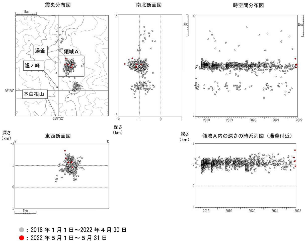
図6 草津白根山 震源分布図（2018年1月1日～2022年5月31日）
