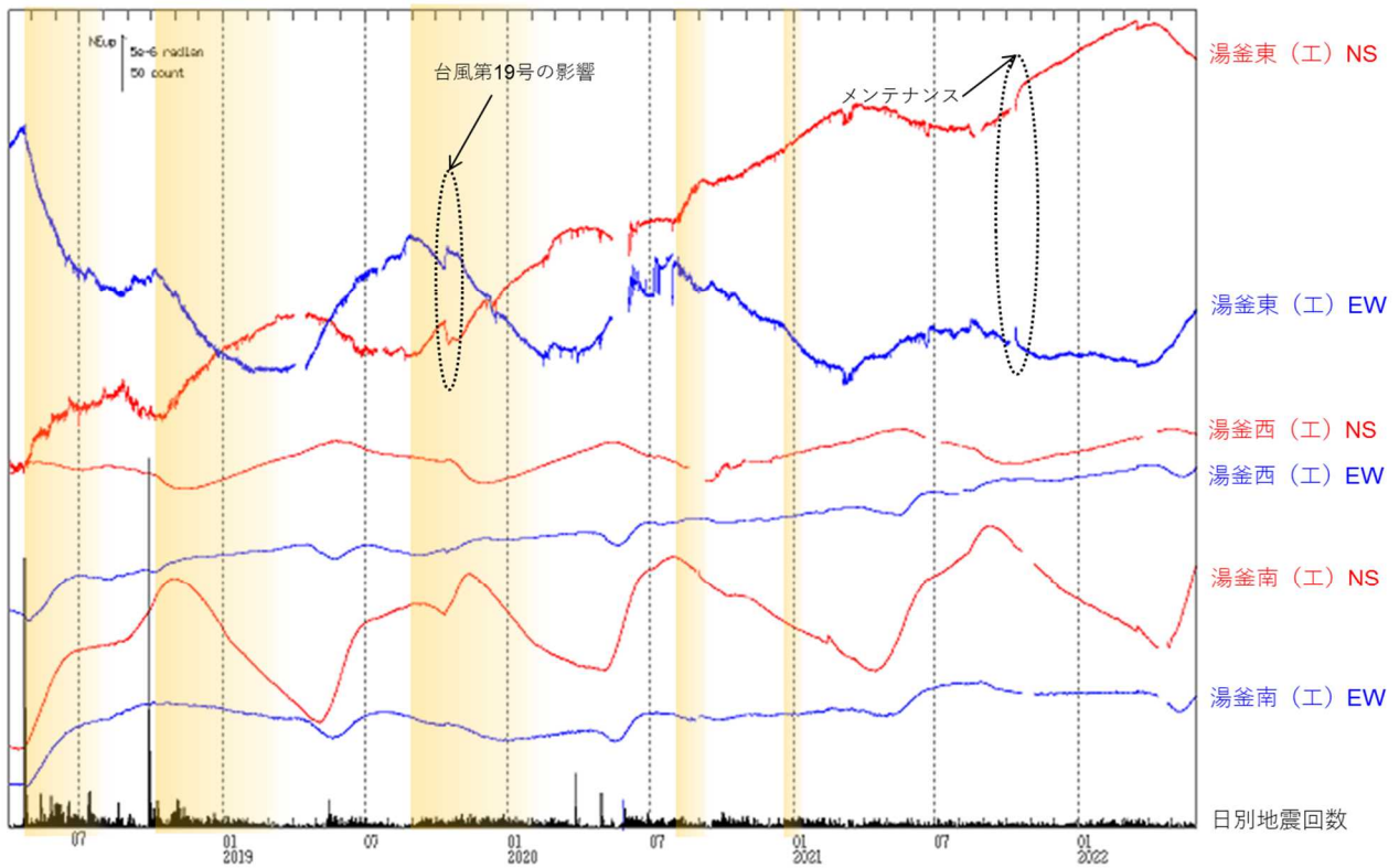
図7 草津白根山（白根山（湯釜付近）） 傾斜変動（2018年4月1日～2022年5月31日）
