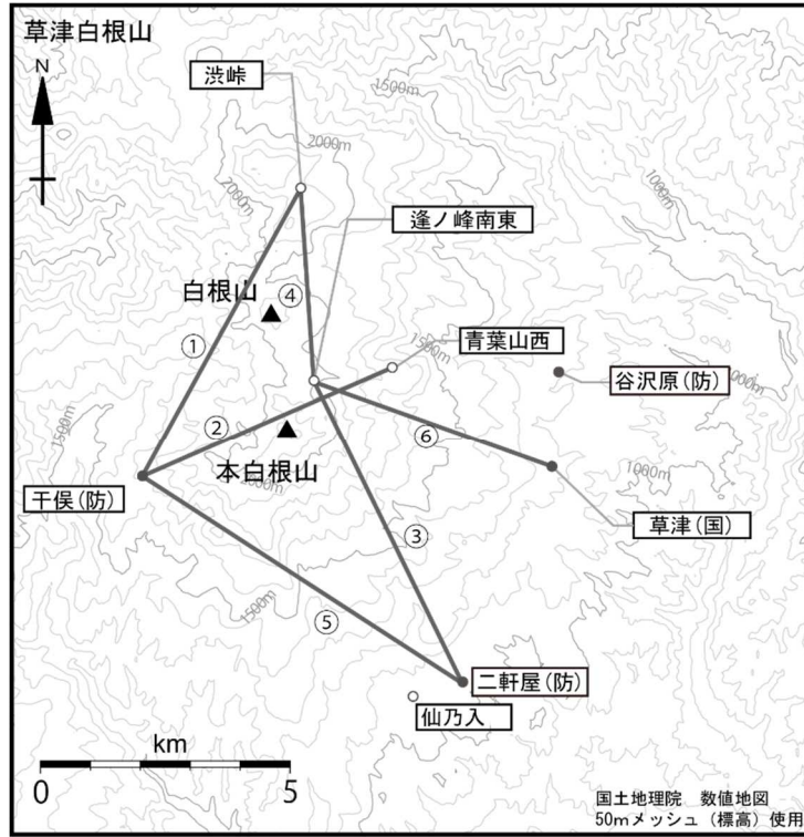
図9 草津白根山 GNSS 観測点配置図
