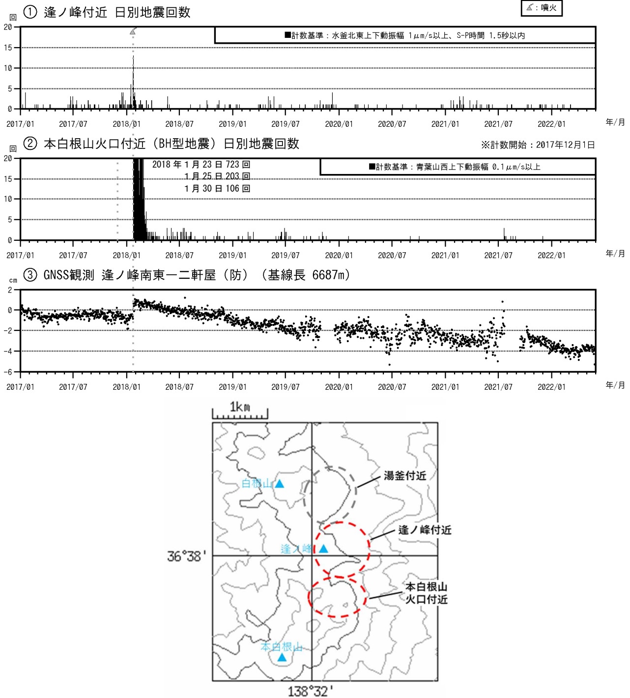
図13 草津白根山（本白根山） 火山活動経過図（2017年1月1日～2022年5月31日）
