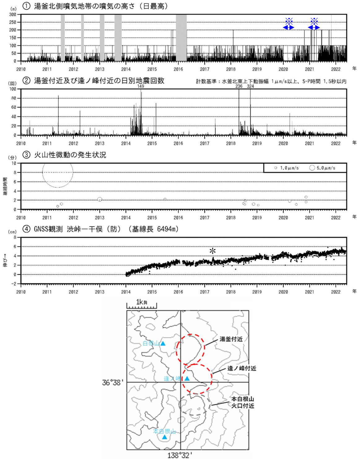
図5 草津白根山（白根山（湯釜付近）） 火山活動経過図（2010年1月1日～2022年5月31日）
