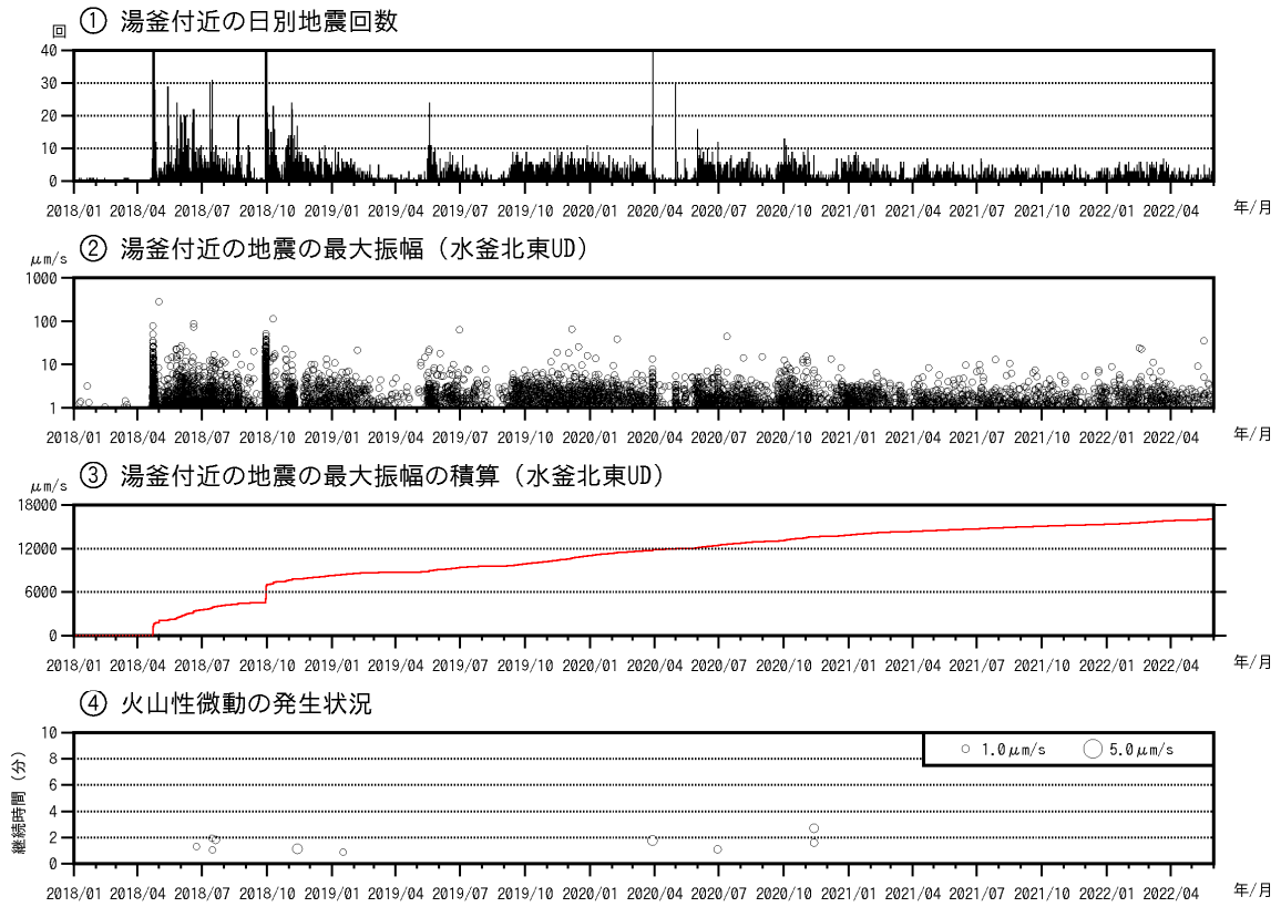
図1 草津白根山（白根山（湯釜付近）） 湯釜付近の地震活動及び火山性微動の発生状況 （2018年1月1日～2022年5月31日）
