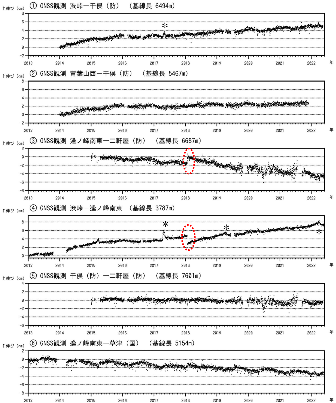
図8 草津白根山 GNSS連続観測の結果（2013年1月1日～2022年5月31日）
