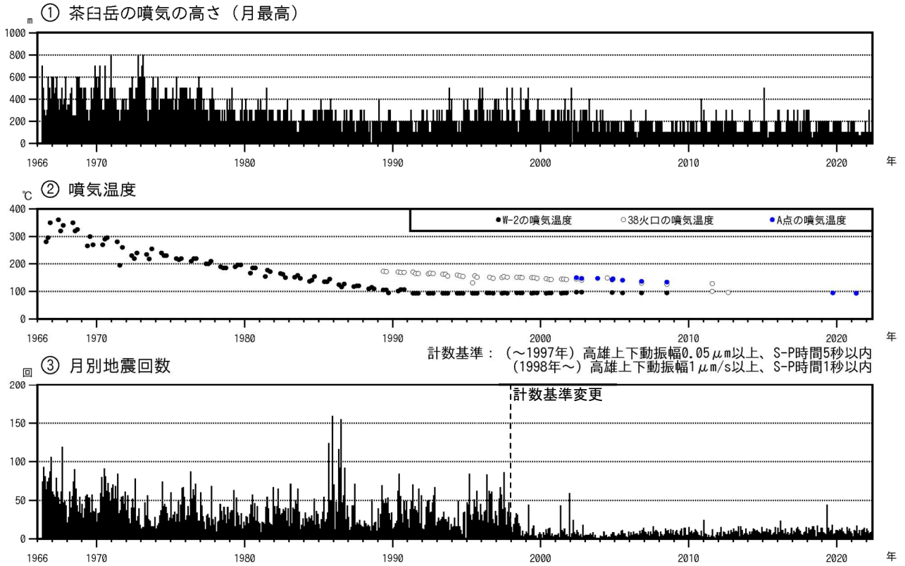
図3-1 那須岳 火山活動経過図（1966年5月～2022年5月）
