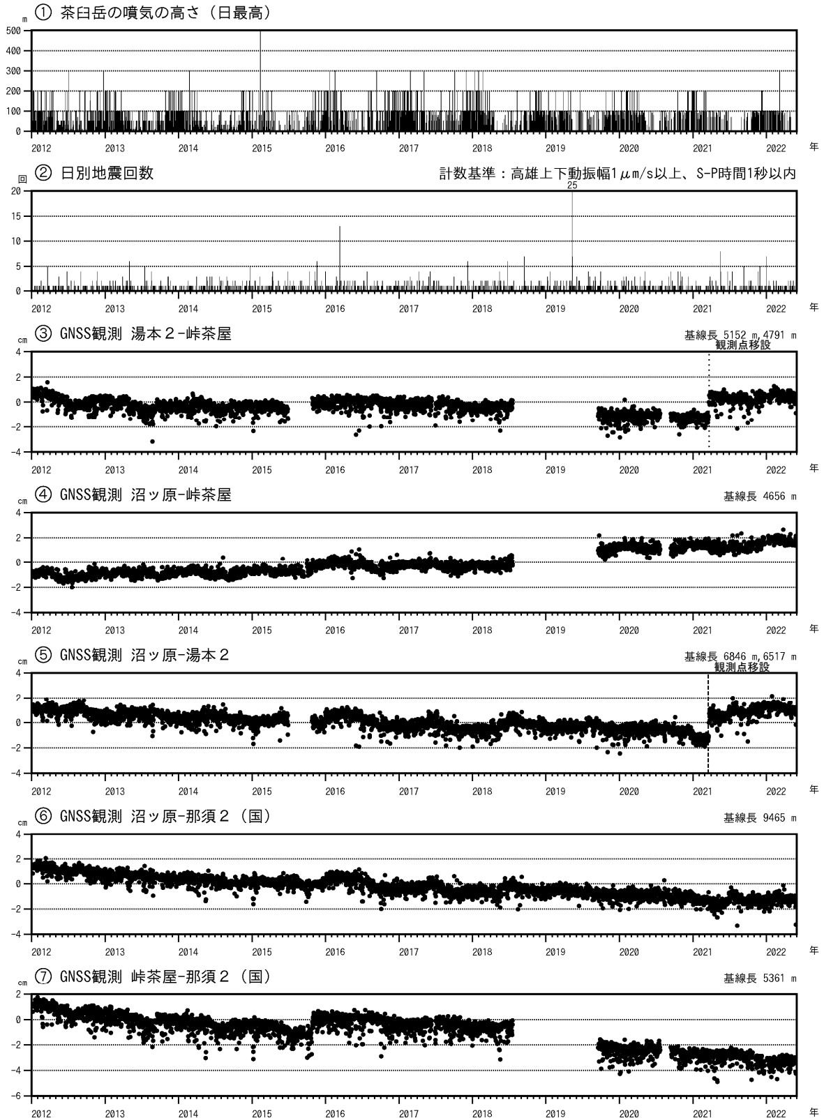
図4 那須岳 火山活動経過図（2012年1月1日～2022年5月31日）
