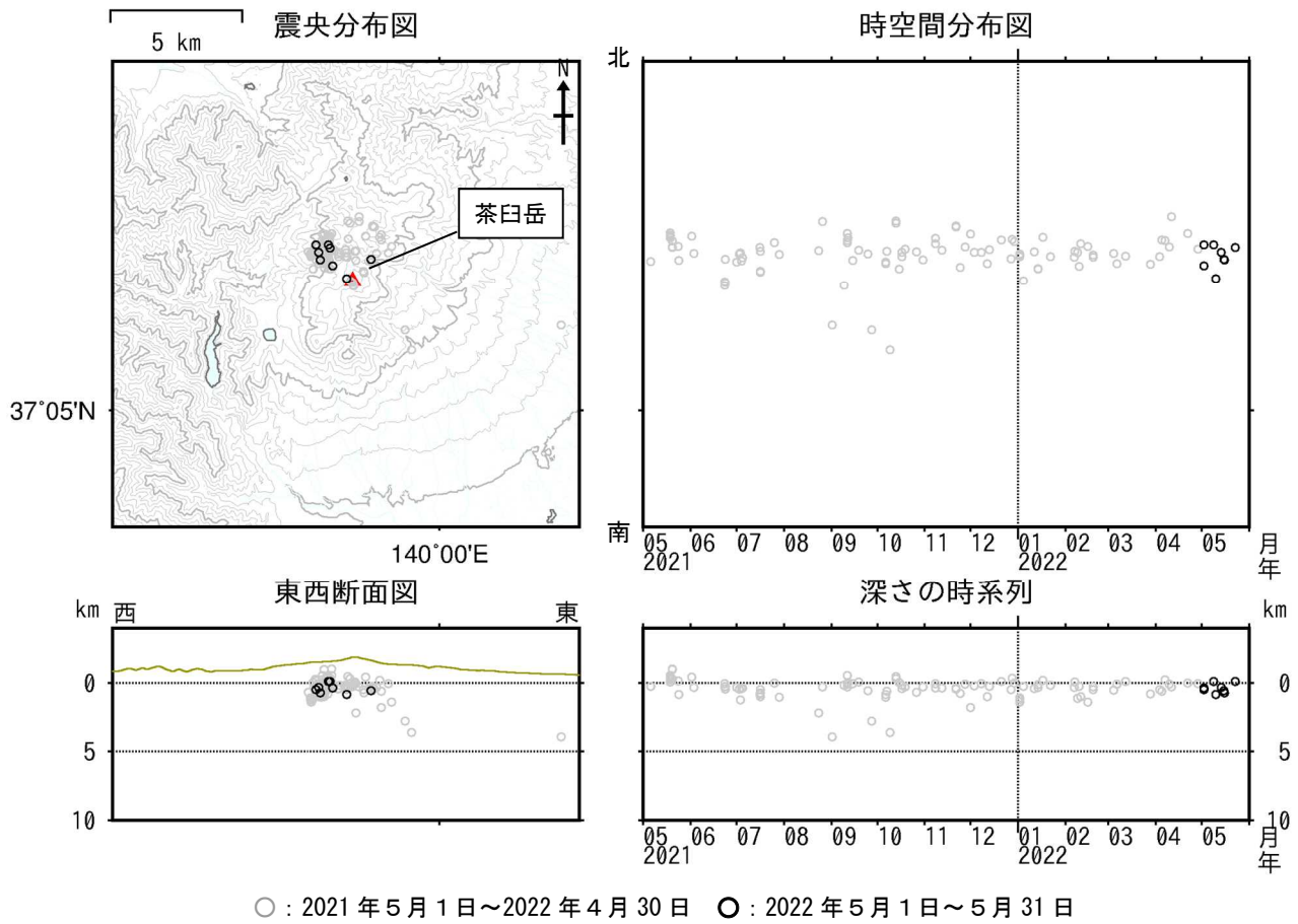
図5 那須岳 震源分布図（2021年5月1日～2022年5月31日）
