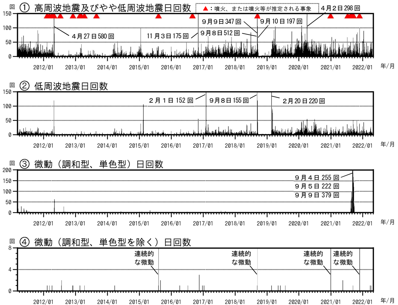
図4 硫黄島 長期火山活動経過図（2011年3月8日～2022年4月30日）
