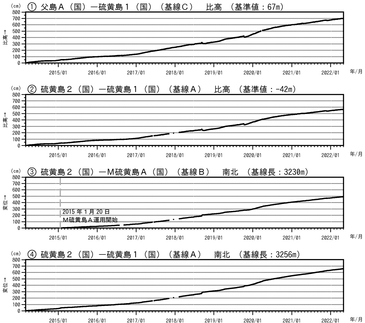
図5 硫黄島 GNSS 連続観測結果（2014 年 3 月 1 日～2022 年 4 月 30 日）
