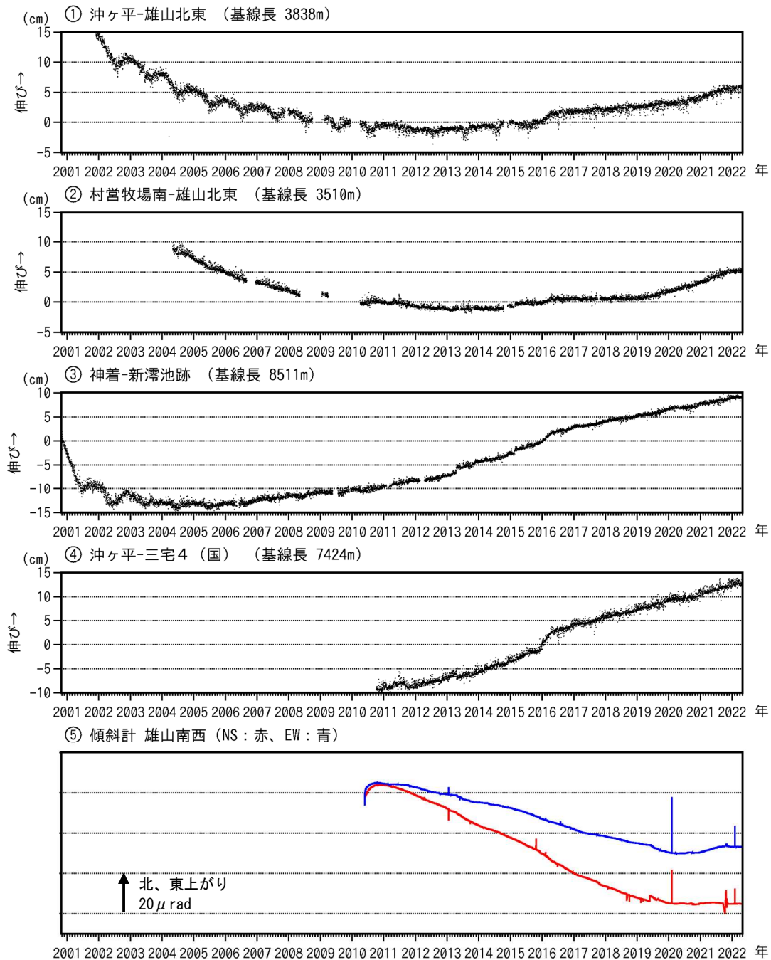
図8 三宅島 GNSS 連続観測及び傾斜計観測結果 (2000年10月26日~2022年4月30日)
