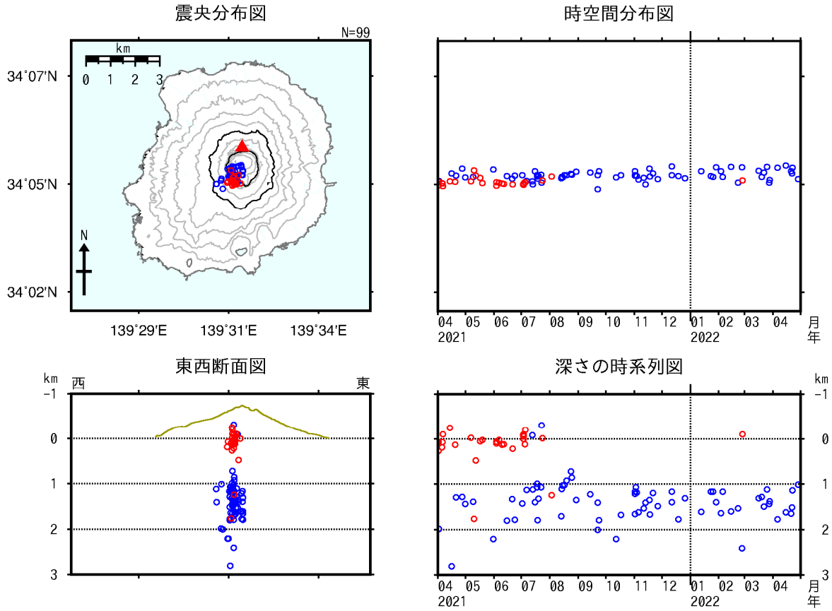
図9 三宅島 震源分布図（2021年4月1日～2022年4月30日）
