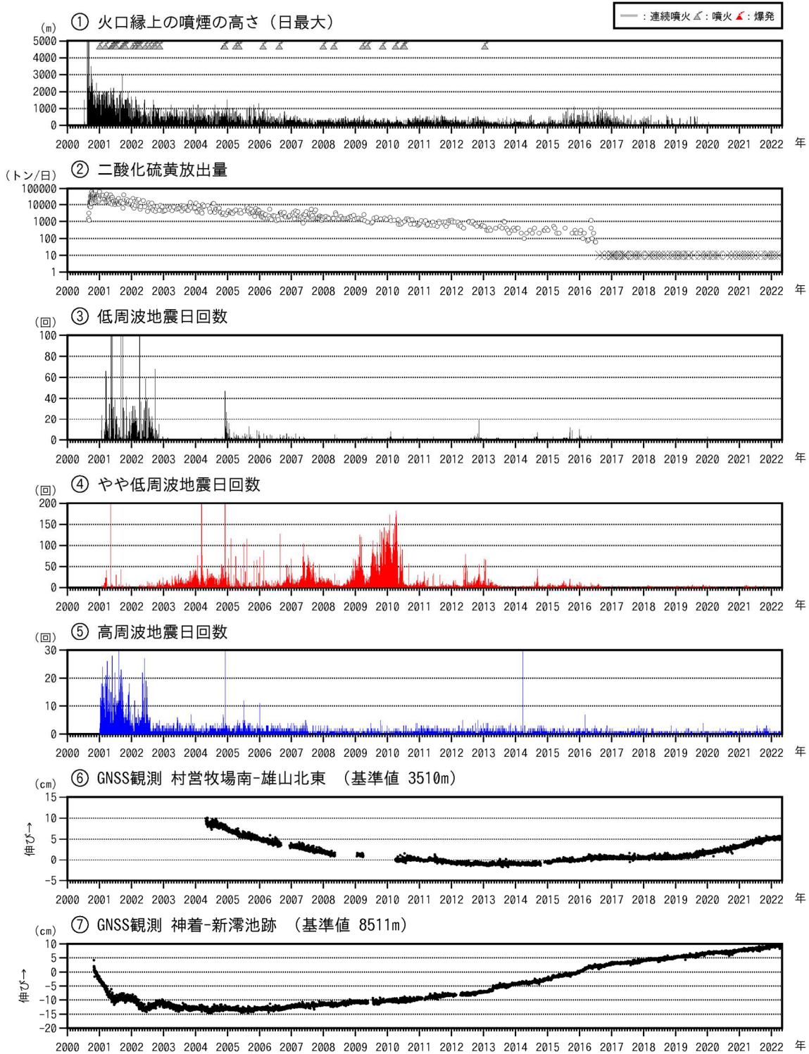
図6 三宅島 長期の火山活動経過図（2000年1月1日～2022年4月30日） ※図6の説明は次ページに掲載。
