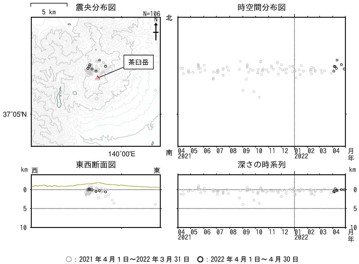
図5 那須岳 震源分布図（2021年4月1日～2022年4月30日）
