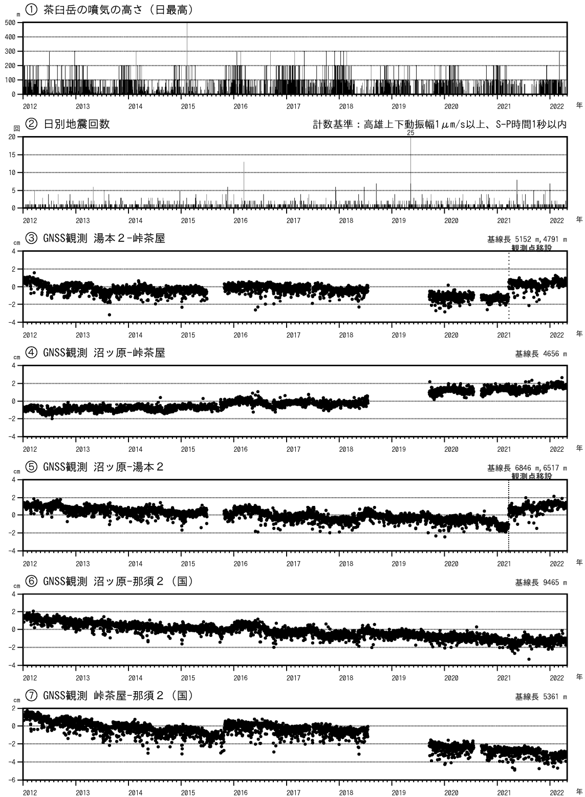
図4 那須岳 火山活動経過図（2012年1月1日～2022年4月30日）
