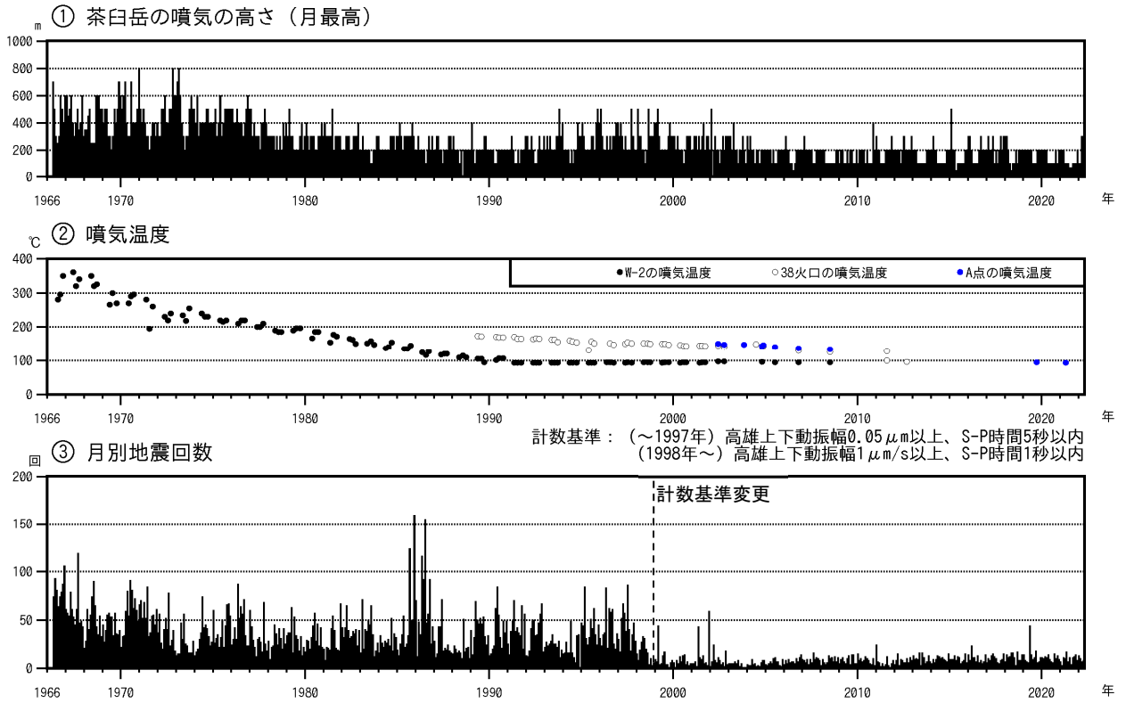
図3-1 那須岳 火山活動経過図（1966年5月～2022年4月）
