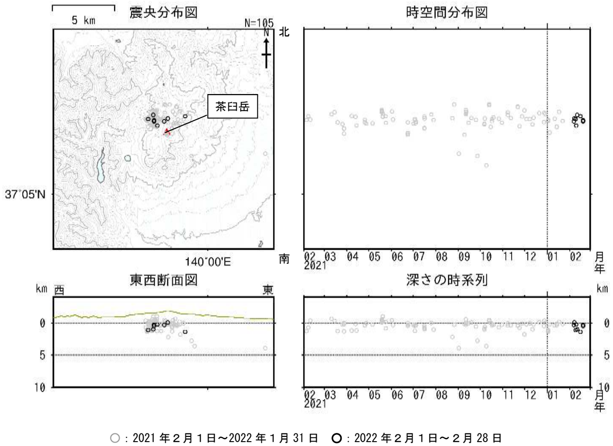
図5 那須岳 震源分布図（2021年2月1日～2022年2月28日）
