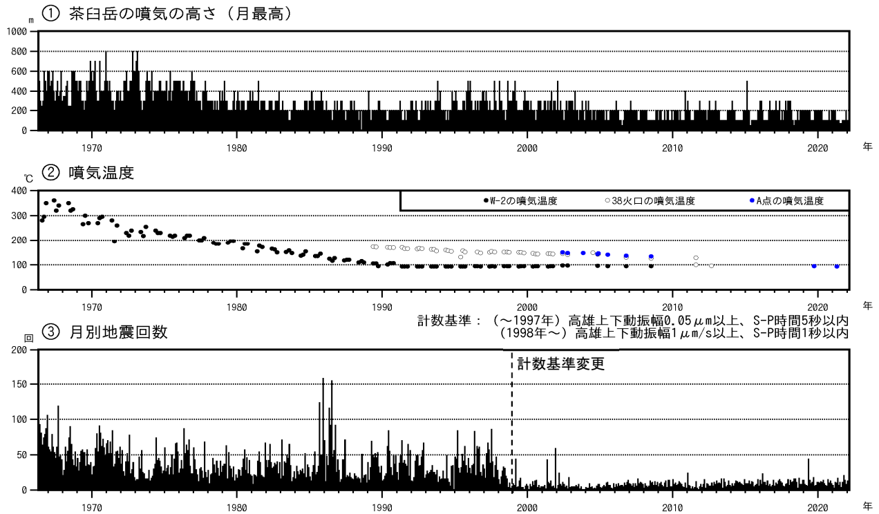
図3-1 那須岳 火山活動経過図（1966年5月～2022年2月）
