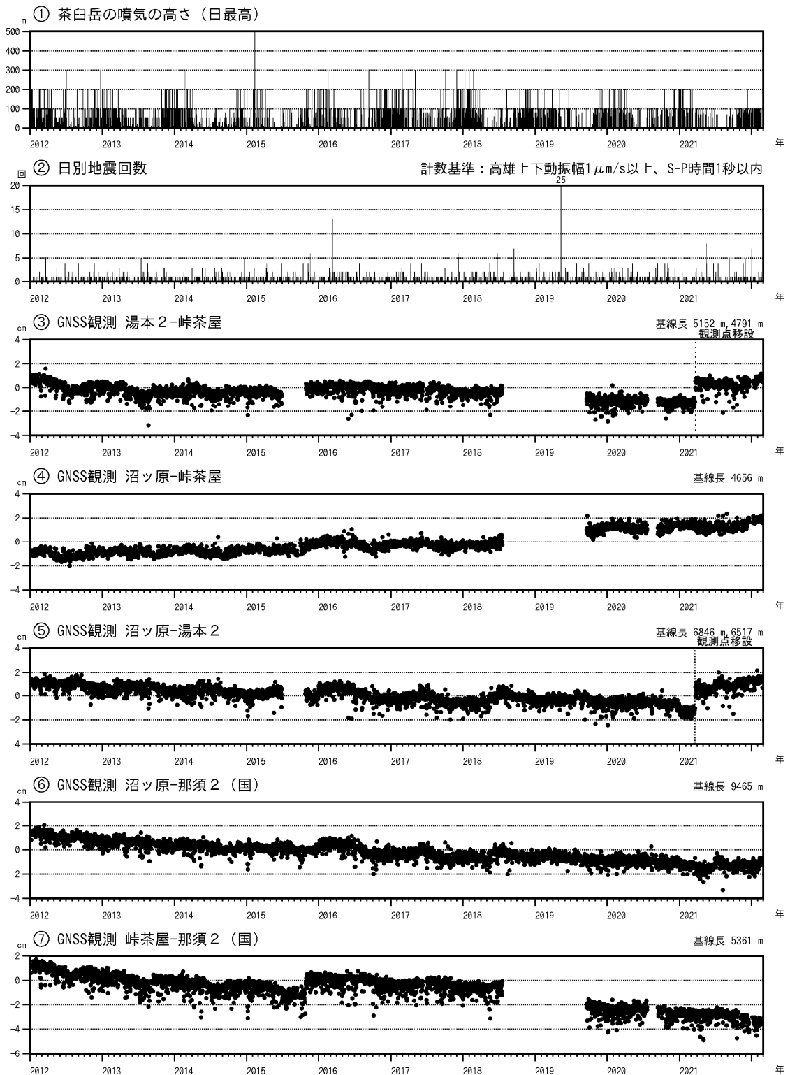
図4 那須岳 火山活動経過図（2012年1月1日～2022年2月28日）
