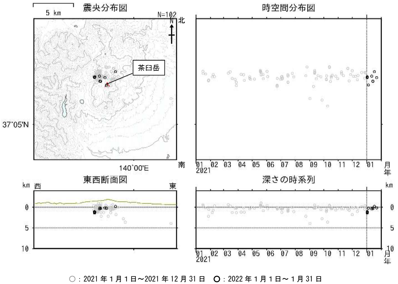
図5 那須岳 震源分布図（2021年1月1日~2022年1月31日）
