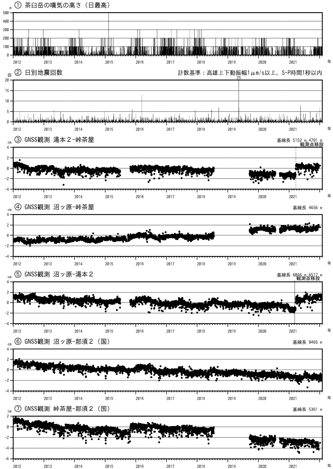
図4 那須岳 火山活動経過図（2012年1月1日～2022年1月31日）
