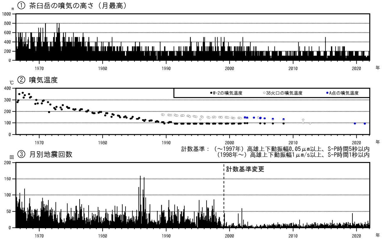
図3-1 那須岳 火山活動経過図（1966年5月～2022年1月）
