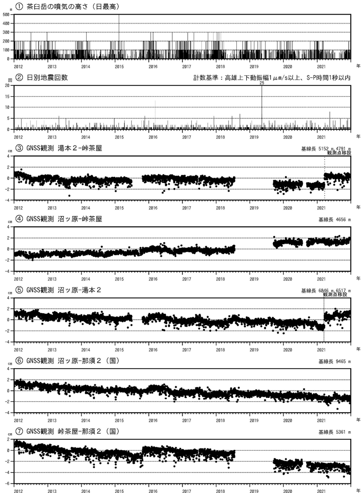
図4 那須岳 火山活動経過図（2012年1月1日～2021年12月31日）
