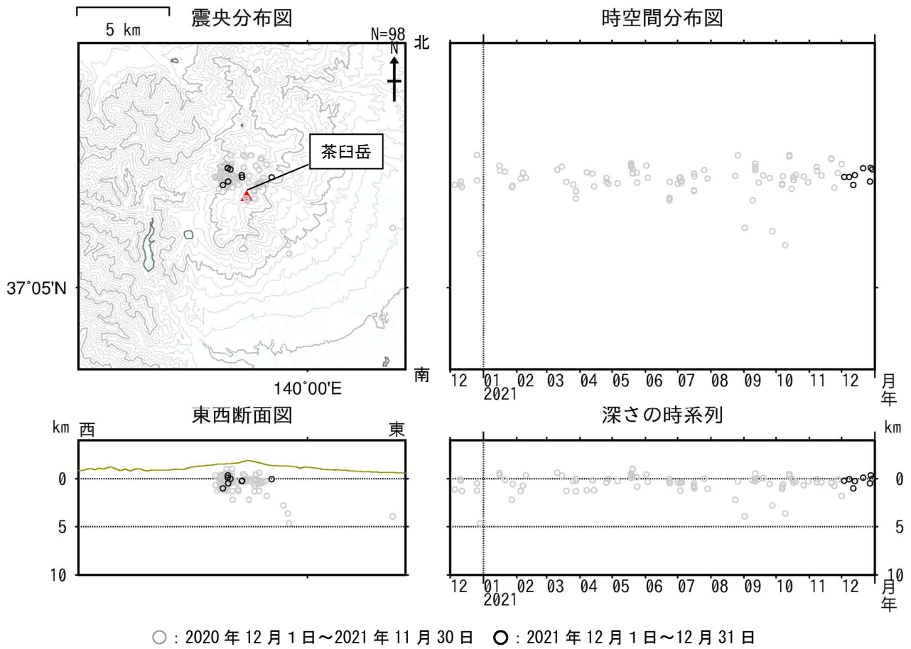
図5 那須岳 震源分布図（2020年12月1日～2021年12月31日）
