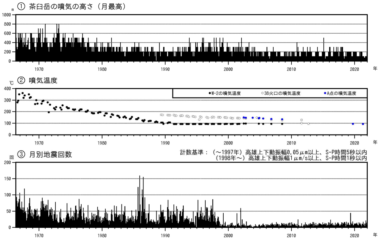
図3-1 那須岳 火山活動経過図（1966年5月～2021年12月）
