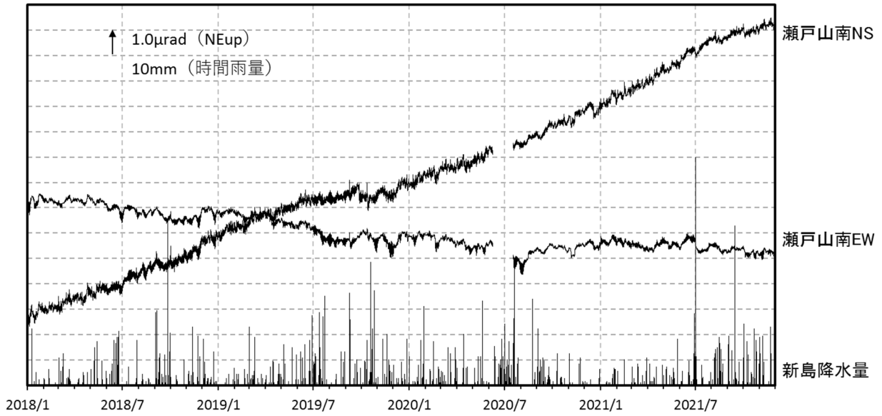
図4 新島 瀬戸山南観測点の傾斜変動（2018年1月1日～2021年11月30日）
