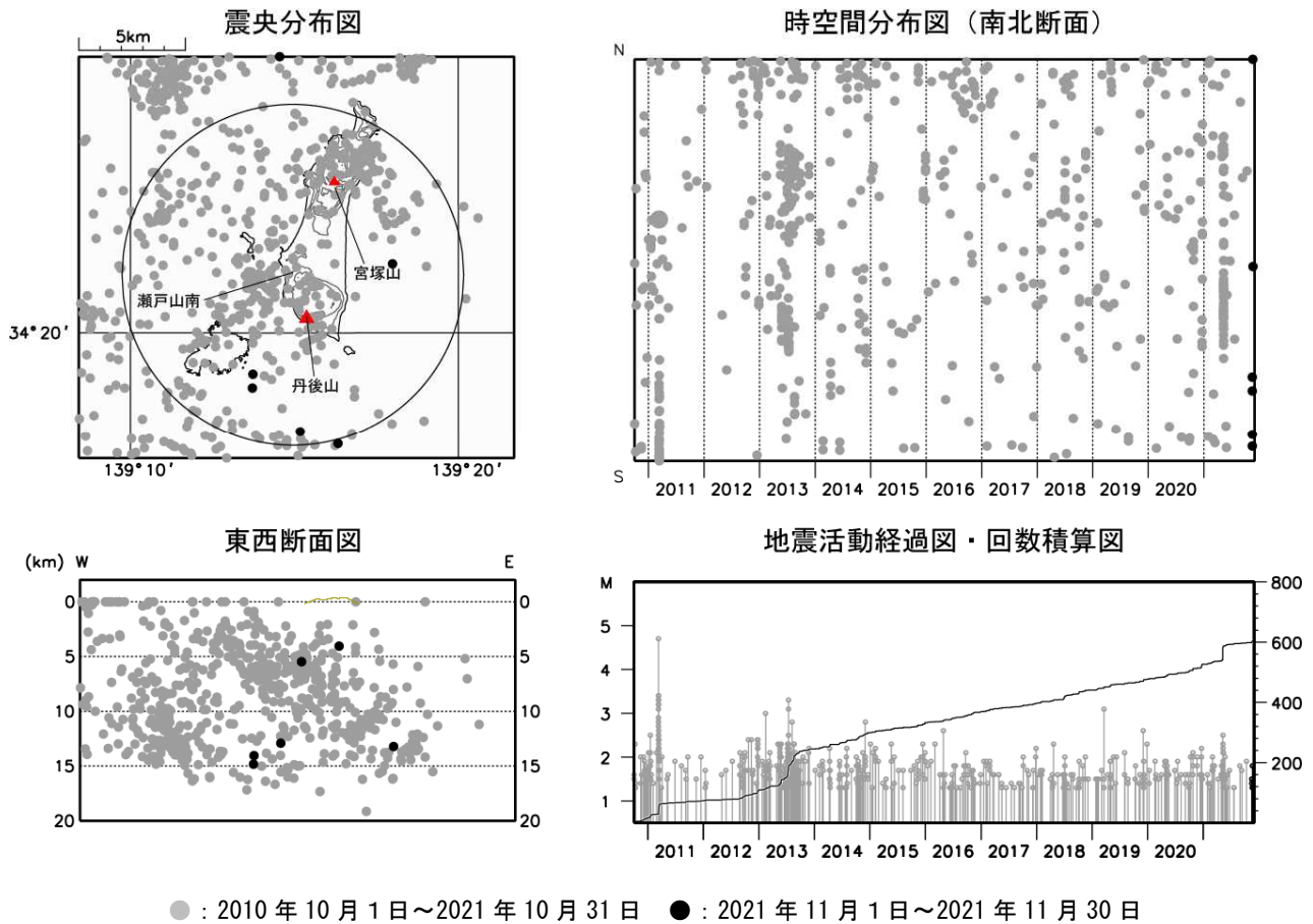
図3 新島 広域地震観測網による山体・周辺の地震活動（2010年10月1日～2021年11月30日） 広域地震観測網により震源決定したもので、深さは全て海面以下として決定しています。 M（マグニチュード）は地震の規模を表し、M1.3以上の地震を示しています。 図中の震源要素は一部暫定値が含まれており、後日変更することがあります。 計数対象（瀬戸山南から半径約8km、深さ約20km以内）以外の地震が含まれるため、図2-①の日別A型地震回数とは異なります。 震央分布図中の円は火山性地震の回数の計数対象（瀬戸山南から半径8km、深さ20km以内）の範囲を示しています。 この図では、関係機関の地震波形を一元的に処理し、地震観測点の標高を考慮する等した新手法で得られた震源を用いています（ただし、2020年8月以前の地震については火山活動評価のための参考震源です）。 2021年12月8日現在、次の期間の地震について、暫定的に震源精査の基準を変更しているため、その前後の期間と比較して微小な地震での震源決定数の変化（増減）が見られます。 (1)2020年9月1日から10月23日まで、(2)2021年1月9日から3月7日まで、(3)2021年4月19日以降
