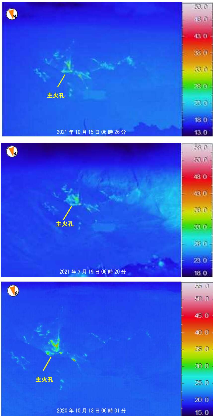
図5 三宅島 山頂火口内の地熱域の状況（スオウ穴からの撮影）
