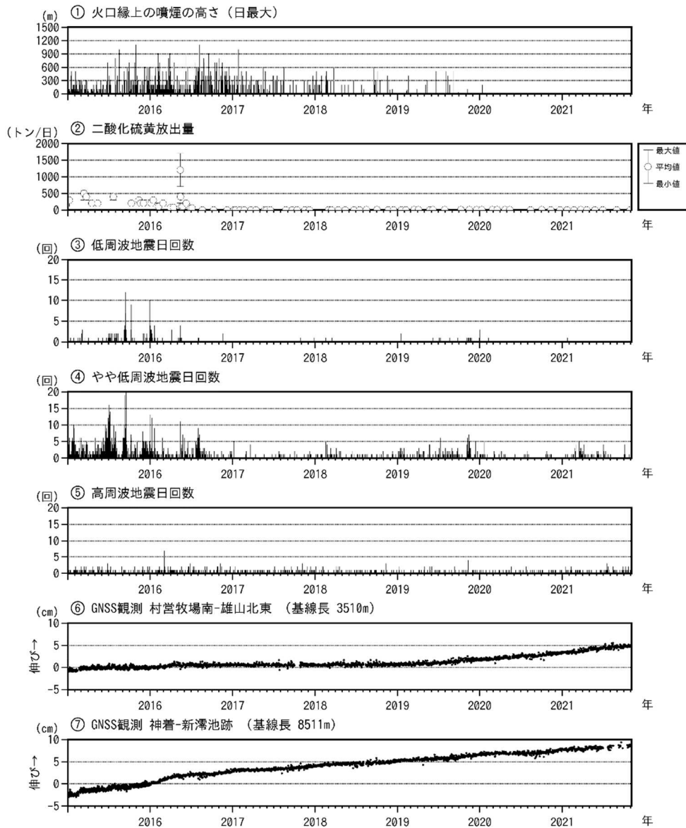
図7 三宅島 火山活動短期経過図（2015年1月1日～2021年10月31日）
