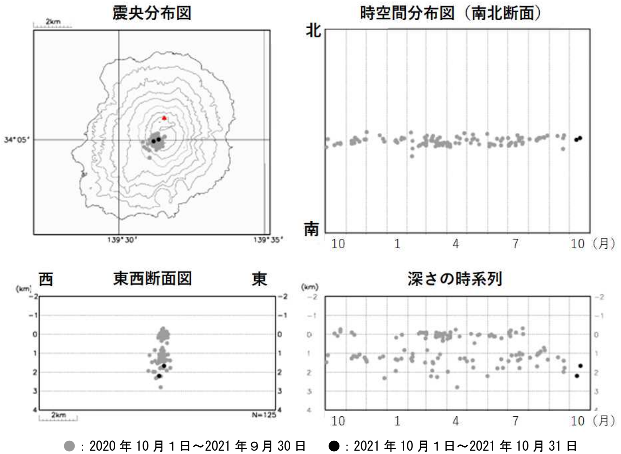
図9 三宅島 震源分布図（2020年10月1日～2021年10月31日）
