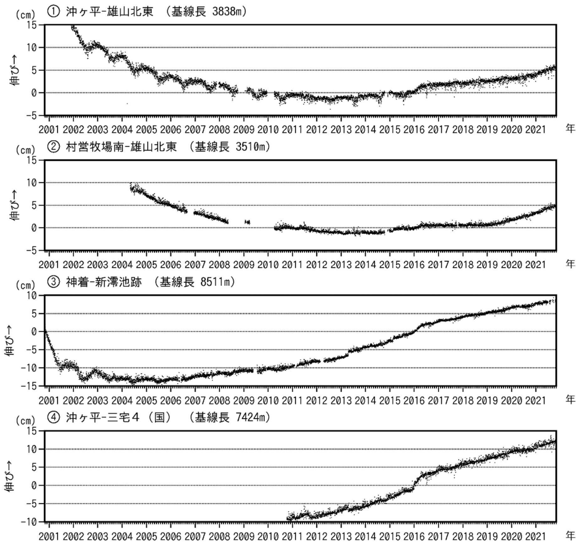
図8 三宅島 GNSS 連続観測結果（2000年10月26日～2021年10月31日）
