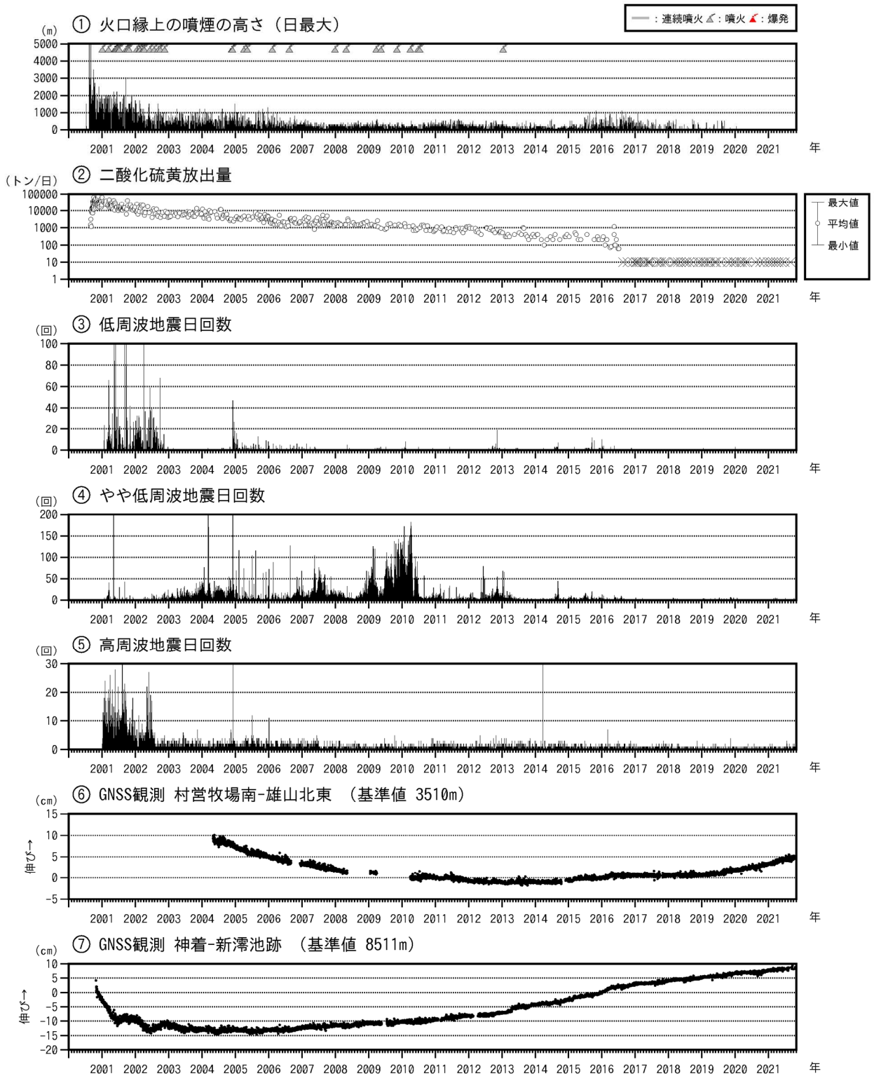
図6 三宅島 火山活動長期経過図（2000年1月1日～2021年10月31日） ※図6の説明は次ページに掲載。
