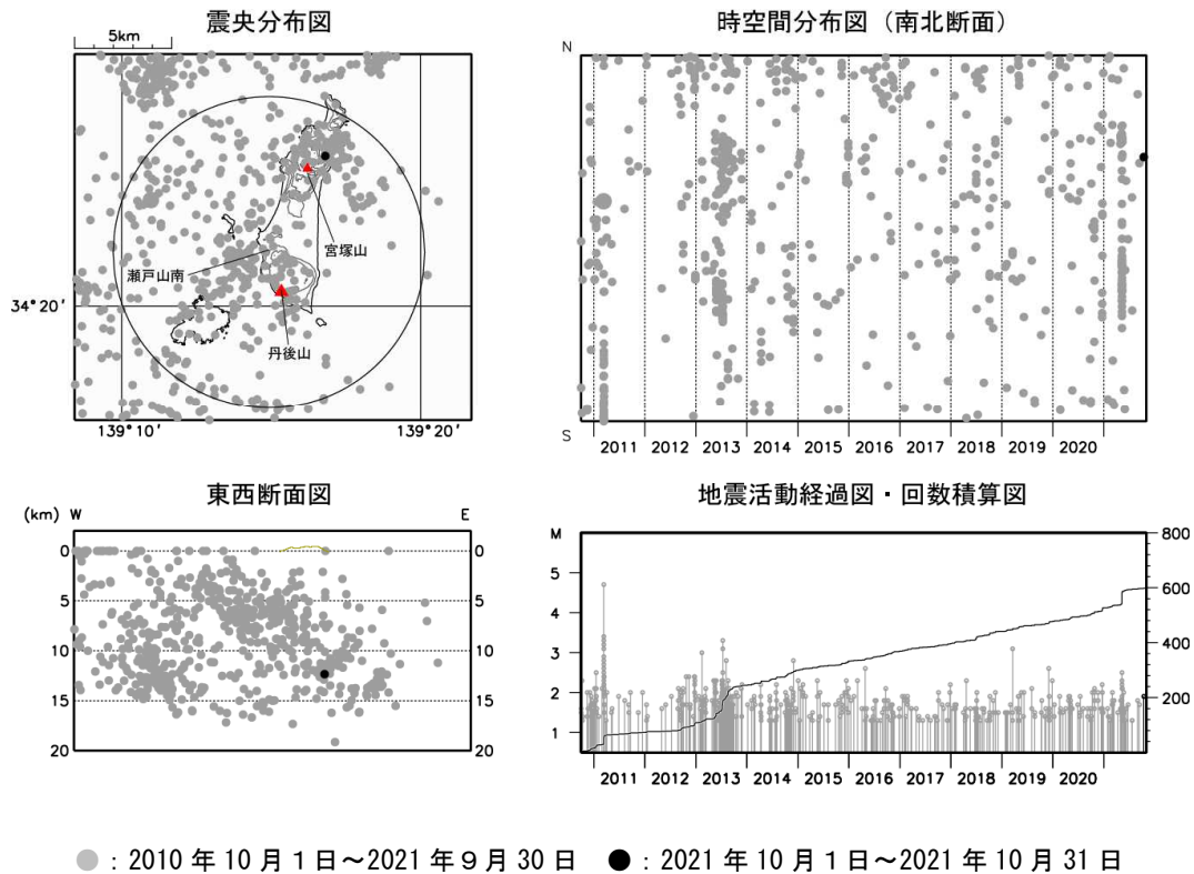
図3 新島 広域地震観測網による山体・周辺の地震活動（2010年10月1日～2021年10月31日） 広域地震観測網により震源決定したもので、深さは全て海面以下として決定しています。 M（マグニチュード）は地震の規模を表し、M1.3以上の地震を示しています。 図中の震源要素は一部暫定値が含まれており、後日変更することがあります。 計数対象（瀬戸山南から半径約8km、深さ約20km以内）以外の地震が含まれるため、図2-①の日別A型地震回数とは異なります。 震央分布図中の円は火山性地震の回数の計数対象（瀬戸山南から半径8km、深さ20km以内）の範囲を示しています。 この図では、関係機関の地震波形を一元的に処理し、地震観測点の標高を考慮する等した新手法で得られた震源を用いています（ただし、2020年8月以前の地震については火山活動評価のための参考震源です）。 2021年11月9日現在、次の期間の地震について、暫定的に震源精査の基準を変更しているため、その前後の期間と比較して微小な地震での震源決定数の変化（増減）が見られます。 (1)2020年9月1日から10月23日まで、(2)2021年1月9日から3月7日まで、(3)2021年4月19日以降
