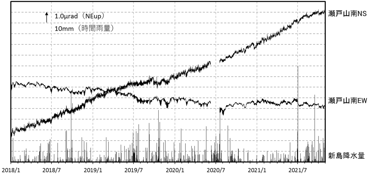
図4 新島 瀬戸山南観測点の傾斜変動（2018年1月1日～2021年10月31日）
