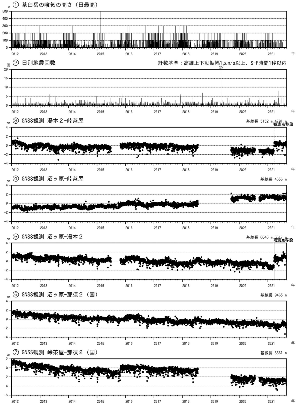
図4 那須岳 火山活動経過図 (2012年1月1日~2021年8月31日)
