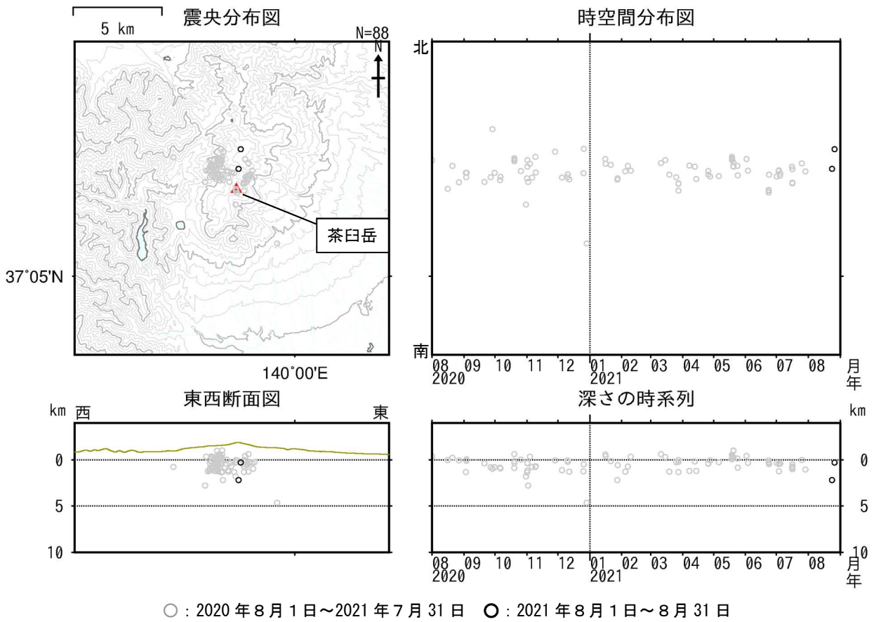
図5 那須岳 震源分布図（2020年8月1日～2021年8月31日）
