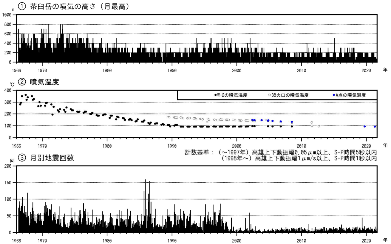
図3-1 那須岳 火山活動経過図（1966年1月～2021年8月）
