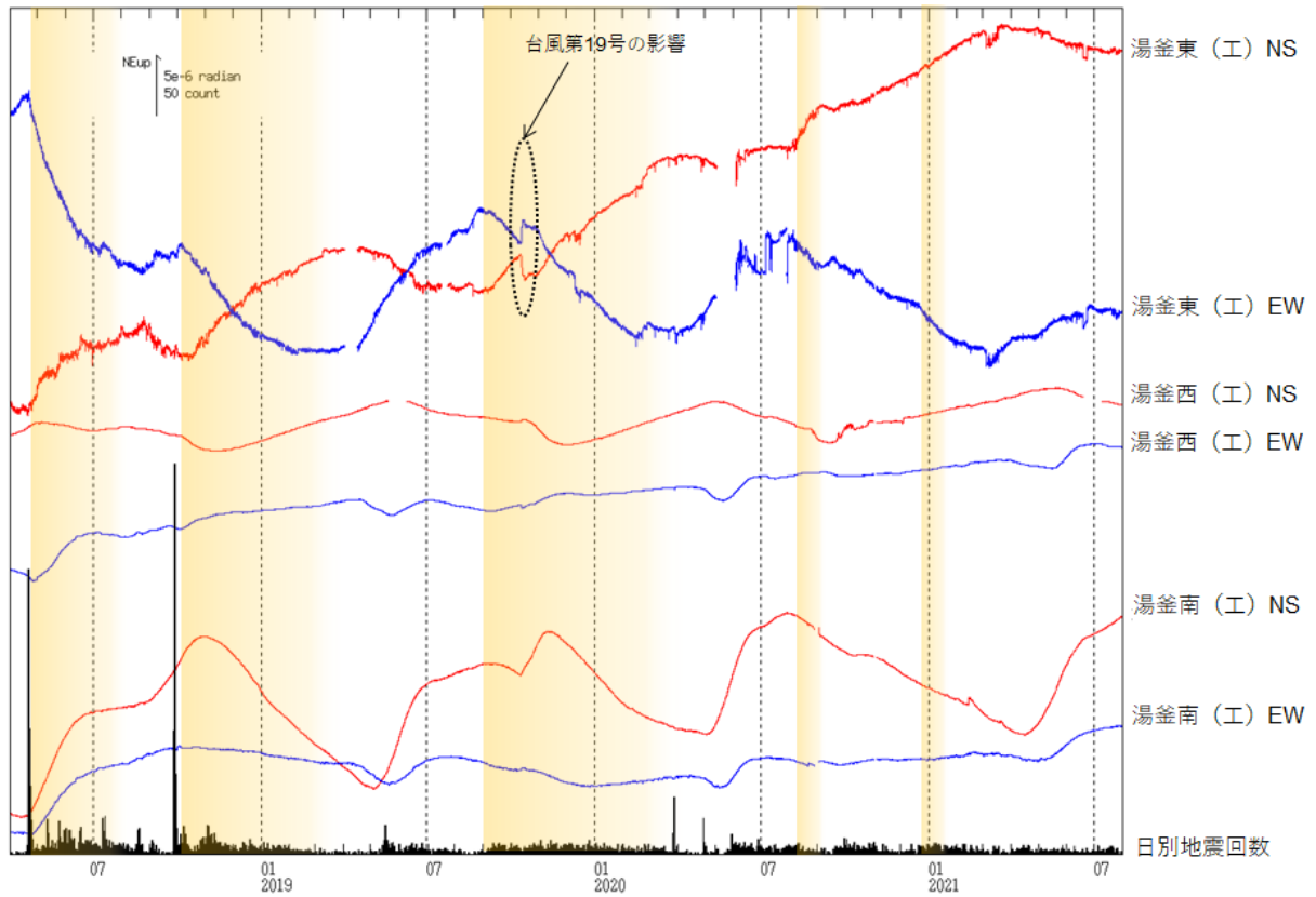
図6 草津白根山（白根山（湯釜付近）） 傾斜変動（2018年4月1日～2021年7月31日） （工）：東京工業大学
