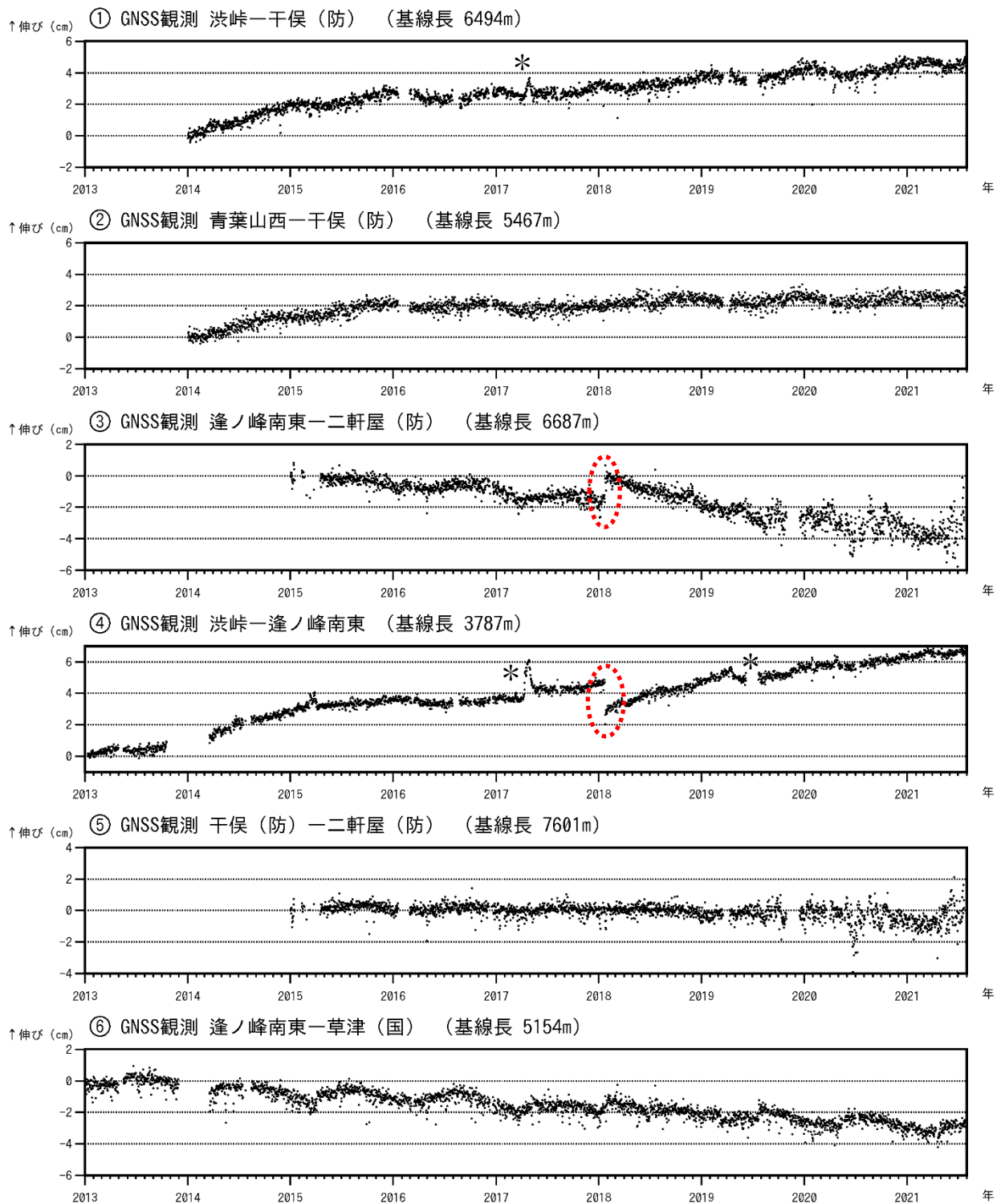
図7 草津白根山 GNSS連続観測の結果 (2013年1月1日~2021年7月31日)
