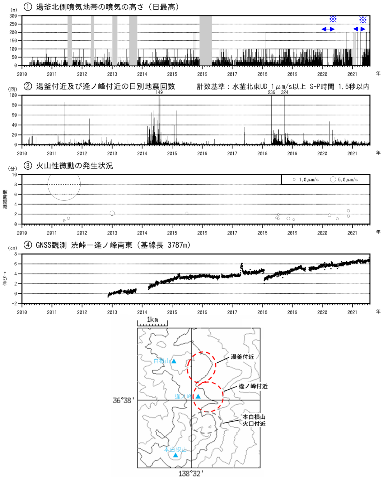
図4 草津白根山（白根山（湯釜付近））火山活動経過図（2010年1月1日～2021年7月31日） ①の灰色部分及び④の空白部分は欠測を示します。また、※の青矢印期間は（2020年1月から4月にかけて、及び2021年1月から4月にかけて）は、一部の観測機器で障害が発生しているため、100m未満の噴気については観測できていない期間があります。 ④は図8の④の基線に対応しています。2013年1月に解析方法を変更しています。 最下段の図は、図2①②③と図4②の地震の震源の概ねの位置を示しています。 ・草津白根山では、2014年や2018年に湯釜付近浅部への火山性流体の著しい供給の増加によると考えられる火山性地震の活発化と浅部の膨張などが観測されました。草津白根山の火山活動は、短期的には活動の消長があるものの、中長期的には活発な状態が継続していると考えられます。 ・GNSS連続観測では、2018年1月の本白根山噴火に伴う変化が認められた後、2020年1月にかけて、噴火後の本白根山の収縮によるものと考えられる変動が見られました。 ・GNSS連続観測では、今期間、火山活動によるとみられる変動は認められません。
