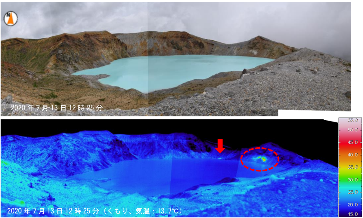
図1-2 草津白根山（白根山（湯釜付近）） 湯釜火口内の状況
