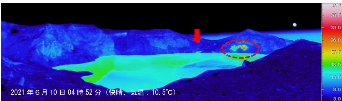
図1-1 草津白根山（白根山（湯釜付近）） 湯釜火口内の状況
