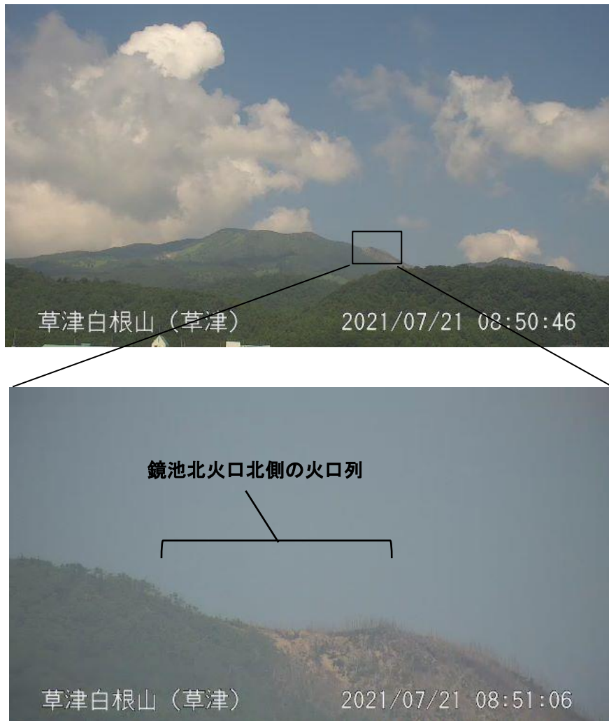
図12 草津白根山（本白根山） 本白根山付近の状況（7月21日草津監視カメラ）
