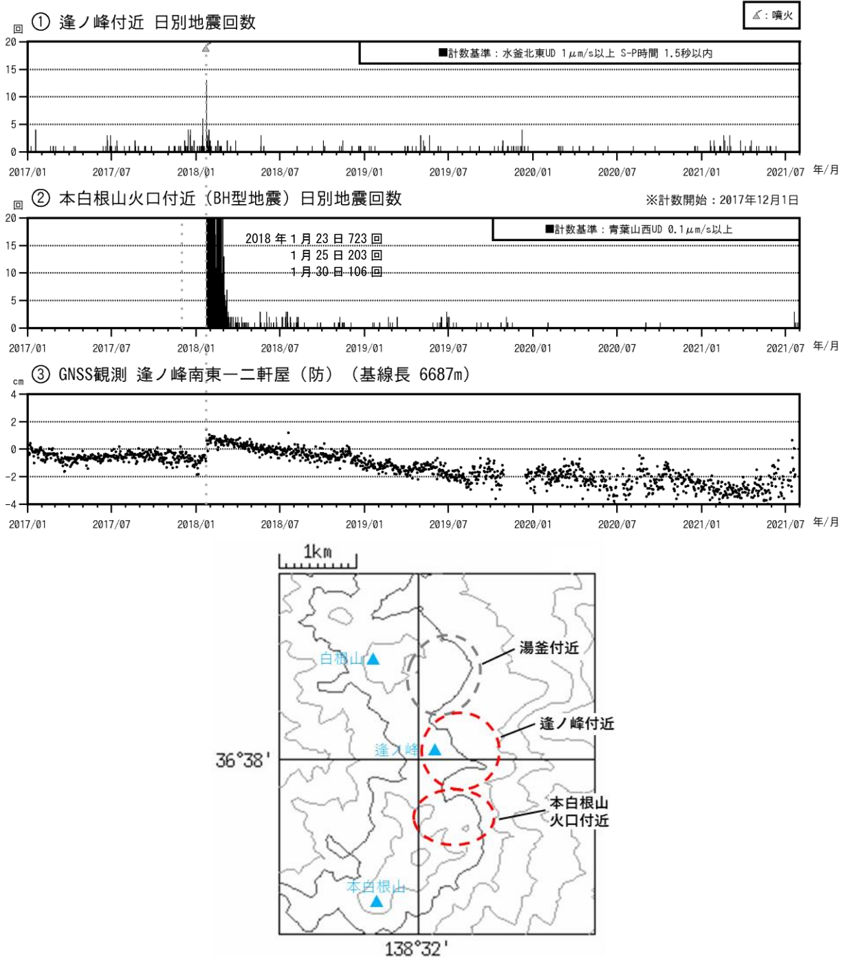
図13 草津白根山（本白根山） 火山活動経過図（2017年1月1日～2021年7月31日）
