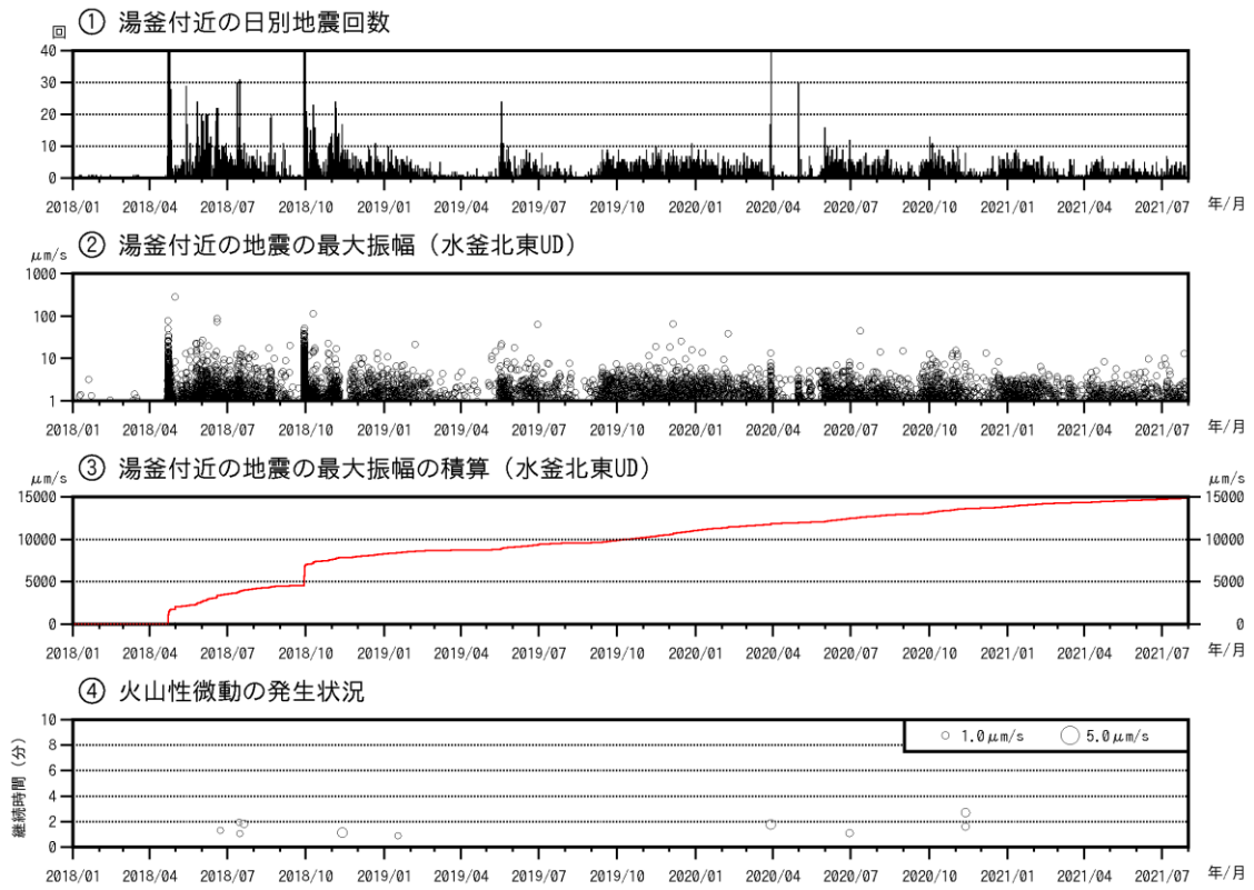
図2 草津白根山（白根山（湯釜付近）） 湯釜付近の地震活動及び火山性微動の発生状況 （2018年1月1日～2021年7月31日）
