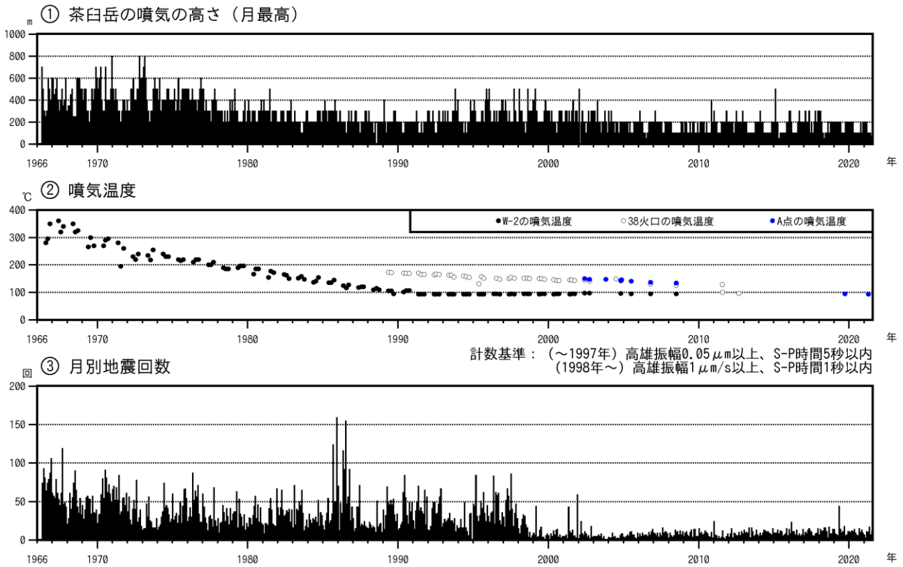
図3 那須岳 火山活動経過図（1966年1月～2021年7月）
