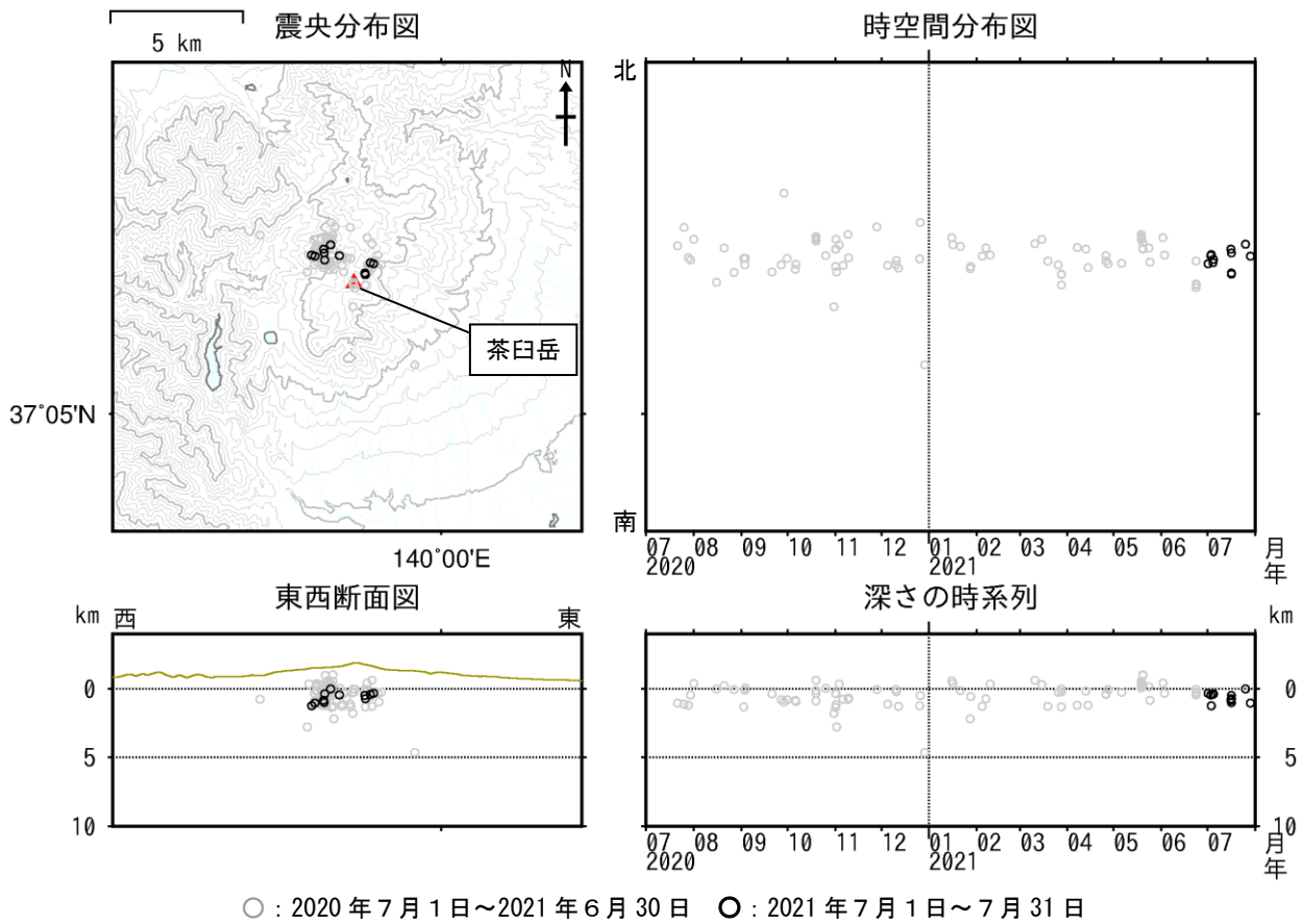
図5 那須岳 震源分布図（2020年7月1日～2021年7月31日）
