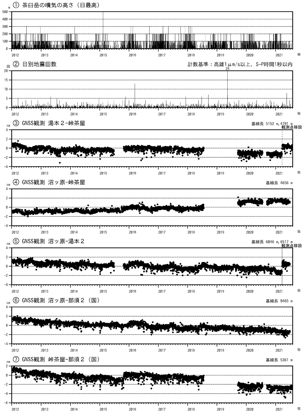
図4 那須岳 火山活動経過図（2012年1月1日～2021年7月31日）
