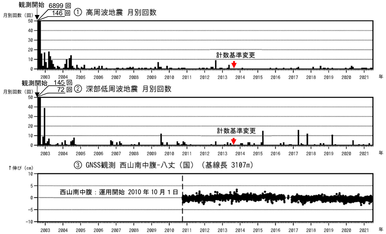
図2 八丈島 火山活動経過図 (2002年8月13日～2021年6月30日)
