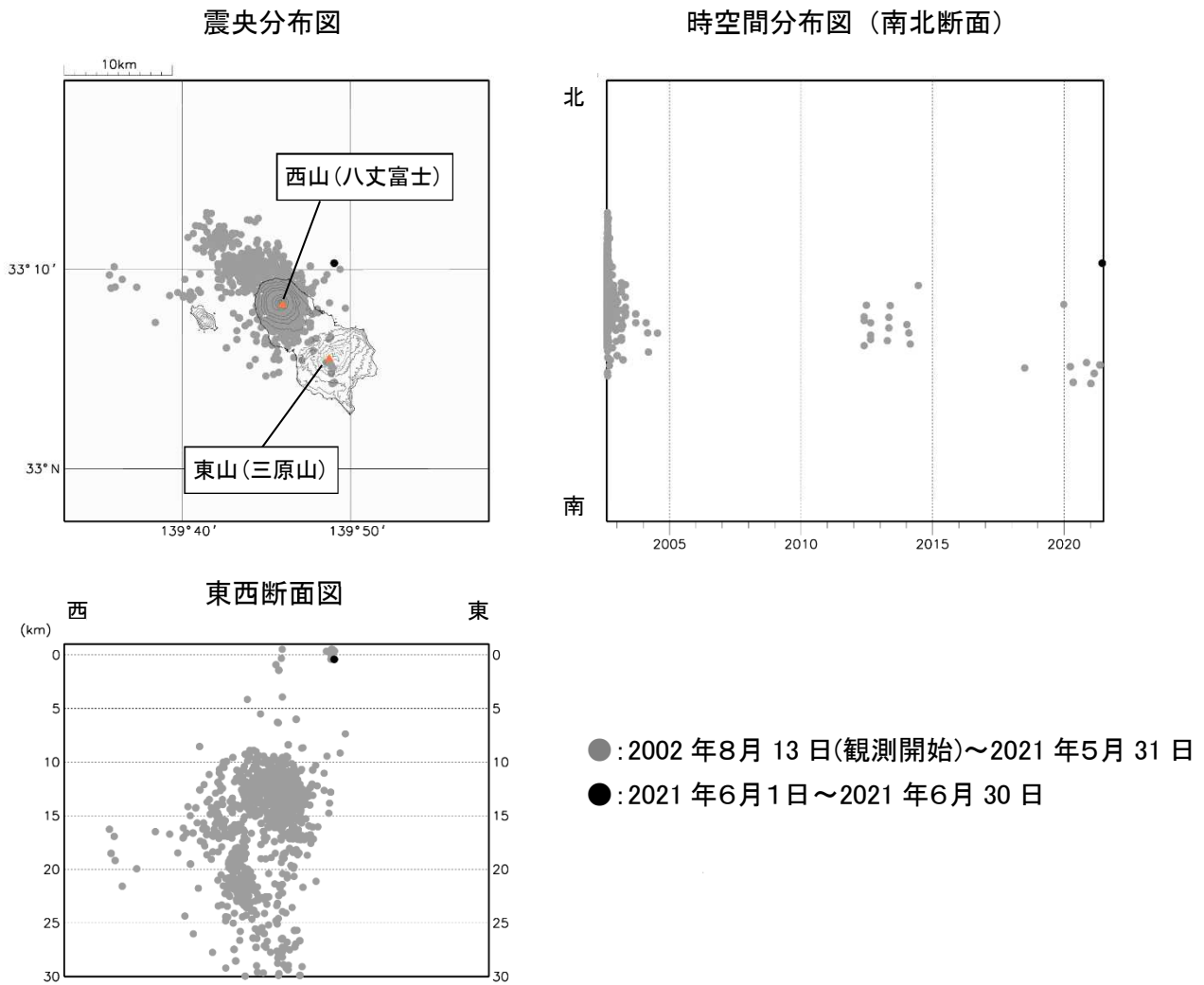
図3 八丈島 震源分布図（2002年8月13日～2021年6月30日）
