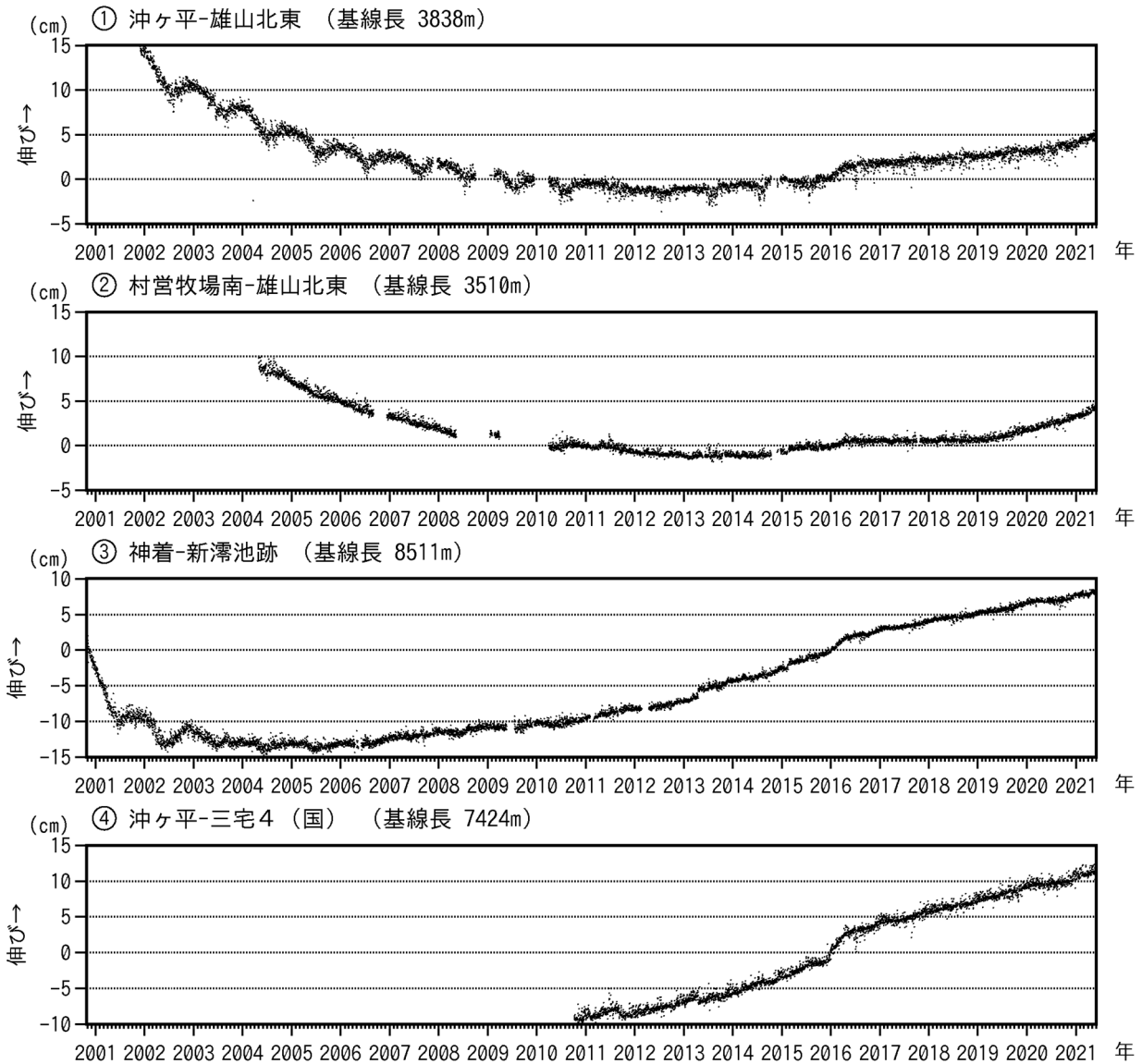
図7 三宅島 GNSS 連続観測結果（2000年10月26日～2021年5月31日）
