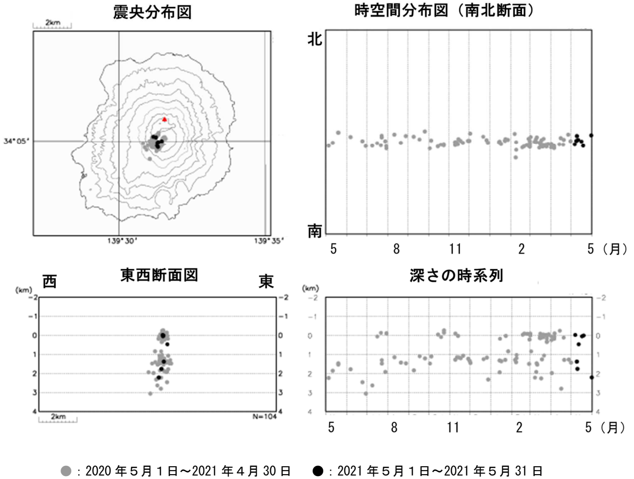
図8 三宅島 震源分布図（2020年5月1日～2021年5月31日）
