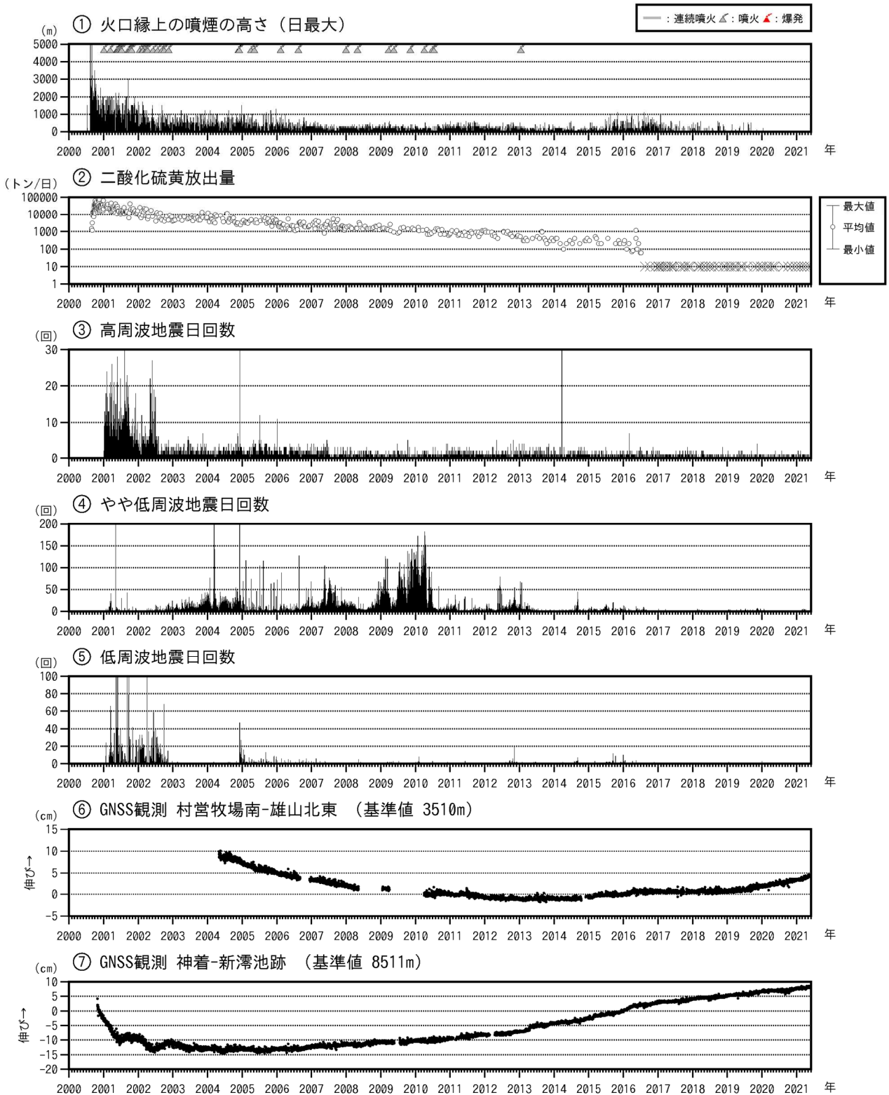
図5 三宅島 火山活動長期経過図（2000年1月1日～2021年5月31日）
