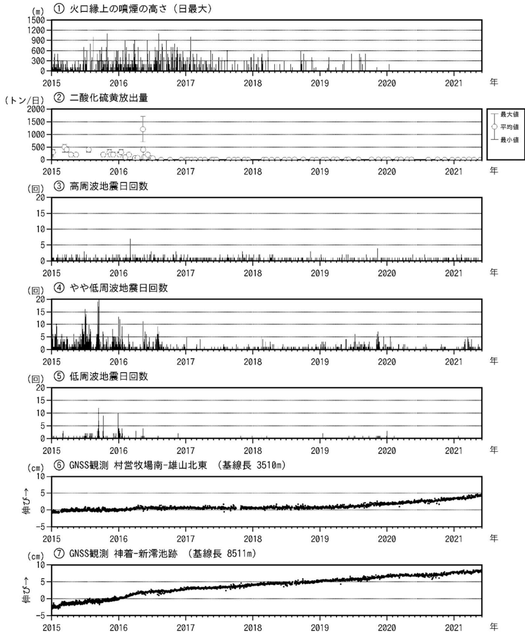
図6 三宅島 火山活動短期経過図（2015年1月1日～2021年5月31日）
