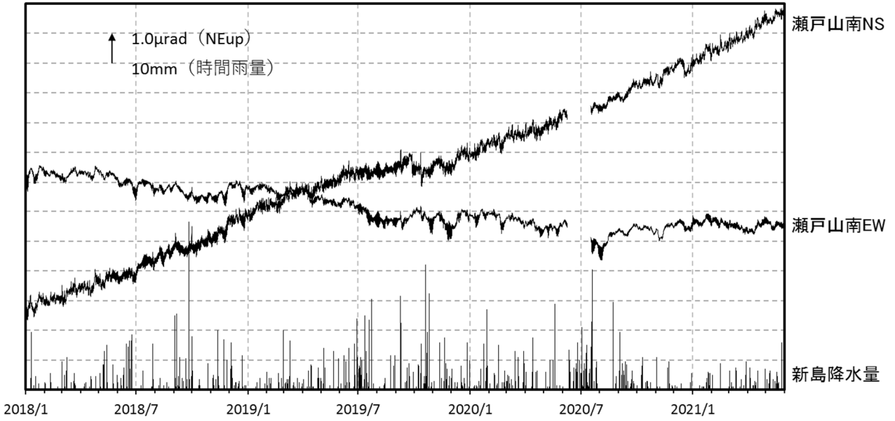
図4 新島 瀬戸山南観測点の傾斜変動（2018年1月1日～2021年5月31日）
