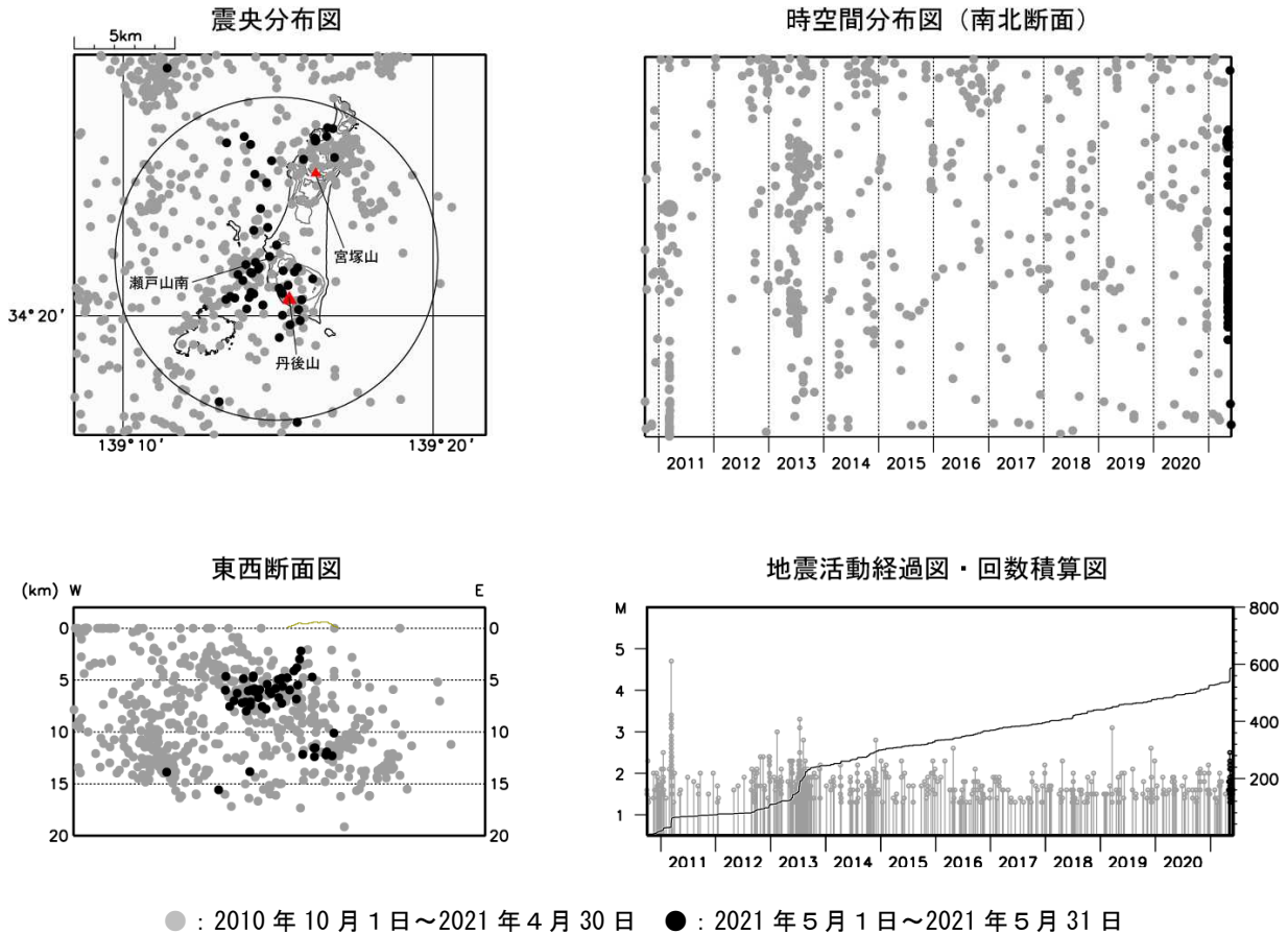
図3 新島 広域地震観測網による山体・周辺の地震活動（2010年10月1日～2021年5月31日） 広域地震観測網により震源決定したもので、深さは全て海面以下として決定しています。 M（マグニチュード）は地震の規模を表し、M1.3以上の地震を示しています。 図中の震源要素は一部暫定値が含まれており、後日変更することがあります。 計数対象（瀬戸山南から半径約8km、深さ約20km以内）以外の地震が含まれるため、図2-①の日別A型地震回数とは異なります。 震央分布図中の円は火山性地震の回数の計数対象（瀬戸山南から半径8km、深さ20km以内）の範囲を示しています。 この図では、関係機関の地震波形を一元的に処理し、地震観測点の標高を考慮する等した新手法で得られた震源を用いています（ただし、2020年8月以前の地震については火山活動評価のための参考震源です）。 2021年6月8日現在、次の期間の地震について、暫定的に震源精査の基準を変更しているため、その前後の期間と比較して微小な地震での震源決定数の変化（増減）が見られます。 (1)2020年4月18日から10月23日まで、(2)2021年1月9日から3月7日まで、(3)2021年4月19日以降 ・10日に新島の北側及び南西側を震源とする地震がまとまって発生しました。最大の地震は10日00時17分に発生したマグニチュード2.5の地震で、新島村で震度2を観測しました。 ・新島では、2013年7月から8月にかけても地震のまとまった発生がみられています。
